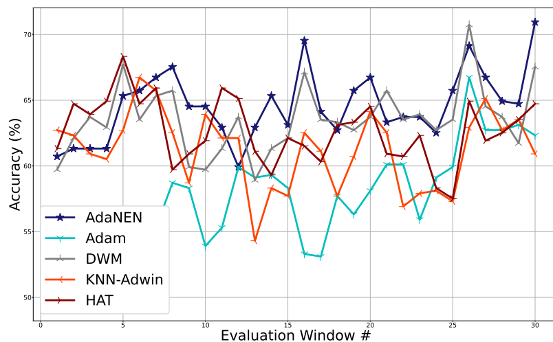
Figure 6.4: NYT.
