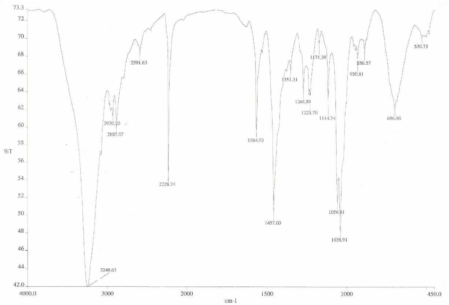
Şekil 5.9 4,5-Bis(2-hidroksietilmerkapt)-1,2-disiyanobenzen'in (5) IR spektrumu (KBr)
