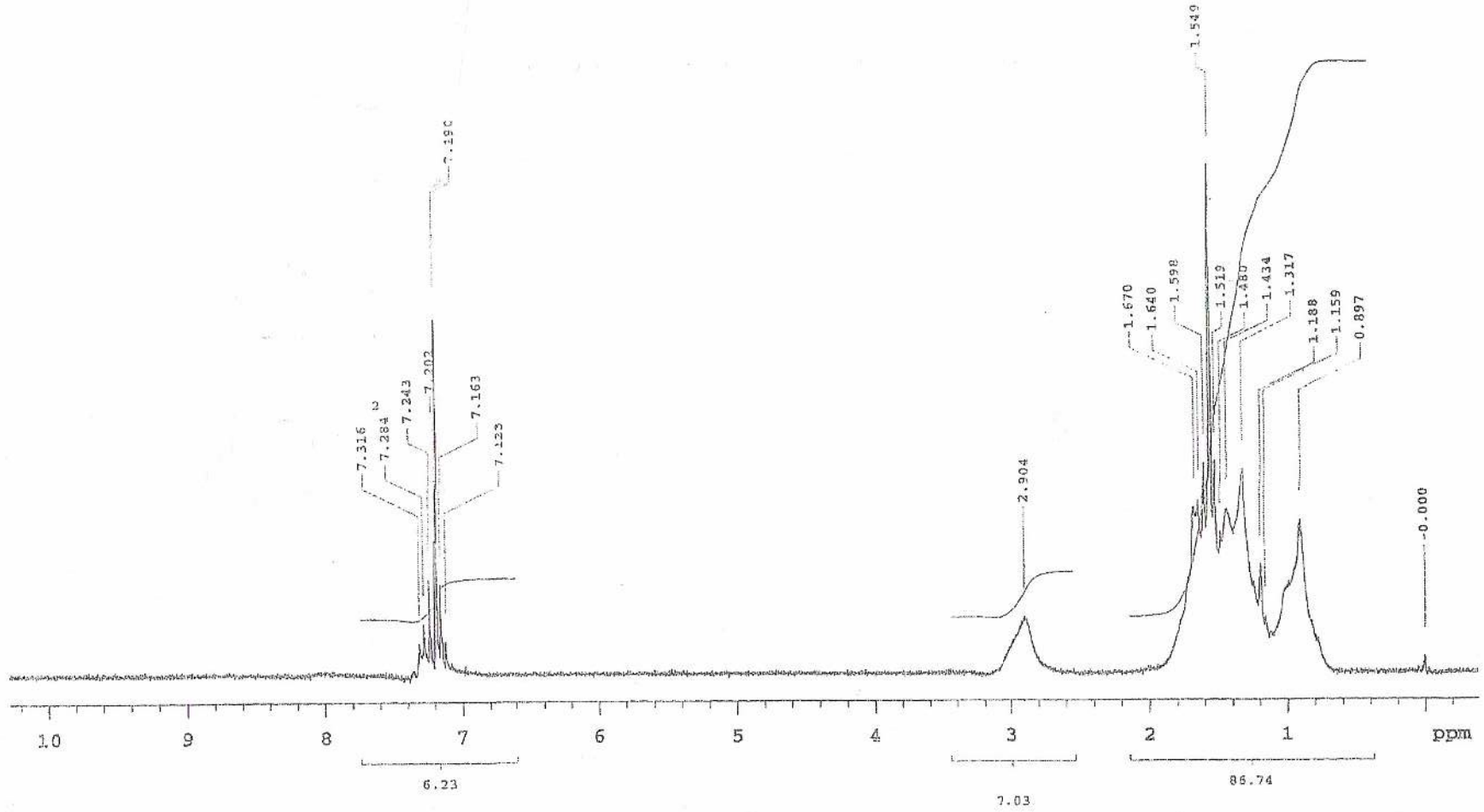
Şekil 5.13 1,2-Bis(2-hidroksietilmerkapto)-9,10,16,17,23,24-hekza(hekziltiyo)-ftalosiyanimatoçinko(II)'nin (7) 1 H-NMR spektrumu (CDCl 3 )
