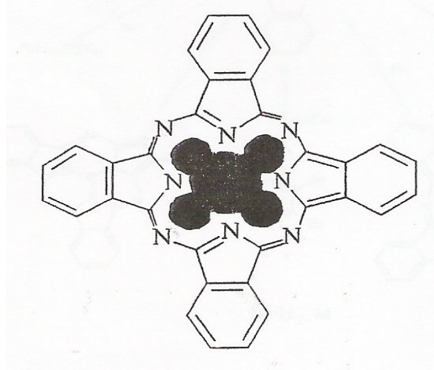
Şekil 2.5 Ftalosiyaninlerin en düşük enerjideki rezonans yapısı
