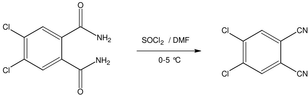
Şekil 4.4 4,5-Dikloro-1,2-disiyanobenzen sentezi (4)
