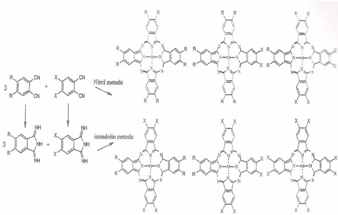
Şekil 2.22 İstatiksel ftalonitrillerin siklotetramerleşmesiyle asimetrik olarak süstitüe ftalosiyeninlerin sentezi
