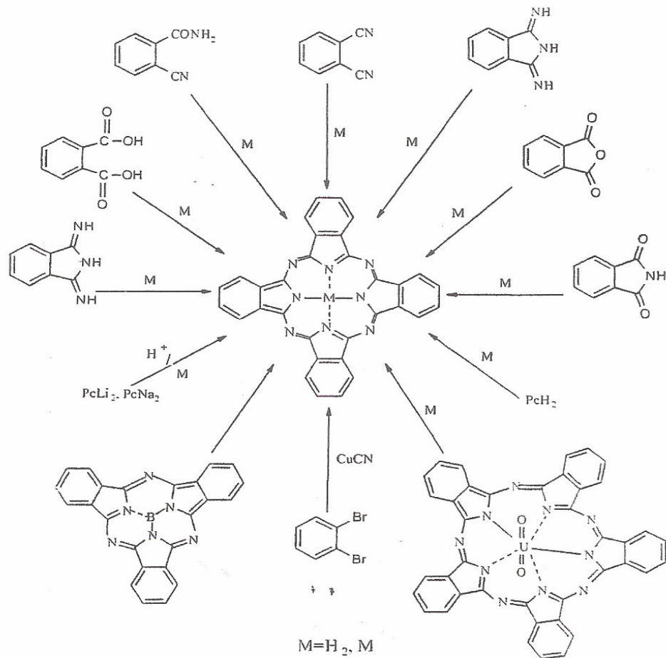
Şekil 2.6 Ftalosiyanın sentez yöntemleri
