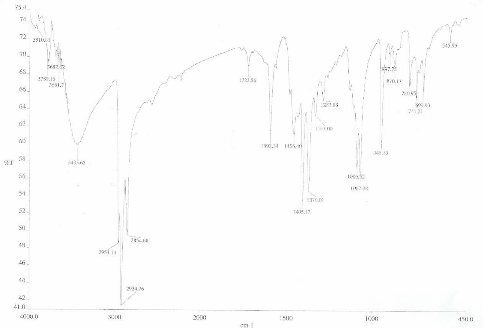
Şekil 5.14 1,2-Bis(2-hidroksietilmerkapt)-9,10,16,17,23,24-hekza(hekziltiyo)-ftalosiyaniatonikel(II)'nin (8) IR spektrumu (KBr)
