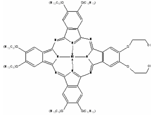
Şekil 5.2 1,2-Bis(2-hidroksietilmerkpto)-9,10,16,17,23,24-hekza(hekziltiyo)-ftalosiyaninatonikel(II)
