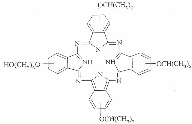
Şekil 2.23 Polimer üzerinden sentezlenen asimetrik ftalosiyenin örneği
