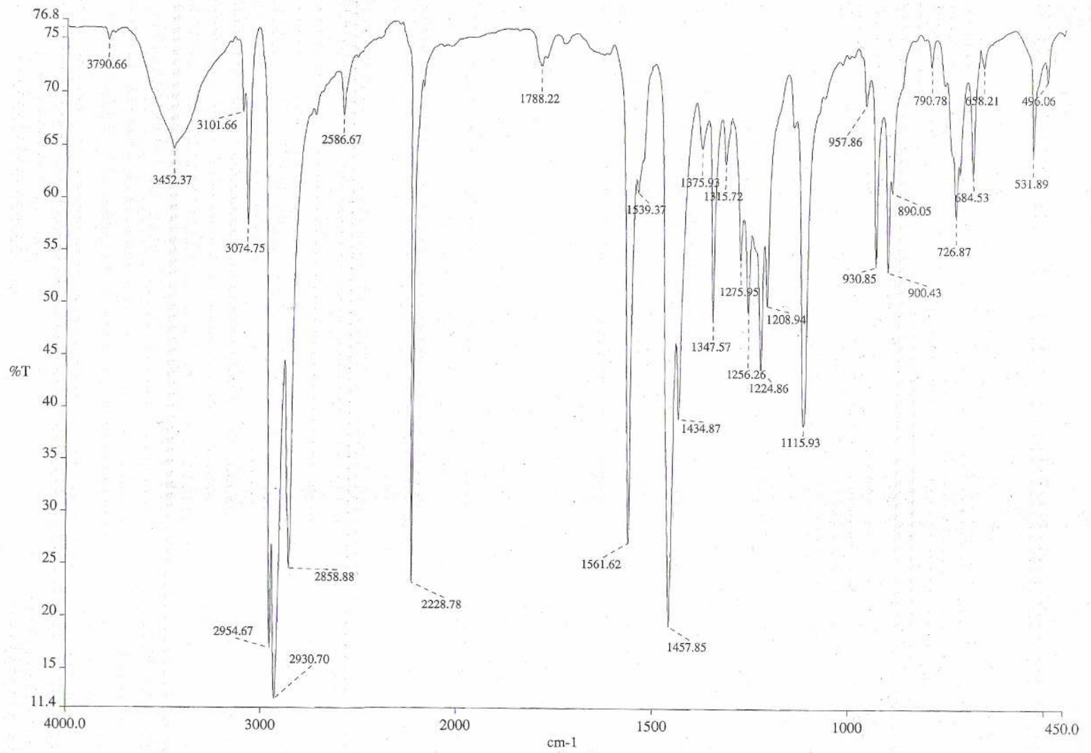
Şekil 5.10 4,5-Bis(hexiltiyo)-1,2-disiyanobenzen'in (6) IR spektrumu (KBr)
