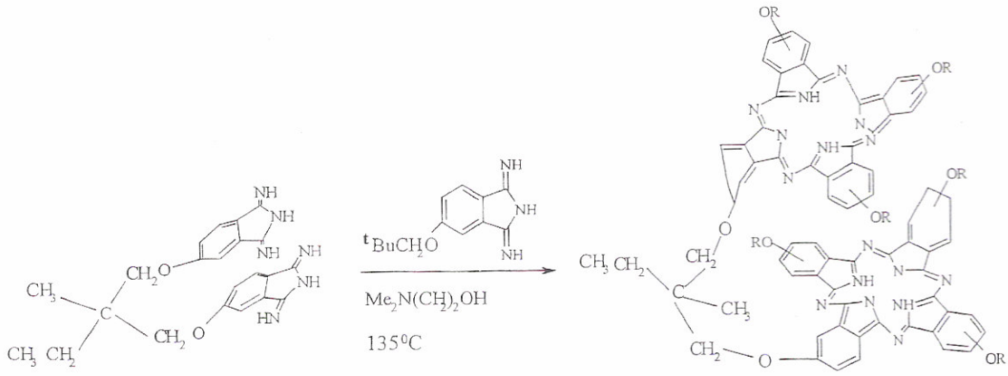
Şekil 2.20 Binükleer ve multinükleer ftalosiyanınlar
