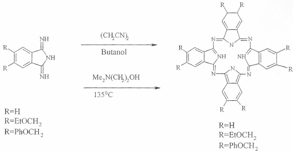
Şekil 2.19 Oktasübstitüe ftalosiyeninlerin sentezi
