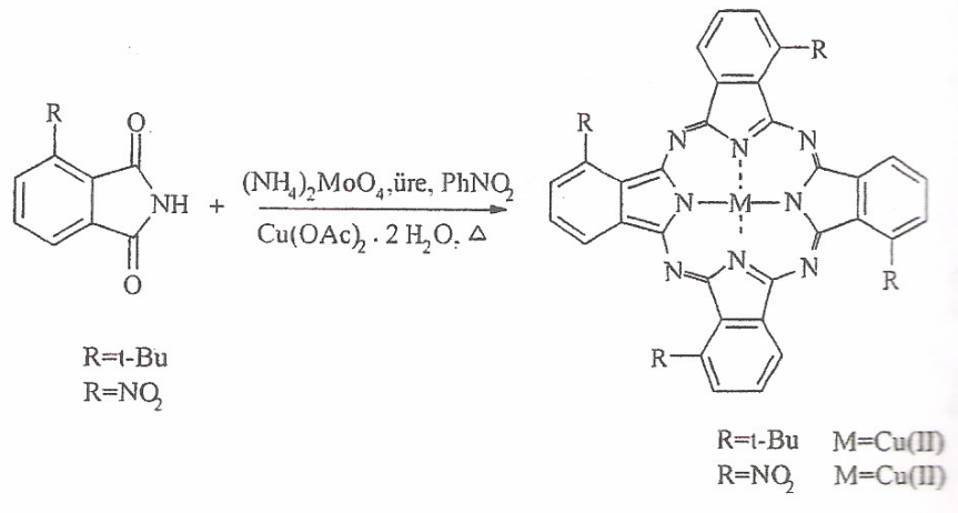
Şekil 2.12 Ftalimidden ftalosiyinin sentezi
