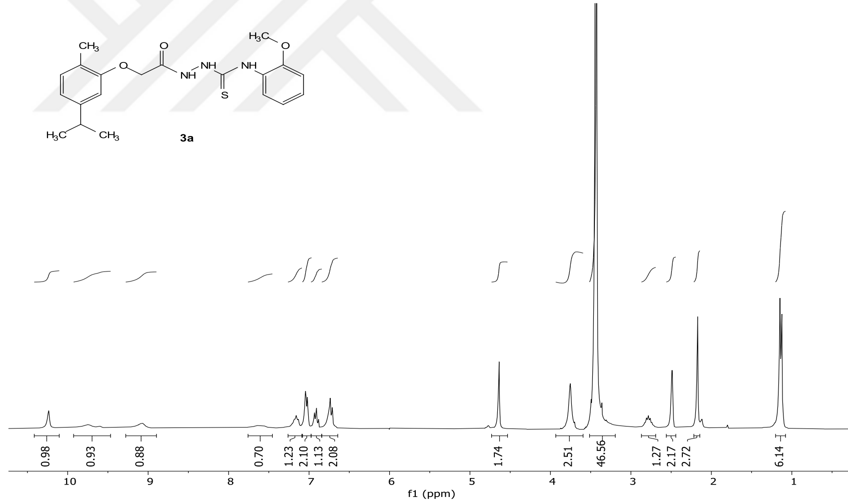
EK-5. (3a) bileşiğinin ^1\text{H} NMR spektrumu (300 MHz, DMSO- d_6 )
