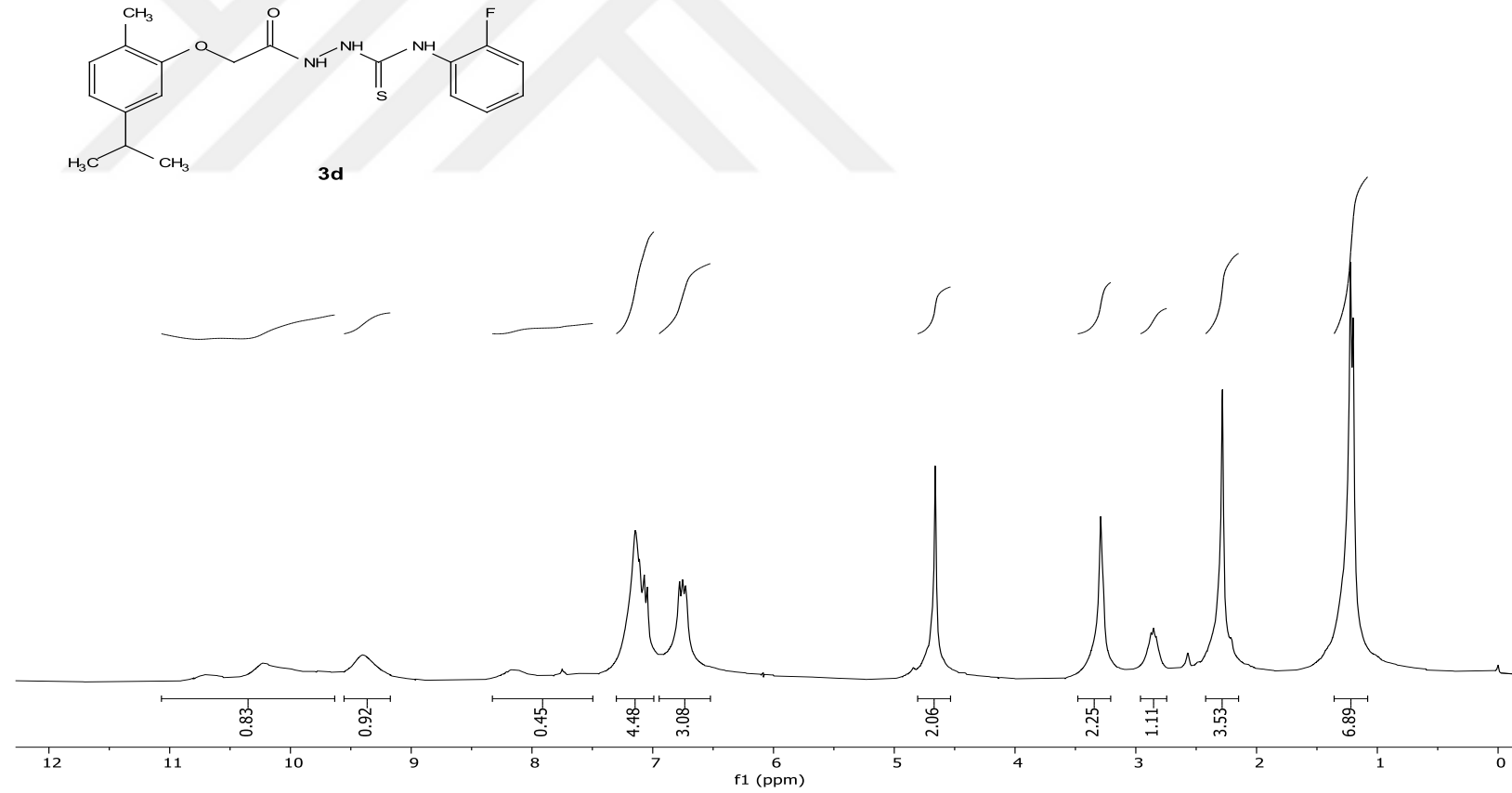
EK-11. (3d) bileşiğinin ^1\text{H} NMR spektrumu (300 MHz, DMSO- d_6 )
