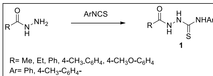
Şekil 2.32. 1,4-disüstitüe tiyosemikarbazitlerin sentezi
