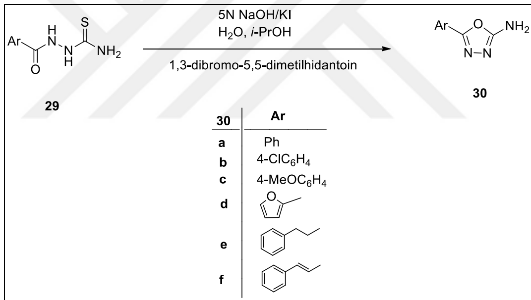
Şekil 2.45. 2-Amino-5-aril-1,3,4-oksadiazollerin sentezi
