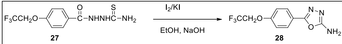
Şekil 2.44. 2-Amino-5-[4-(2',2',2'-trifluoroetoksi)-fenil]-1,3,4-oksadiazol sentezi
