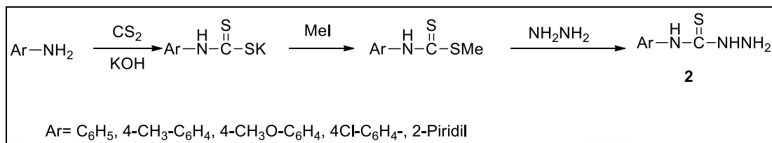
Şekil 2.33. 4-Ariltiyosemikarbazitlerin sentezi
