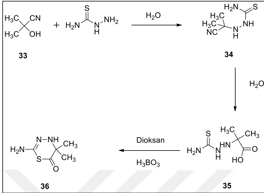
Şekil 2.47. 2-Amino-5,5-dimetil-1,3,4-tiadiazin sentezi
