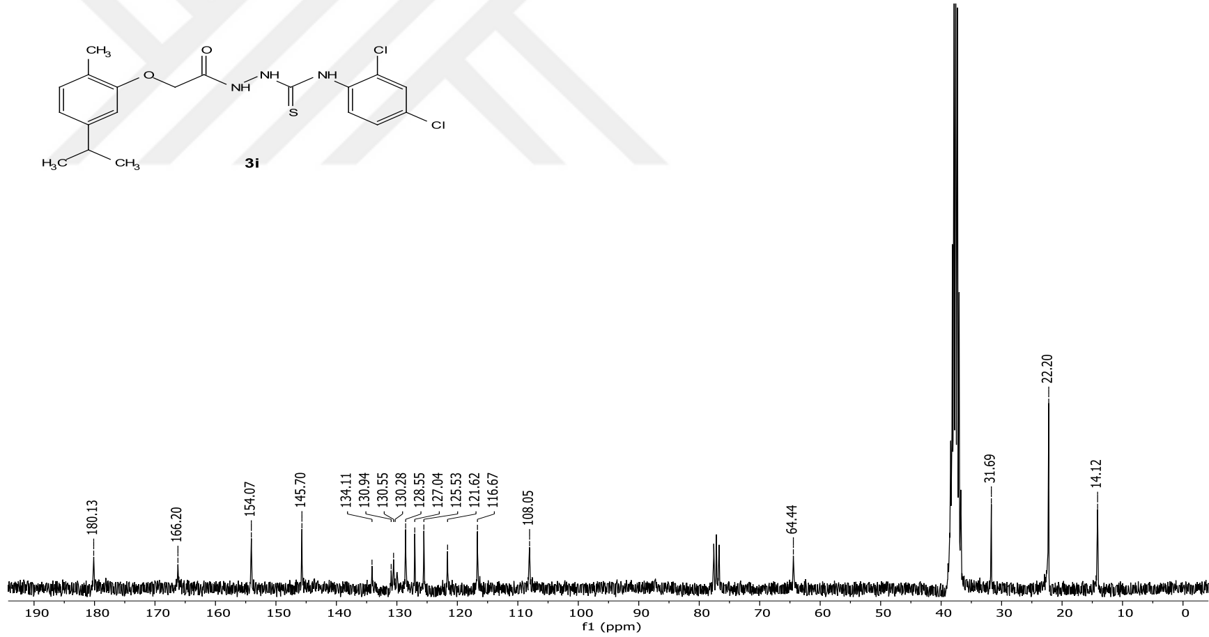
EK-22. (3i) bileşiğinin ^{13}\text{C} NMR spektrumu (75 MHz, \text{CDCl}_3 + \text{DMSO-d}_6 )
