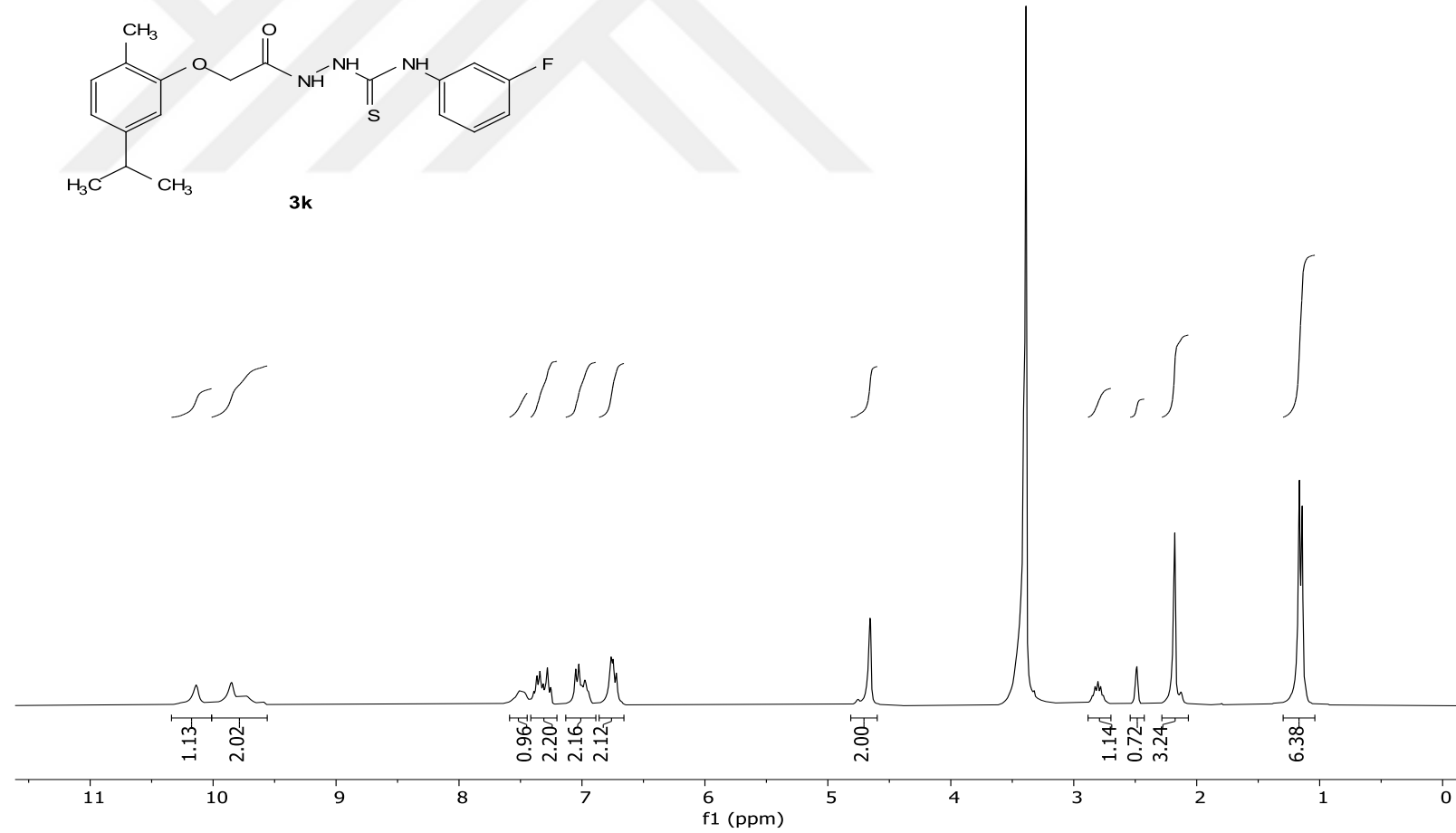
EK-25. (3k) bileşığının ^1\text{H} NMR spektrumu (300 MHz, DMSO- d_6 )
