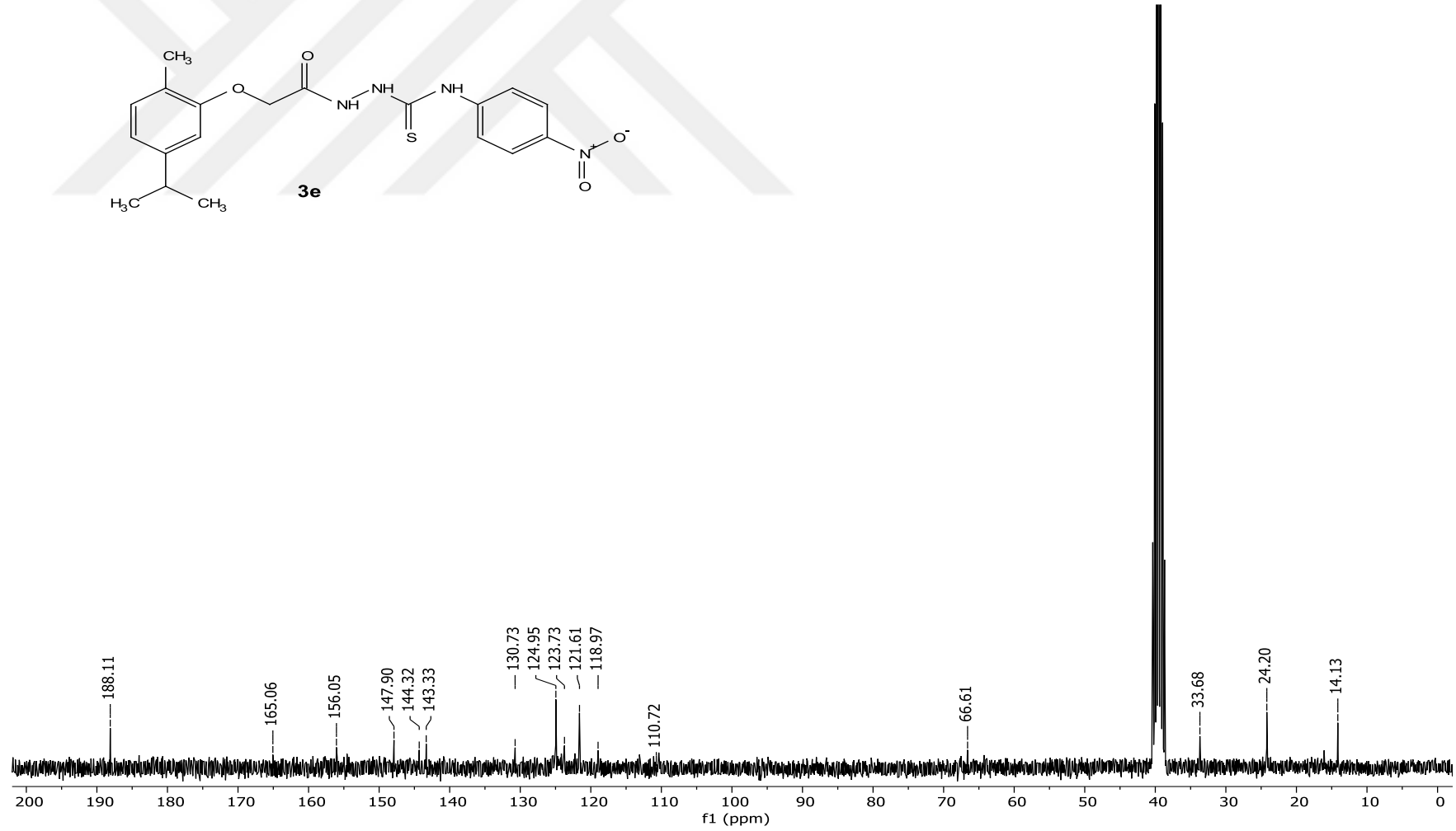
EK-14. (3e) bileşiğinin ^{13}\text{C} NMR spektrumu (75 MHz, DMSO-d 6 )
