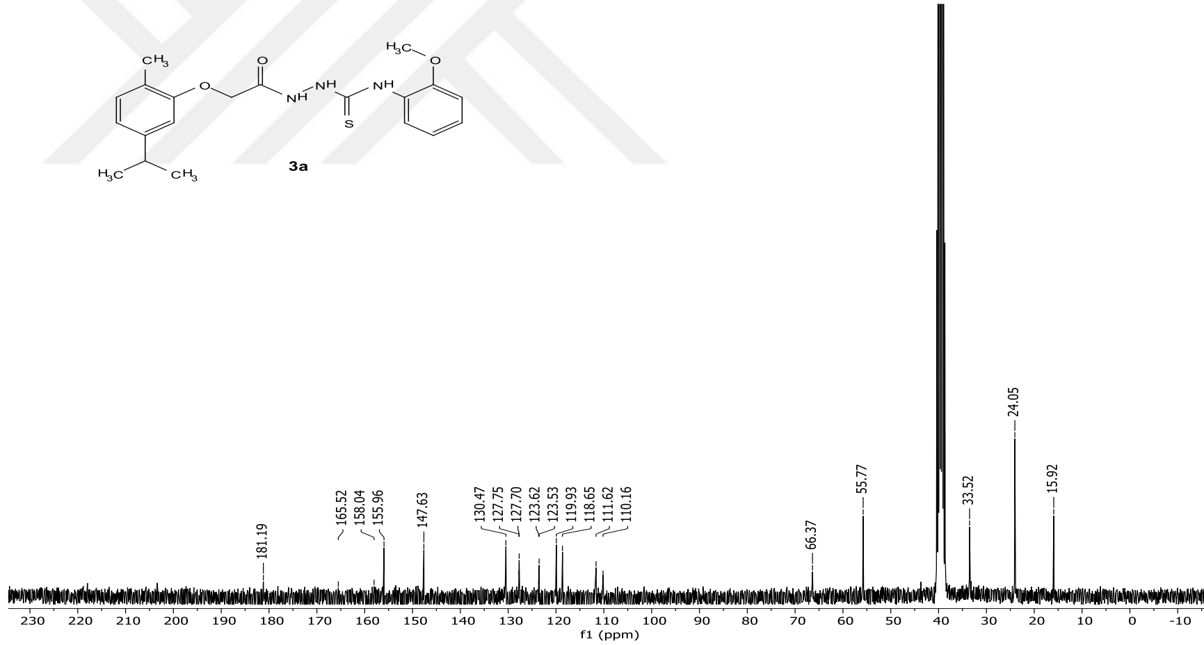
EK-6. (3a) bileşiminin ^{13}\text{C} NMR spektrumu (75 MHz, DMSO-d 6 )
