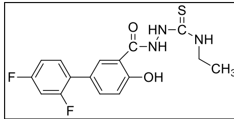
Şekil 2.16. Antibakteriyel etkili etil izosiyosiyonat türevi tiyosemikarbazit
