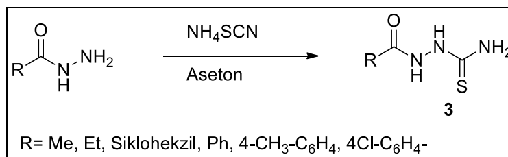
Şekil 2.34. 1-Aroiltiyosemikarbazitlerin sentezi
