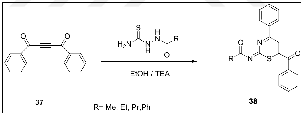
Şekil 2.48. 2-Aryoylimino-4-fenil-6-benzoil-1,3-tiazinlerin sentezi
