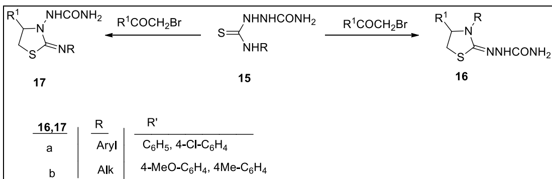
Şekil 2.39. 4-Ariltiazolin sentezi
