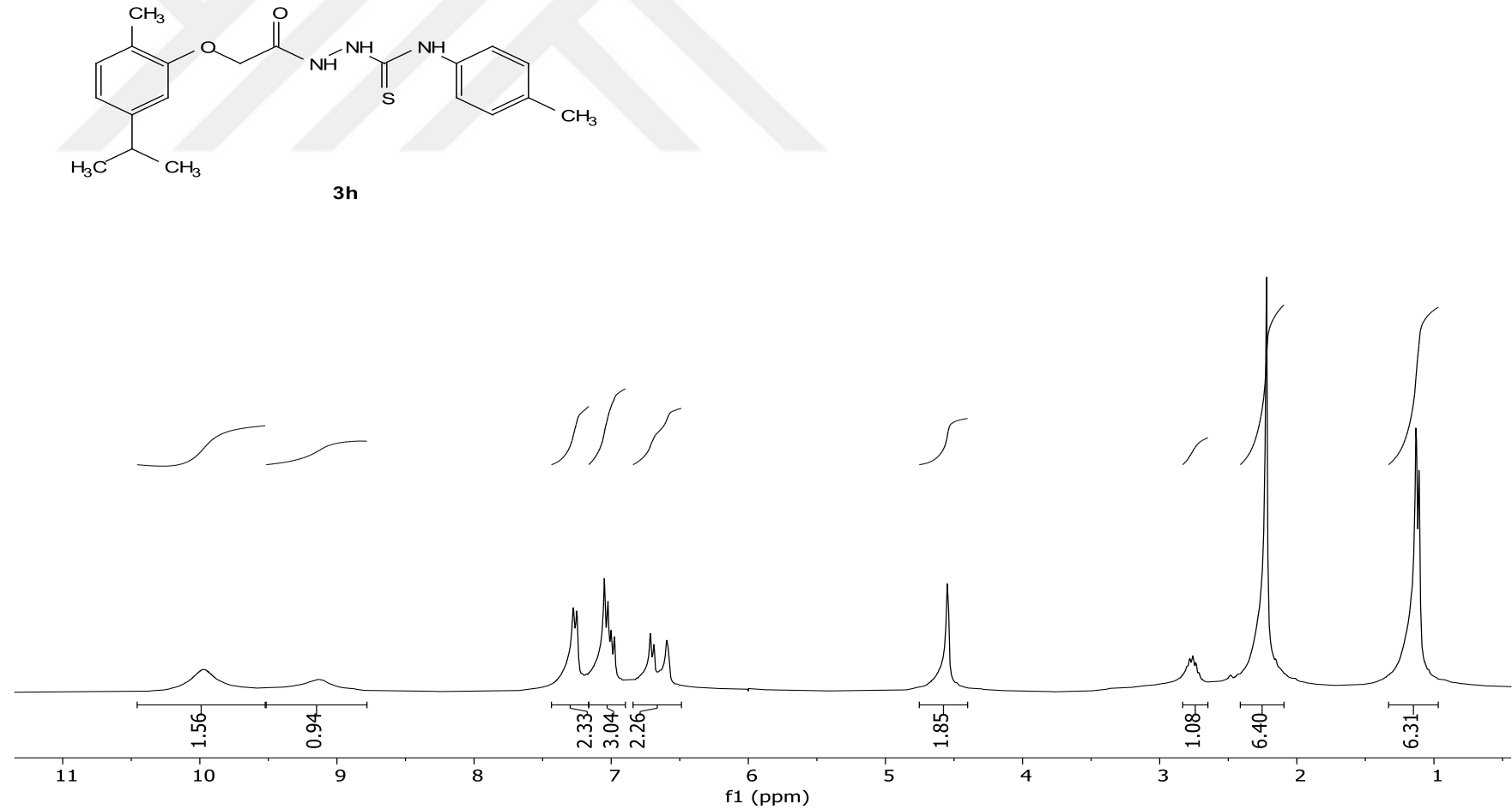
EK-19. (3h) bileşiğinin ^1\text{H} NMR spektrumu (300 MHz, DMSO- d_6 )
