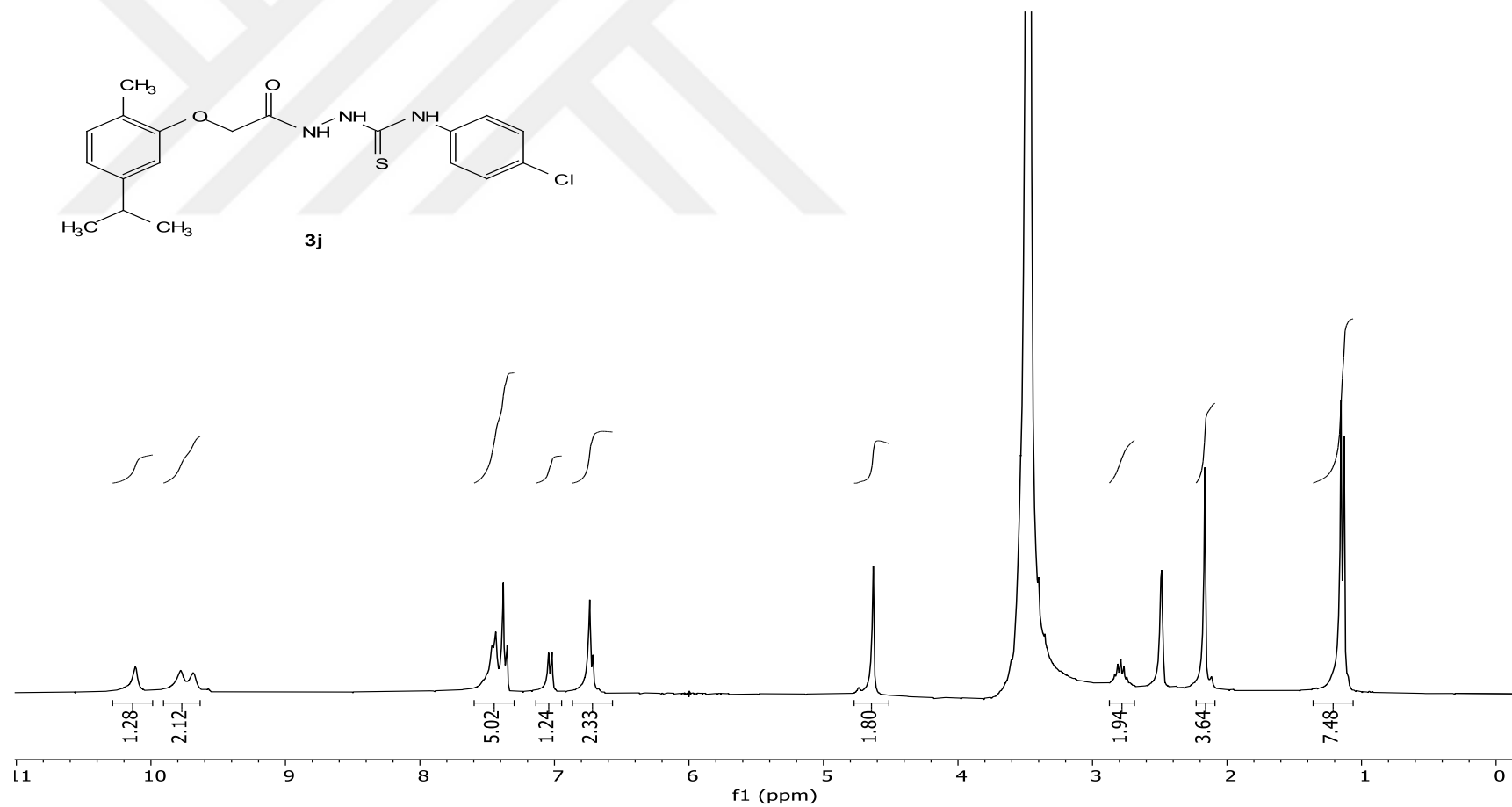
EK-23. (3j) bileşiğinin ^1\text{H} NMR spektrumu (300 MHz, \text{CDCl}_3 + \text{DMSO-d}_6 )
