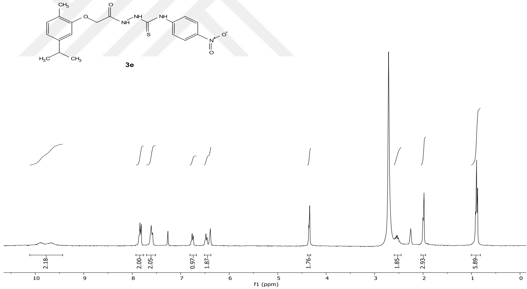
EK-13. (3e) bileşiminin ^1\text{H} NMR spektrumu (300 MHz, DMSO- d_6 )
