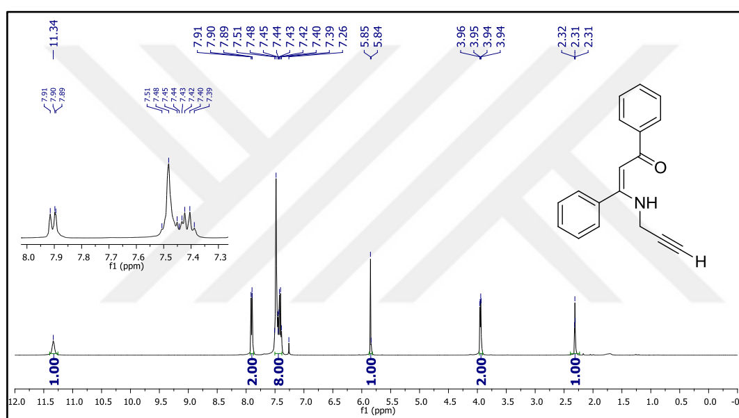
Figure 13. ^1\text{H} NMR spectrum of (Z)-1,3-diphenyl-3-(prop-2-yn-1-ylamino)prop-2-en-1-one ( 26a ).
