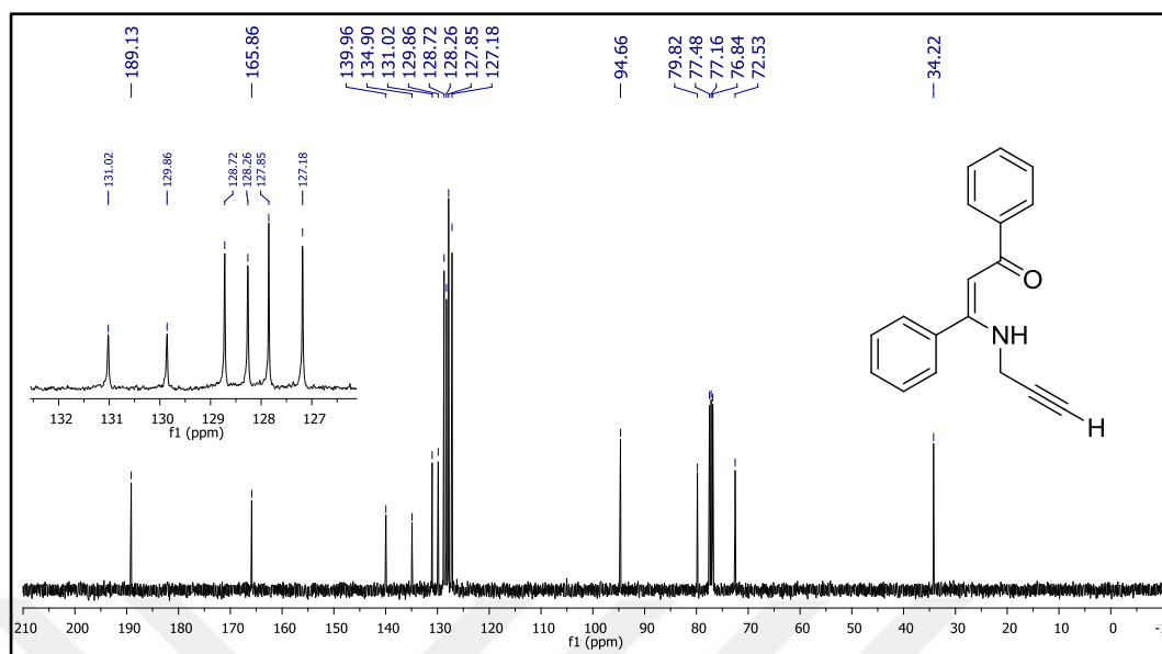
Figure 14. ^{13}\text{C} NMR spectrum of (Z)-1,3-diphenyl-3-(prop-2-yn-1-ylamino)prop-2-en-1-one ( 26a ).
