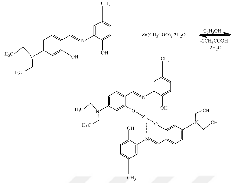
Şekil 3.5. 4-Dietilaminosilisiliden-2-amino-4-metilfenol Ligandının \text{Zn}(\text{II}) Kompleksi
