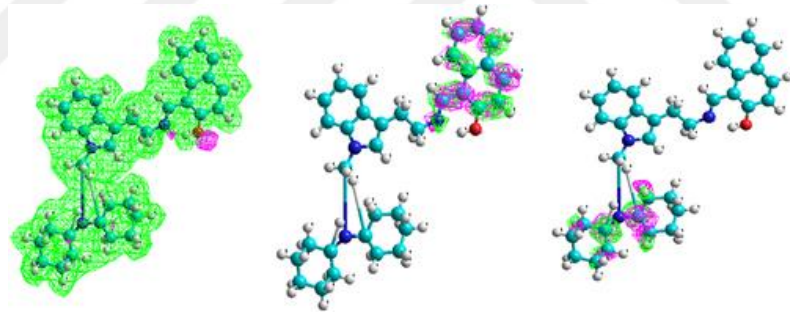
Şekil 2.14. HL Ligandı için Elektostatik Potansiyel (HOMO ve LUMO)
