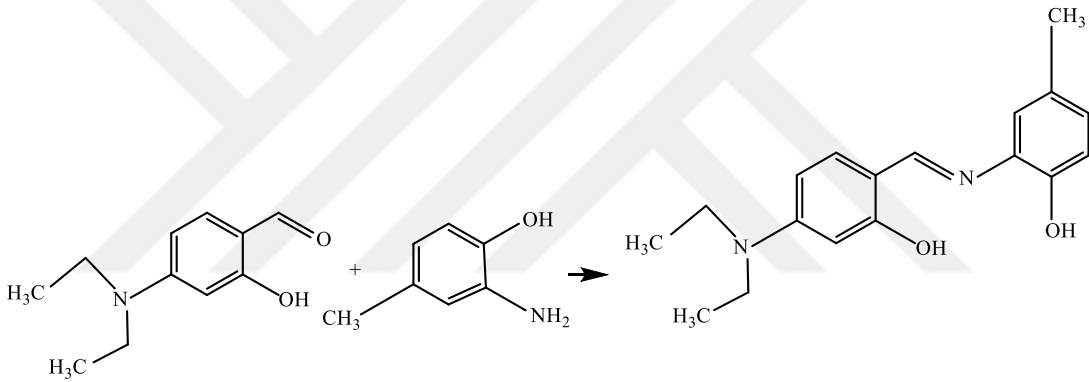
Şekil 3.1. 4-Dietilaminosalisiliden-2-amino-4-metilfenol
