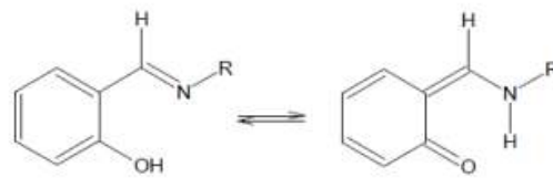
Şekil 2.2. Schiff Bazlarında Tautomerizim
