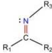
Şekil 2.1. Schiff Bazının Genel Yapısı
