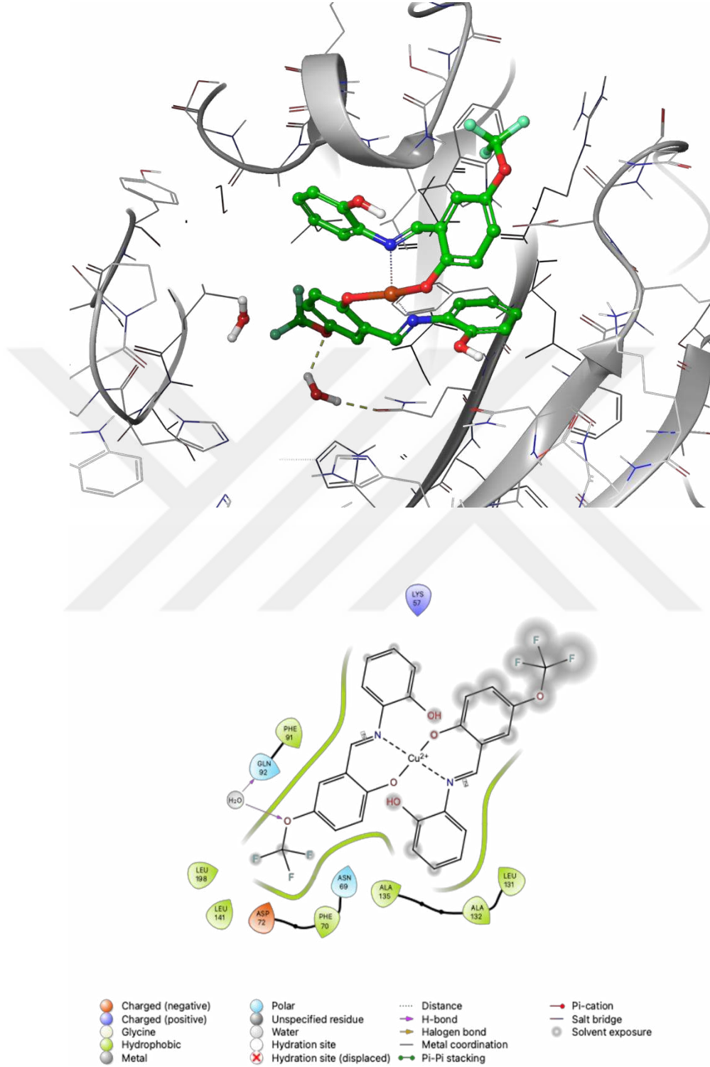
Şekil 4. 13. Moleküler Kenetlenme Sonucunda Elde Edilen CuL 2 – hCA I (PDB ID: 1AZM) Etkileşim Diyagramı
