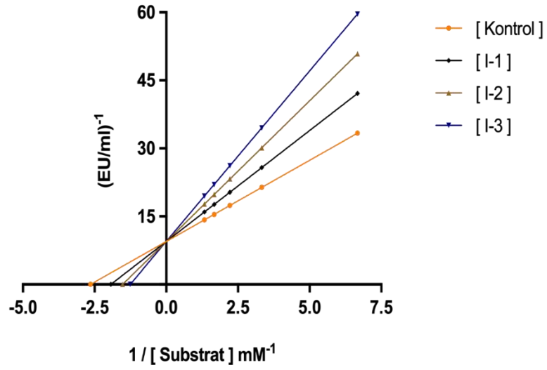
Şekil 4. 5. Yeni Sentezlenen Schiff Bazı Türevi Olan \text{CuL}_2 Bileşiğinin h\text{CA I} İzoenzimi Aktivitesi Üzerine Etkisini Gösteren ve K_I Sabitinin Belirlenmesi İçin Kullanılan Lineweaver-Burk Grafiği
