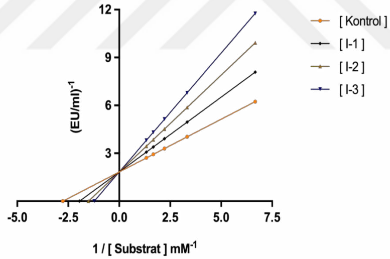
Şekil 4. 8. Yeni Sentezlenen Schiff Bazı Türevi Olan LH Bileşiğinin hCA II İzoenzimi Aktivitesi Üzerine Etkisini Gösteren ve K_I Sabitinin Belirlenmesi İçin Kullanılan Lineweaver-Burk Grafiği
