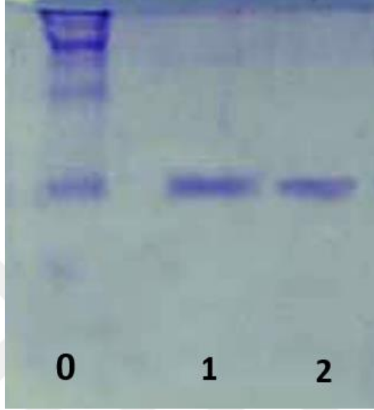
řekil 4. 2. SDS-PAGE Elektrofözezi Karakterizasyon Grseli (0: Standart 1: h CA I Enzimi, 2: h CA II Enzimi)
