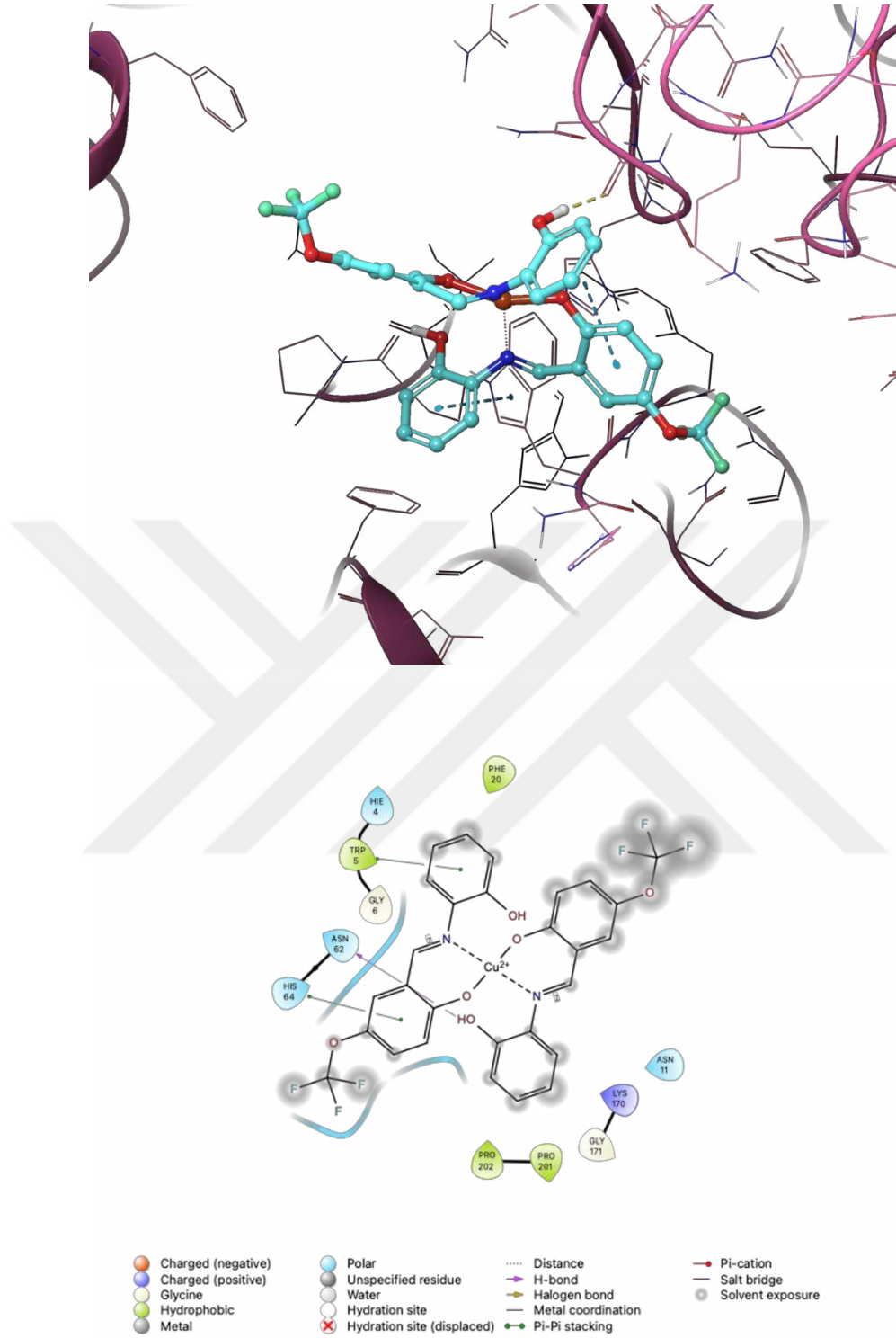
Şekil 4. 14. Moleküler Kenetlenme Sonucunda Elde Edilen CuL 2 – hCA II (PDB ID: 3HS4) Etkileşim Diyagramı
