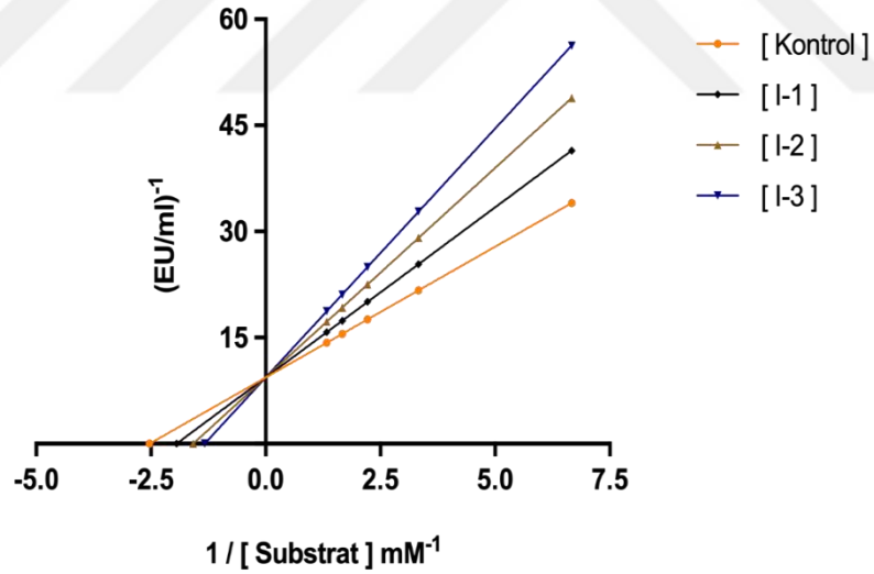
Şekil 4. 6. Yeni Sentezlenen Schiff Bazı Türevi Olan \text{NiL}_2 Bileşiğinin h\text{CA I} İzoenzimi Aktivitesi Üzerine Etkisini Gösteren ve K_I Sabitinin Belirlenmesi İçin Kullanılan Lineweaver-Burk Grafiği
