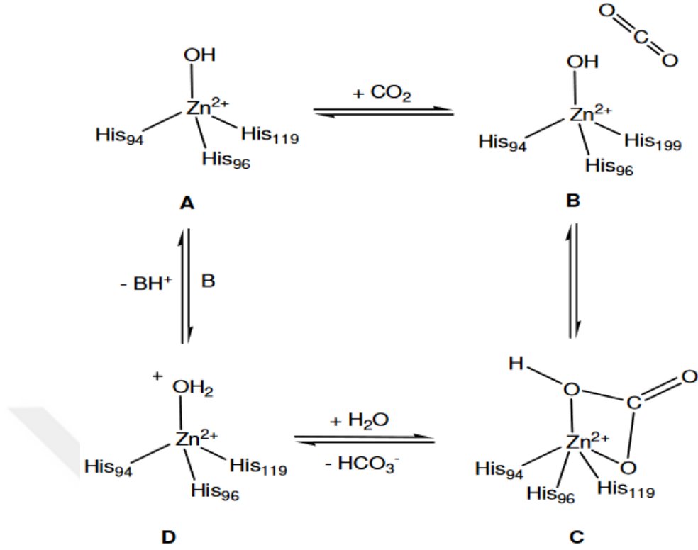
Şekil 2. 8. CA'nın Katalizlediği CO 2 -Hidratasyon Tepkimesi Mekanizmasının Görseli.
