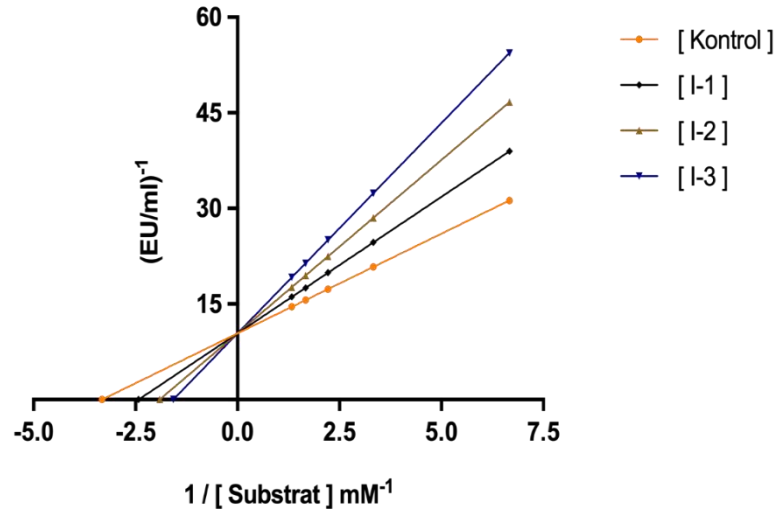
Şekil 4. 7. Yeni Sentezlenen Schiff Bazı Türevi Olan ZnL_2 Bileşiğinin hCA I İzoenzimi Aktivitesi Üzerine Etkisini Gösteren ve K_I Sabitinin Belirlenmesi İçin Kullanılan Lineweaver-Burk Grafiği
