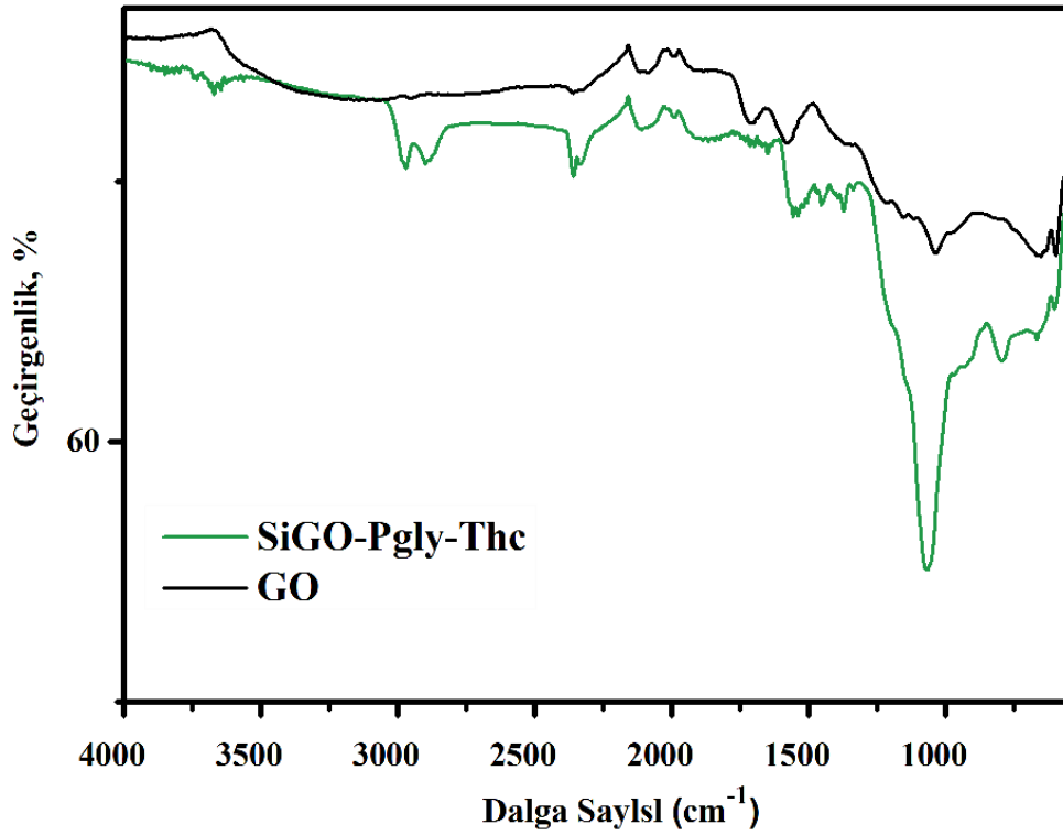
Şekil 8. 3. SiGO-Pgly-Thc hibrit nanokompozite ait FT-IR spektrumları.
