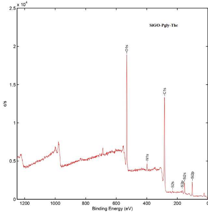
Şekil 5. 13. SiGO-Pgly-Thc hibrit nanokompozite ait XPS spektrumu.
