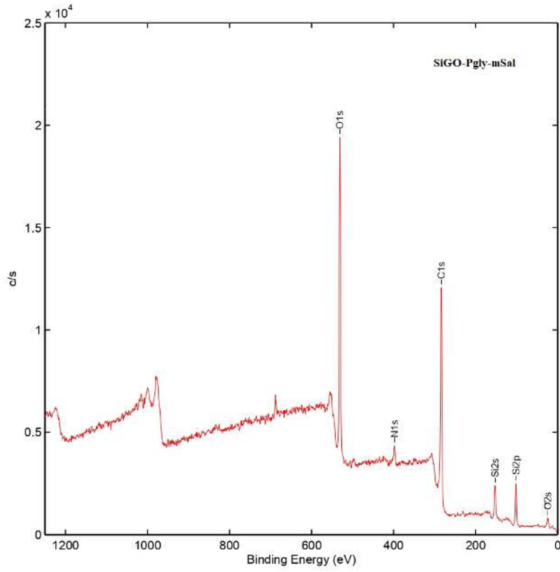
Şekil 5. 12. SiGO-Pgly-mSal hibrit nanokompozite ait XPS spektrumu.
