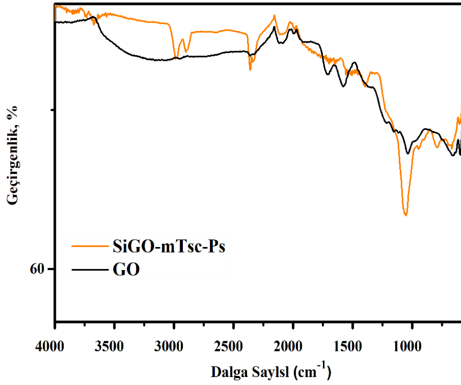
Şekil 8. 4. SiGO-mTsc-Ps hibrit nanokompozite ait FT-IR spektrumları.
