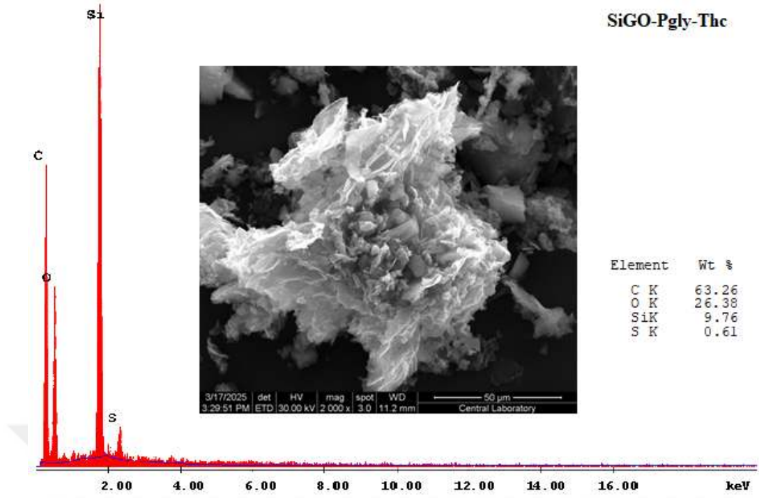
Şekil 8. 8. SiGO-Pgly-Thc hibrit nanokompozite ait SEM-EDX analizi.
