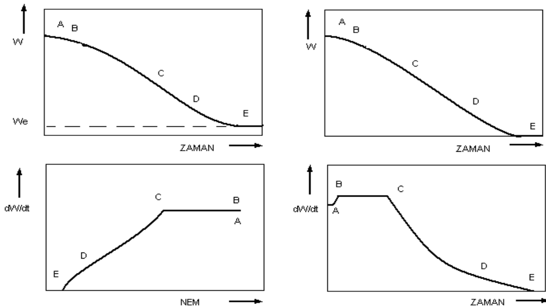
Şekil 2.1 Karakteristik kuruma eğrileri
