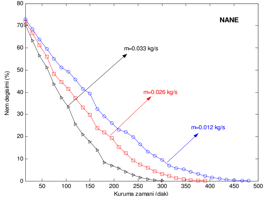
Şekil 4.25 Nane için nem değişiminin zamana göre değişimi
