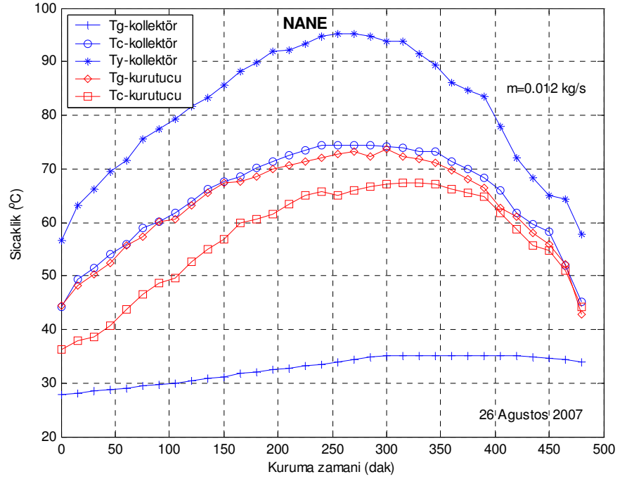
Şekil 4.30 Nane kurutulmasında sıcaklıkların zamana göre değişimi ( m=0.012 \text{ kg/s} )
