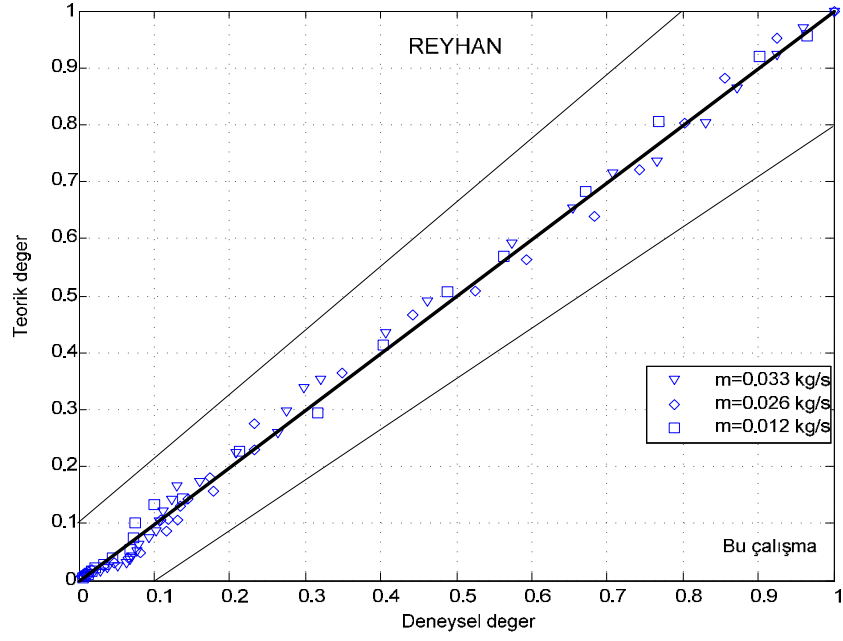
Şekil 4.52 Reyhan için teorik değerlerin deneysel değerlere göre değişimi (Bu çalışma)
