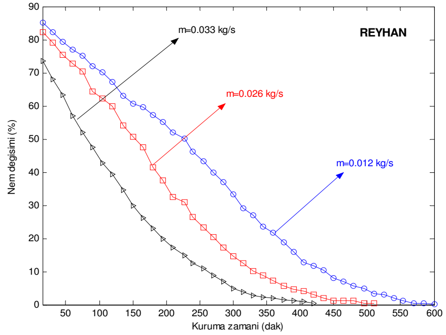
Şekil 4.26 Nane için nem değişiminin zamana göre değişimi
