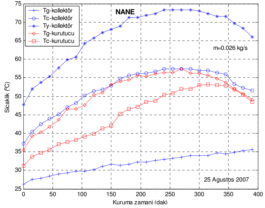
Şekil 4.29 Nane kurutulmasında sıcaklıkların zamana göre değişimi ( m=0.026 \text{ kg/s} )
