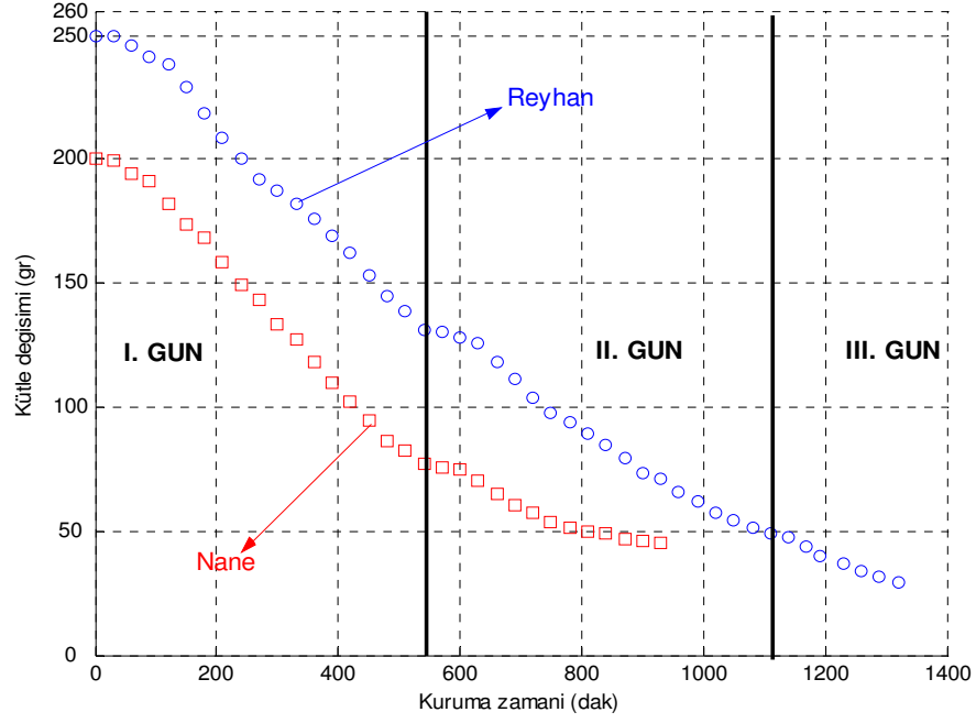
Şekil 4.11 Nane ve reyhan için doğal kurutma şartlarında kütlenin değişimi
