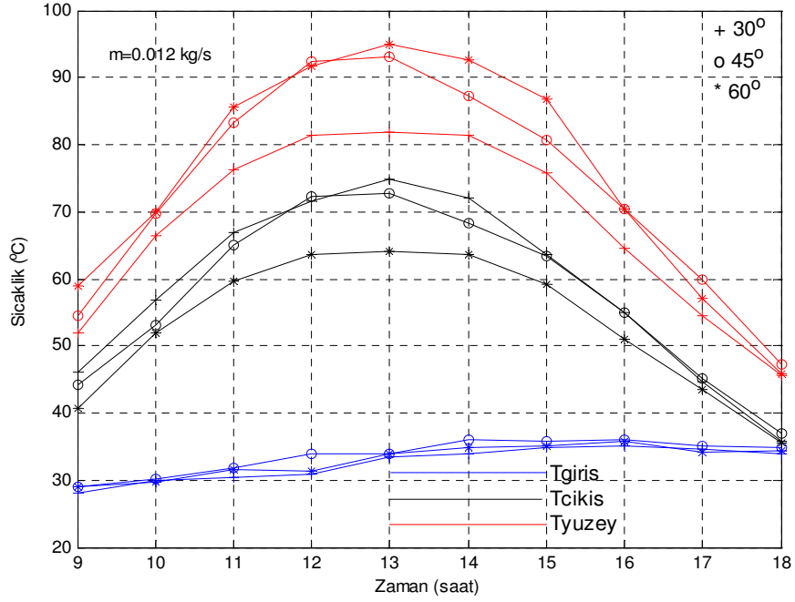
Şekil 4.7 \dot{m} = 0.012 \text{ kg/s} için sıcaklıkların günün zamanına göre değişimi
