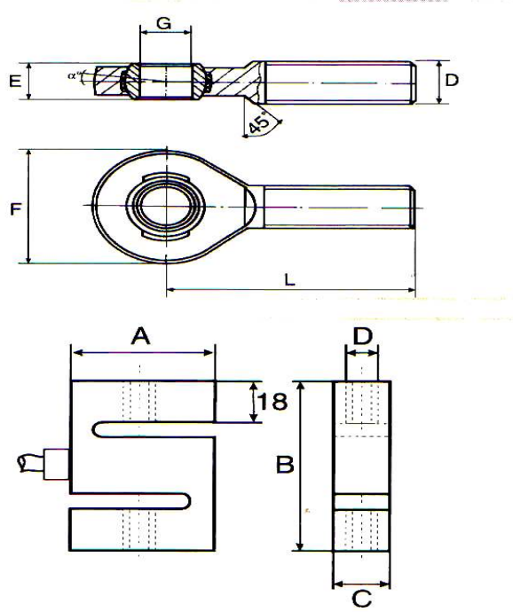
  ekil 3.11 K25-FKA0251 Gerilme ve sıkı  tırma sens  r  n  n (streng  ) teknik resim detayı
