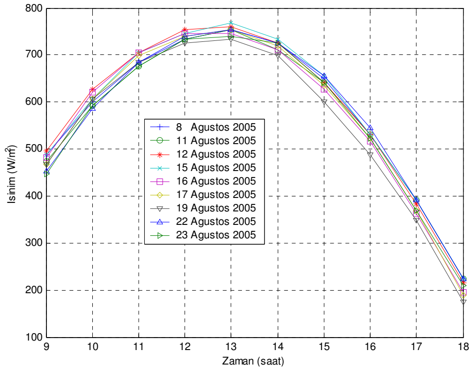
Şekil 4. 1 Kollektör deneylerinin yapıldığı günlere ait ışınlm değerlerinin günün zamanına göre değişimi
