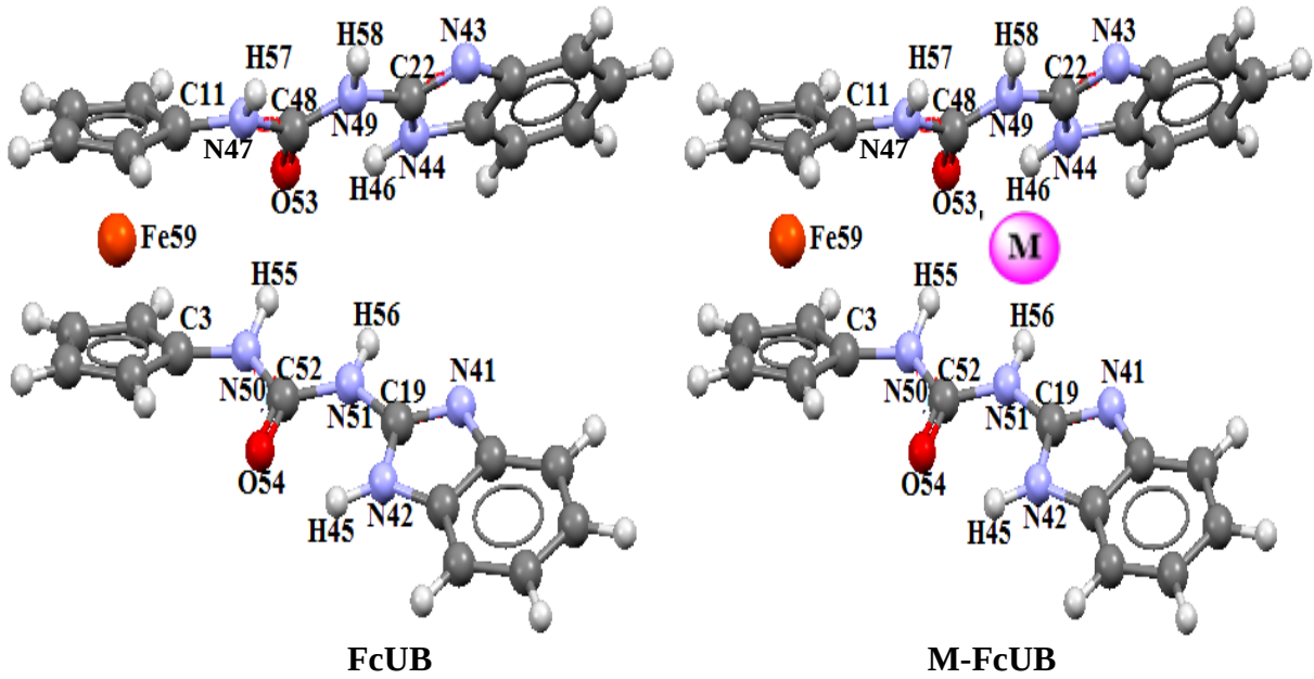
Şekil 15. Hesaplanan yapıların atom numaraları
