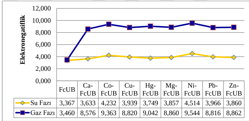
Şekil 18. Gaz ve su fazları için elektonegatiflik değerleri
