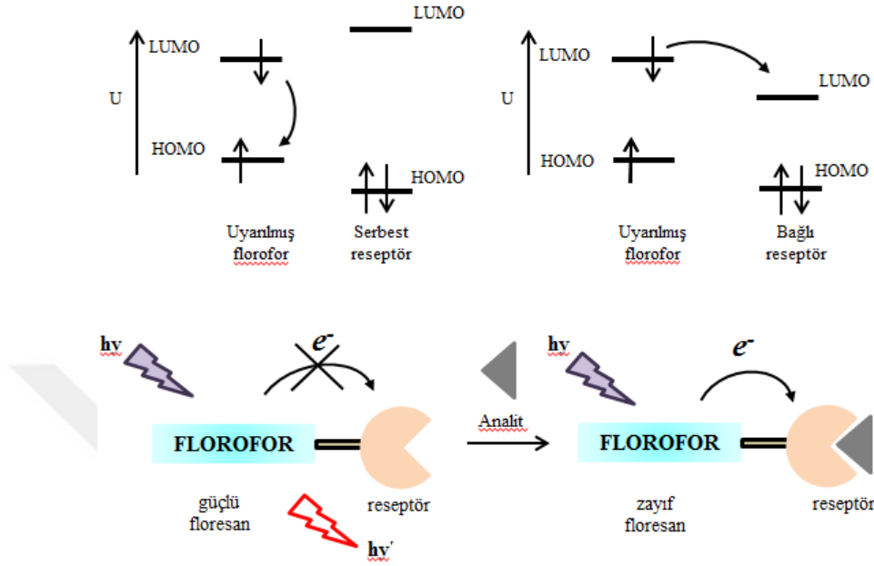
Şekil 8. Oksidatif PET mekanizmasının şematik gösterimi
