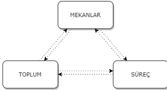
Şekil 6.1. Hipotez üçgeni.
