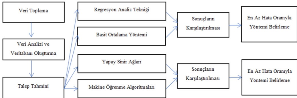
Şekil 4.1. Yolcu talep tahmini için çalışmanın adımları
