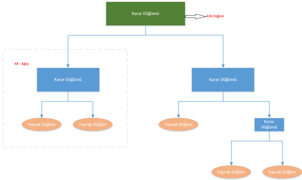
 ekil 3.3. Karar a acı diyagramı (Noviantoro ve Huang, 2021).
