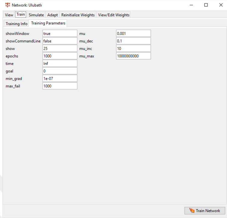
Şekil 4.13. Ulubatlı istasyonu matlab eğitim parametreleri ekranı
