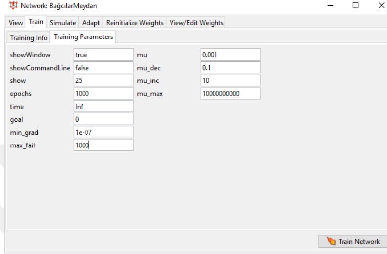
Şekil 4.29. Bağcılar Meydan istasyonu matlab eğitim parametreleri ekranı
