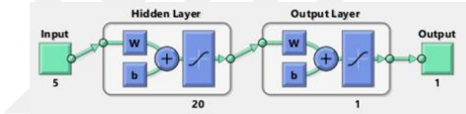
Şekil 4.2. Modeli en başarılı sonuca ulaştıran yapay sinir ağı mimarisi
