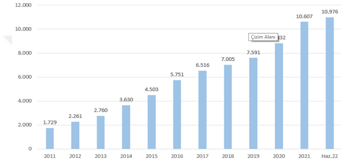
Şekil 4. 4. Türkiye’de rüzgar enerjisine dayalı kurulu güç grafiği (Anonim 1)
