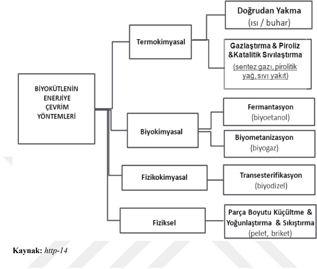
Şekil 2.10. Biyokütle Çevrim Yöntemleri
