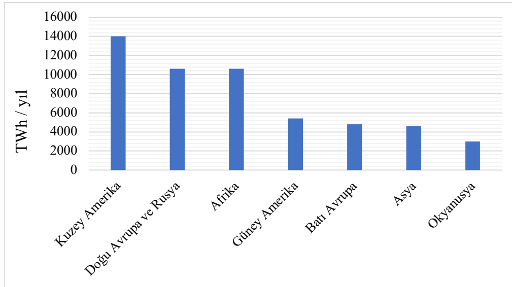
Şekil 2.6. Rüzgâr Potansiyelinin Dağılımı
