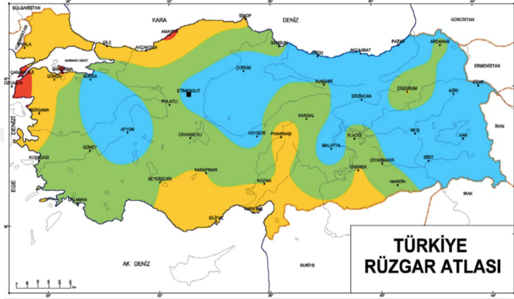
Görsel 3.2. Türkiye Rüzgâr Atlası
