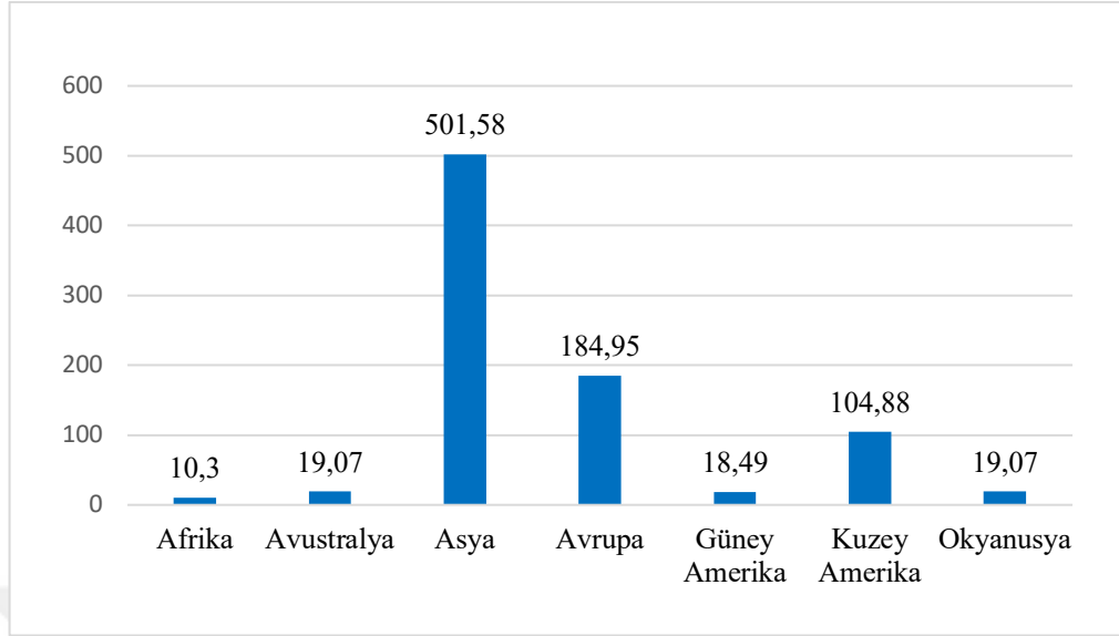
Şekil 2.5. Kıtaların Kurulu Güneş Enerjisi Kapasitesi, GW
