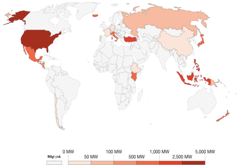
Şekil 2.8. Kurulu Jeotermal Enerji Kapasitesi, 2020
