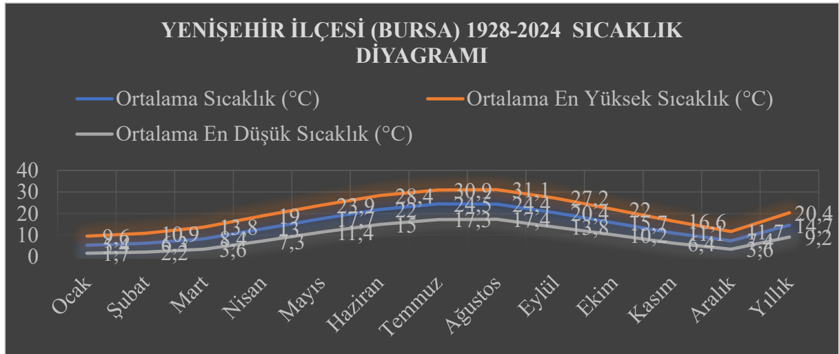
Grafik 2.1 Yenisehir İlçesi (Bursa) 1928-2024 Sıcaklık Diyagramı
