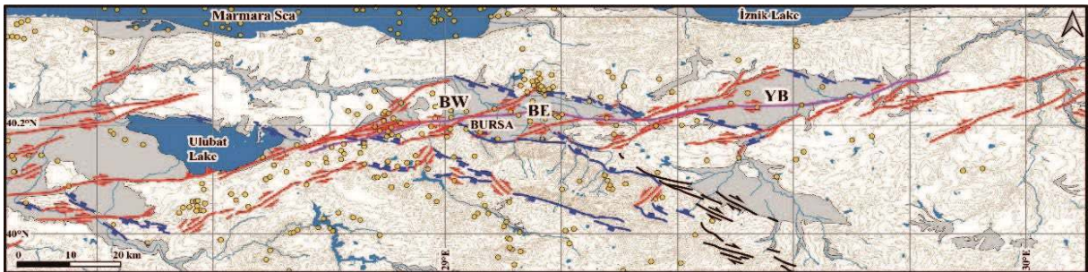
Harita 2.2 Bursa ve Çevresinde Çek-Ayır Havzalar ve Havza Biçen Faylar
