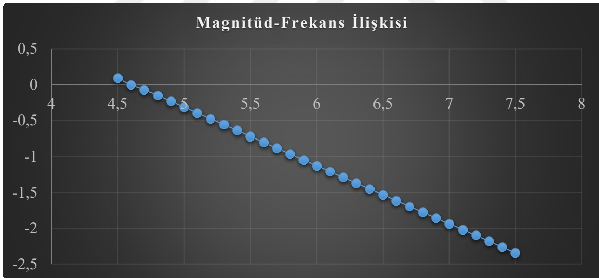
Grafik 3.1 Yenişehir Magnitüd-Frekans İlişkisi
