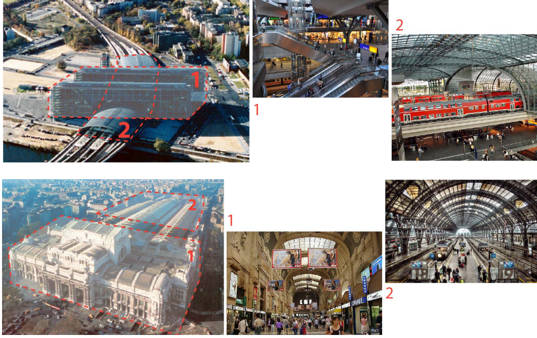
Şekil 3.13 : Berlin Merkezi Tren İstasyonu (üstte) ve Milano Merkezi Tren İstasyonu'ndaki (altta) yolcu ve araç mekanlarının ayrımı.
