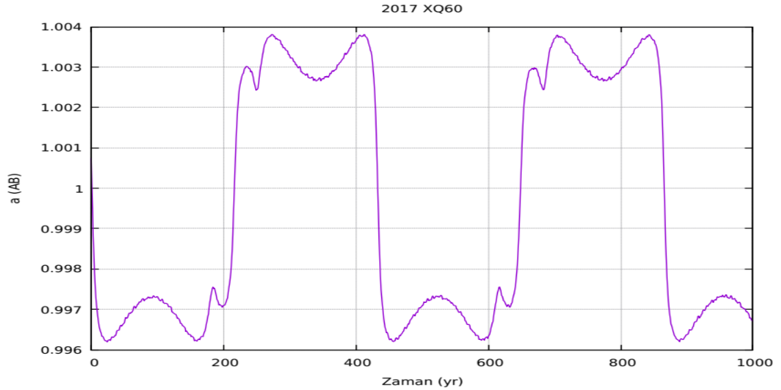
Şekil 4.41. 2017 XQ60 asteroidine ait zaman-yarı büyük eksen grafiği
