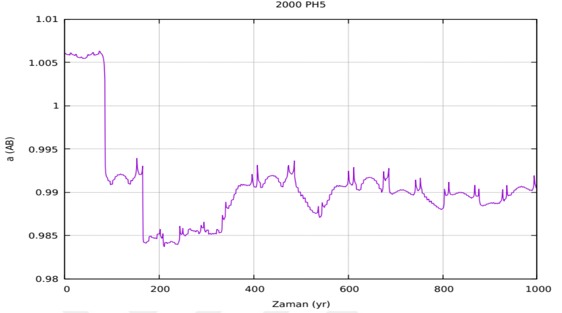
Şekil 4.17. 2000 PH5 asteroidine ait zaman-yarı büyük eksen grafiği
