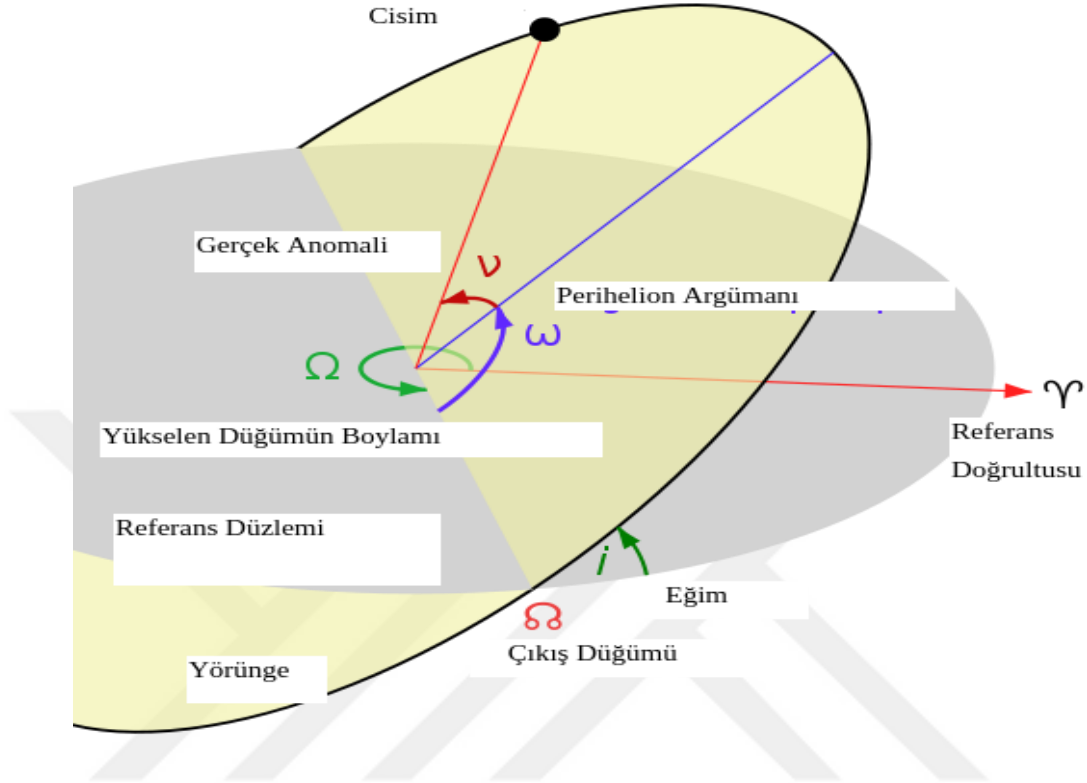
Şekil 2.2. Yörünge elemanları
