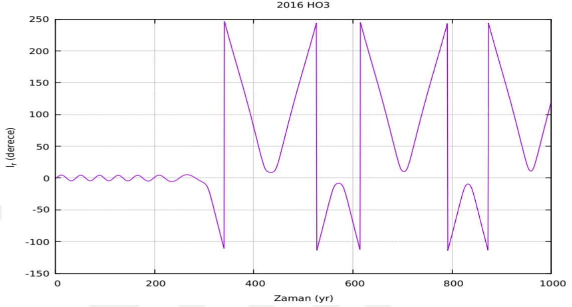
Şekil 4.14. 2016 HO3 asteroidine ait zaman-rölatif ortalama boylam grafiği
