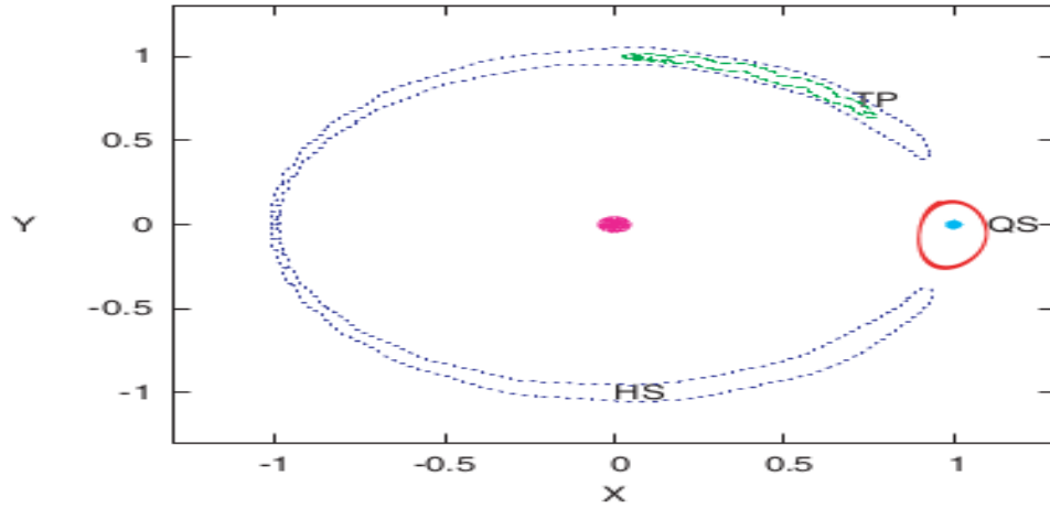
Şekil 2.4. At nalı (HS), İribaş (TP) ve yarı-uydu (QS) eş yörüngelerinin dönen referans çerçevesinde temsili gösterimi (Mikkola vd. 2006)
