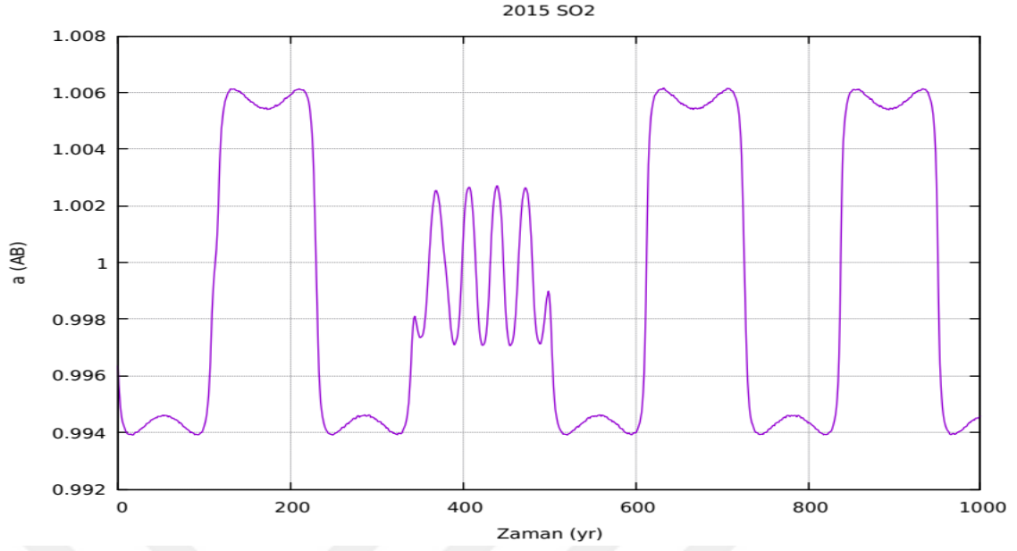
Şekil 4.29. 2015 SO2 asteroidine ait zaman-yarı büyük eksen grafiği
