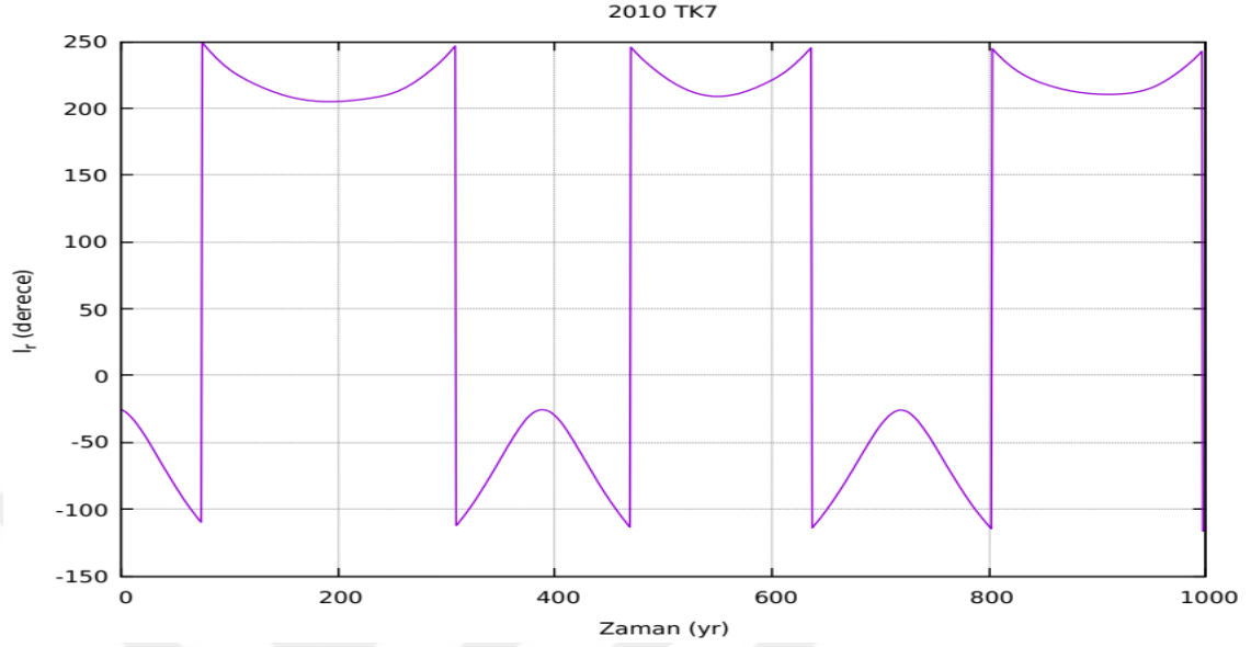
Şekil 4.2. 2010 TK7 asteroidine ait zaman-rölatif ortalama boylam grafiği
