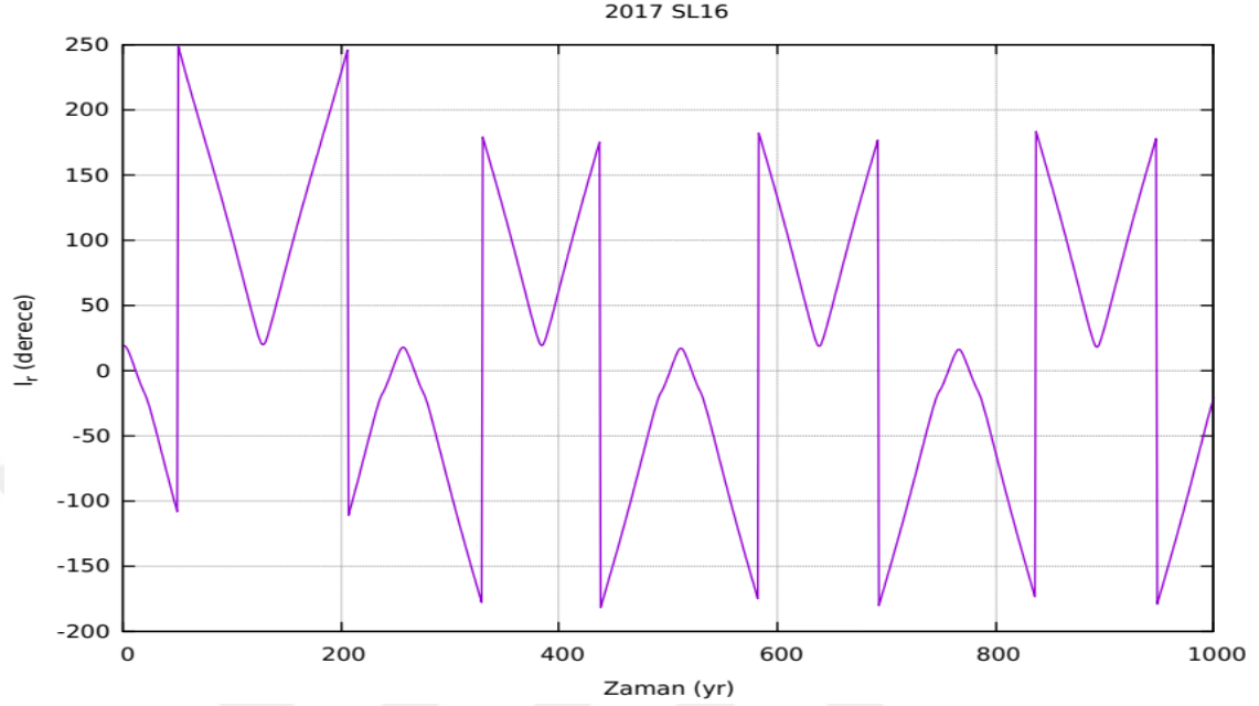
Şekil 4.40. 2017 SL16 asteroidine ait zaman-rölatif ortalama boylam grafiği
