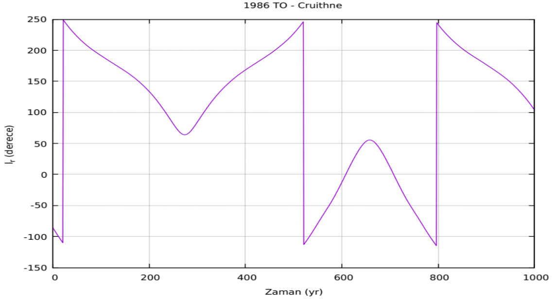
Şekil 4.16. Cruithne (1986 TO) asteroidine ait zaman-rölatif ortalama boylam grafiği
