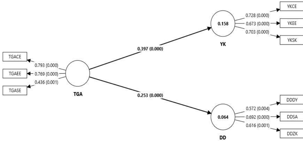
Şekil 7. Yapısal Model Sonuçları
