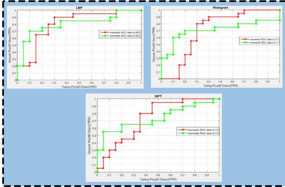
Şekil 4.14. YSA ROC alanlarının karşılaştırılması
