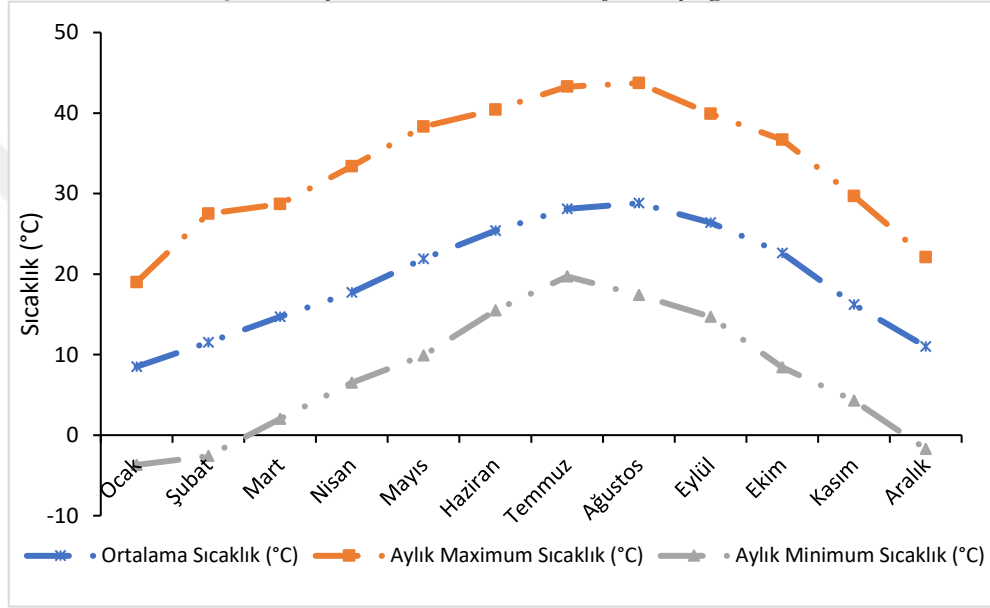
Şekil 4. Çukurova'nın Termik Rejim Diyagramı
