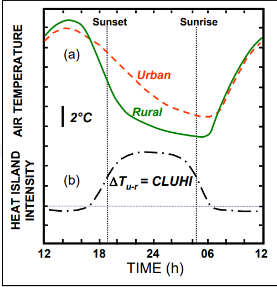
Şekil 2. Isı Adası ve Hava Sıcaklığının Değişimi
