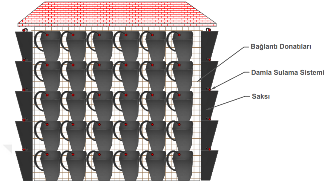
Şekil 3.9. Yeşil duvar sistemi, bağlantı ve sulama ekipmanları
