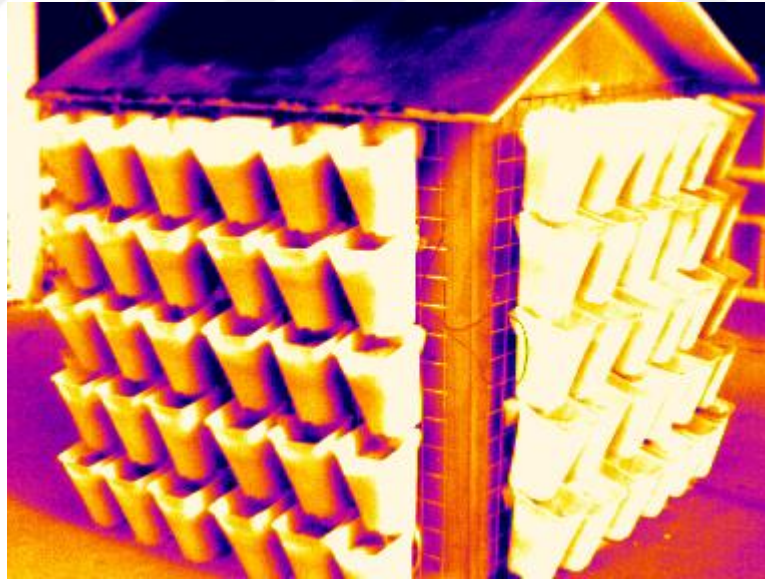
Şekil 4.5. Yalnız yetiştirme ortamı bulunan yeşil duvar uygulamasının termal görüntüsü
