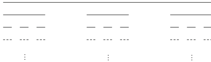
Şekil 5.9. 5-lü Cantor kümesi
