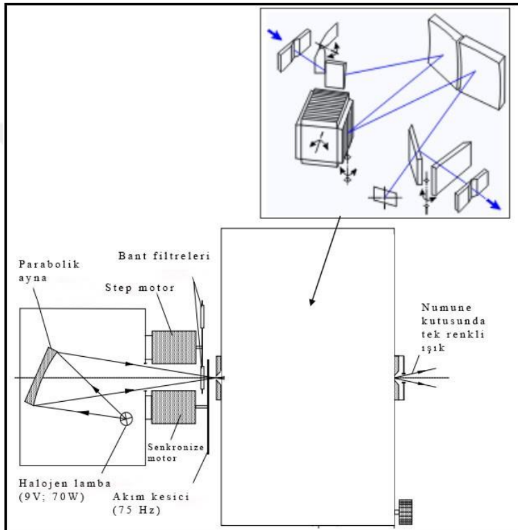
Şekil 3.2. Spektral ölçüm için kullanılan sistemin halojen lamba kutusu ve monokromatörün iç optik yapısı (Ioffe 2010)
