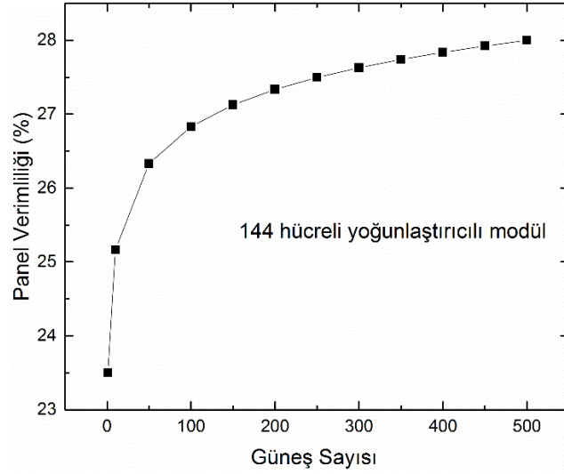
Şekil 4.13. 144 adet GaInP/GaAs/Ge üç eklemlili güneş hücresi içeren yoğunlaştırıcı panelin güneş sayısına göre verimliliğinin değişimi
