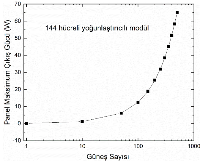
Şekil 4.14. 144 adet GaInP/GaAs/Ge üç eklemlili güneş hücresi içeren yoğunlaştırıcı panelin güneş sayısına göre maksimum güç değerinin değişimi
