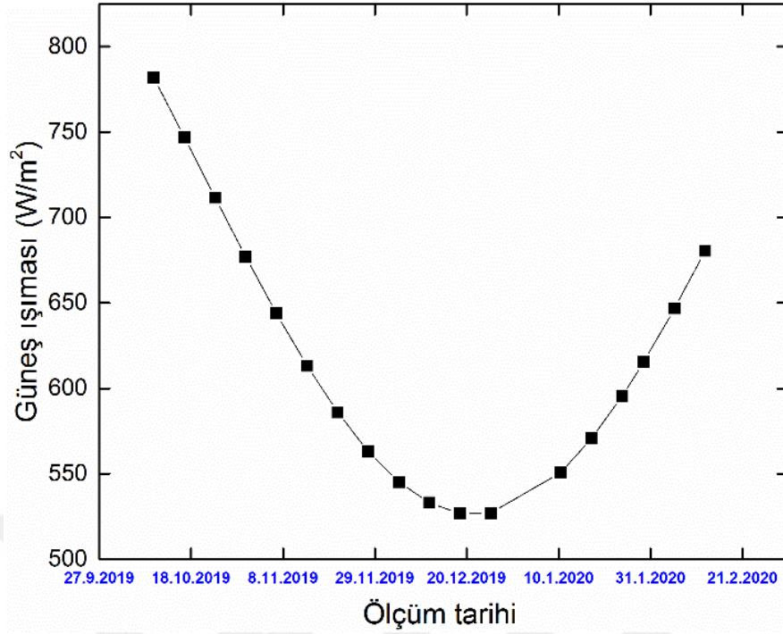
Şekil 4.12. 10 Ekim 2019 – 13 Şubat 2020 tarihler arasında güneş ışıının birim alana düşen gücünün değişimi
