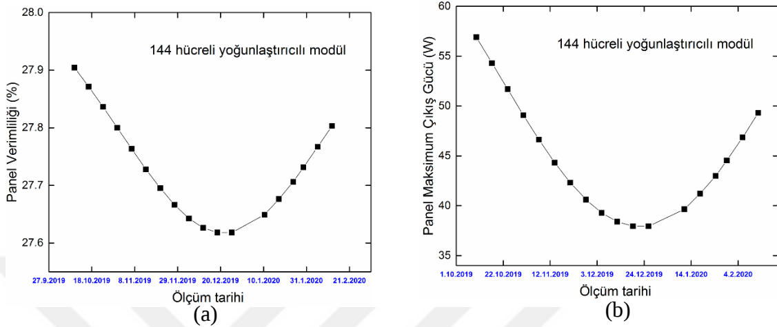
Şekil 4.15. 144 adet GaInP/GaAs/Ge üç eklemlı güneş hücresi içeren yoğunlaştırıcı panelin 2019 Eylül ve 2020 Şubat ayları arasında ölçülmüş a) verimlilik; b) maksimum güç değerlerinin zamana göre dağılımı
