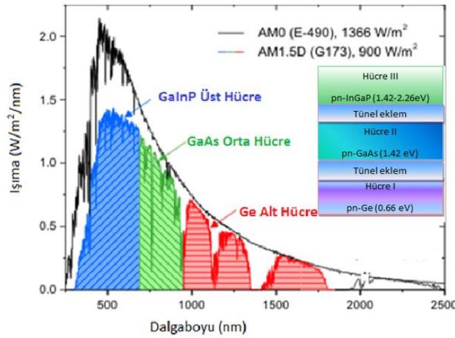
Şekil 2.9. GaInP/GaAs/Ge çok eklemlı güneş hücresinin şematik yapısı ve güneş spektrumunun hangi bölgelerini soğurduğunu gösteren spektral dağılımı
