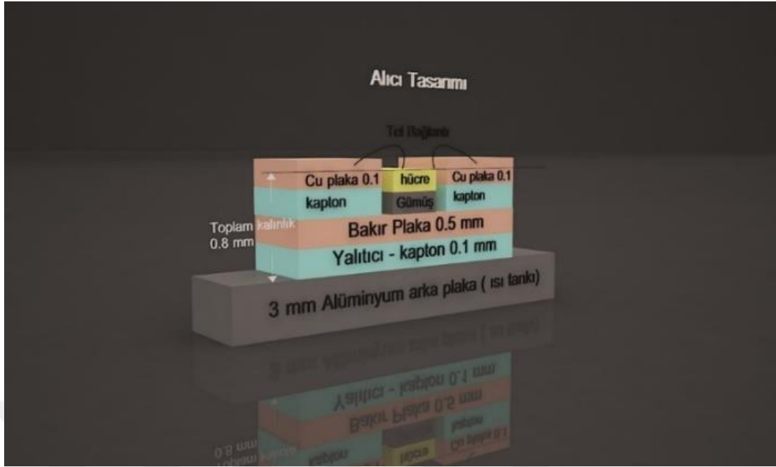
Şekil 3.4. Yoğunlaştırıcı modül içerisinde güneş hücresi ve alıcı tasarımının şematik olarak gösterimi
