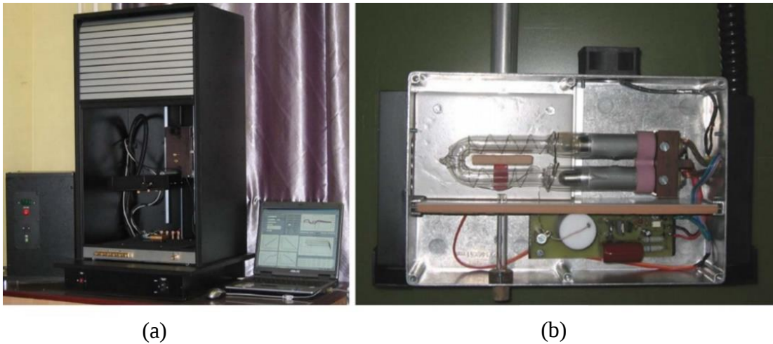
Şekil 3.12. GaInP/GaAs/Ge üç eklemlü güneş hücresi için akım-voltaj ölçüm sistemi, (a) genel dış görünümü ; (b) 10ms gibi kısa sürede flaş ışık vermek için kullanılan Xenon lamba kutusunun iç görünümü
