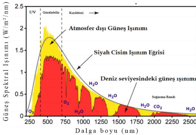
Şekil 2.1. AM0 ve AM1.5 standartlarında güneş spektrumu ve kara cisim ışıma spektrumunun karşılaştırılması. Güneş ışınlarının dünya atmosferine girdiğinde spektrumun hangi bölgelerinde ve hangi moleküller tarafından soğurulduğunu gösteren soğurma bölgeleri (Kitai 2011)
