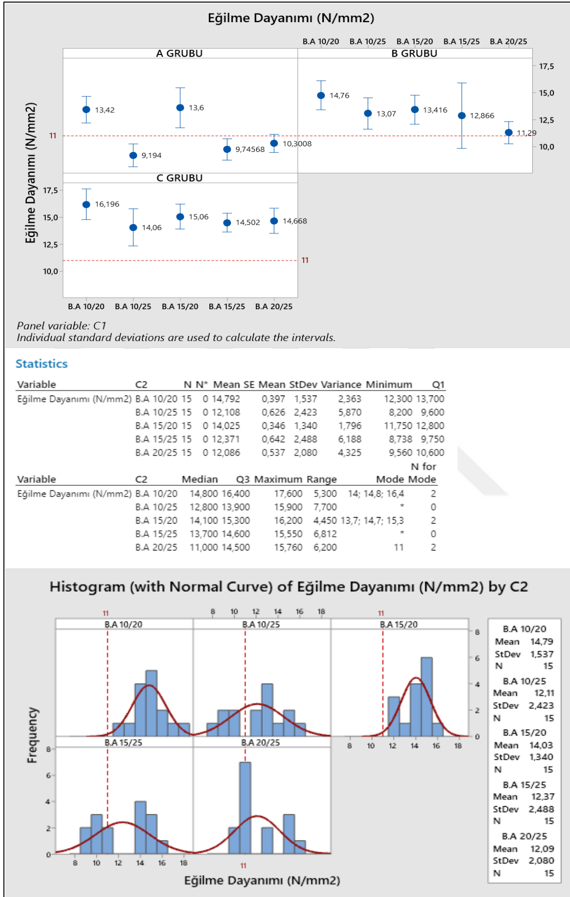
Şekil 4.12: Eğilme dayanımı test sonuçları
