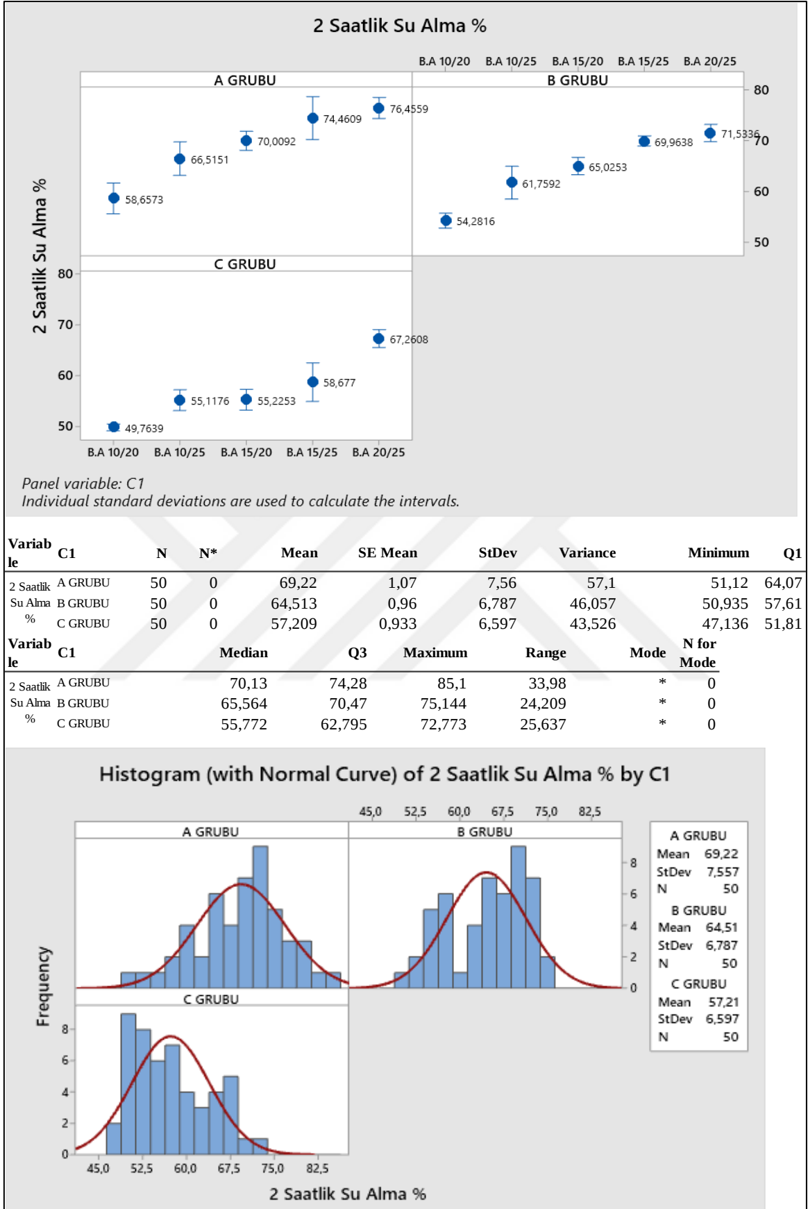
Şekil 4.2: İki saatlik su alma sonuçlarının gruplara göre dağılımı
