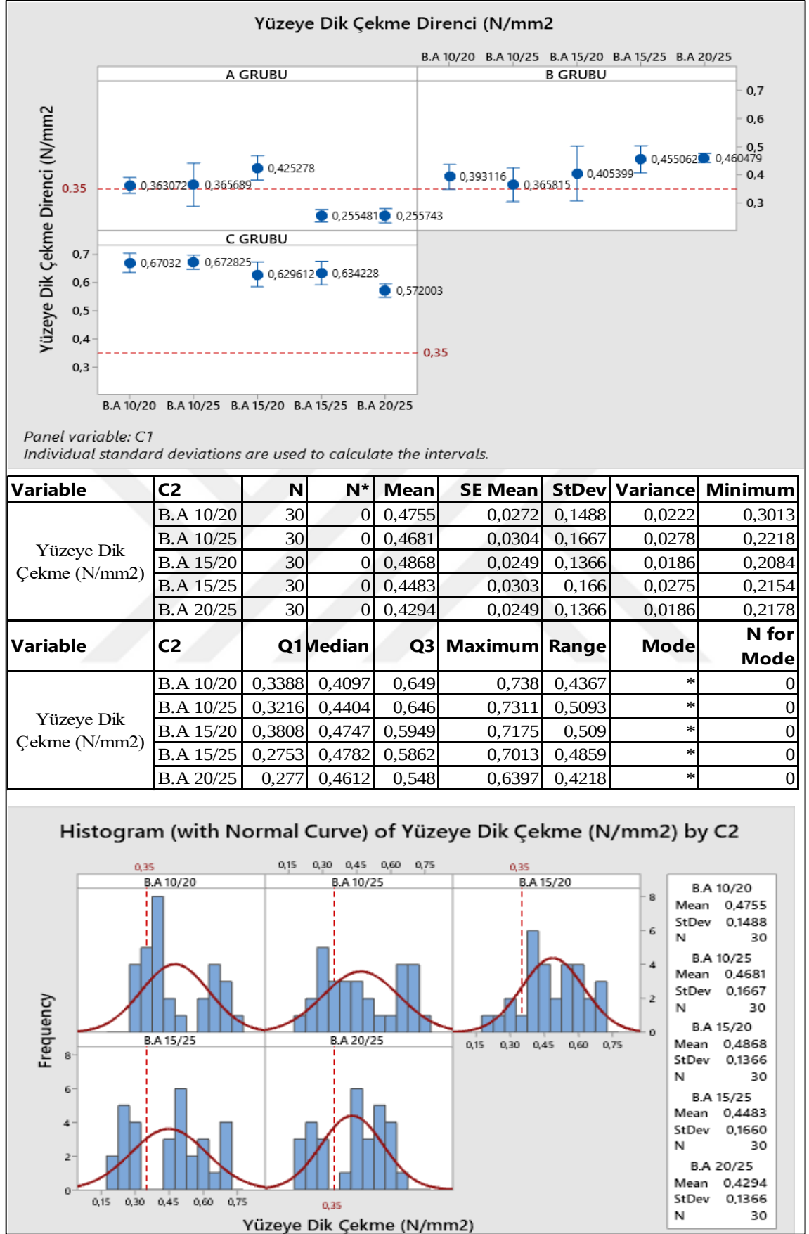
Şekil 4.16: Yüzeye dik çekme direnci test sonuçları
