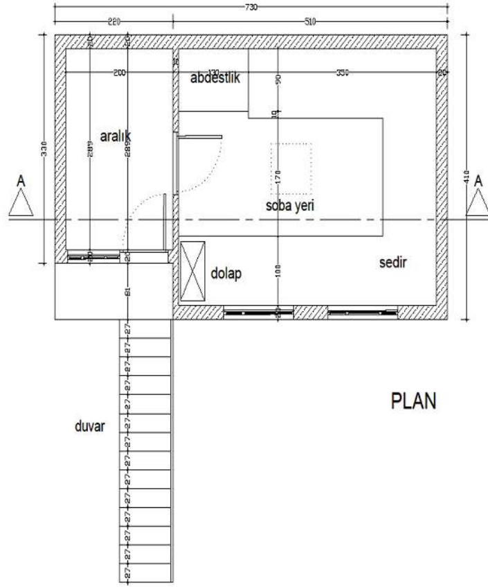
Resim 3.128. Koca Emrullah'ın Köy Odası Planı
