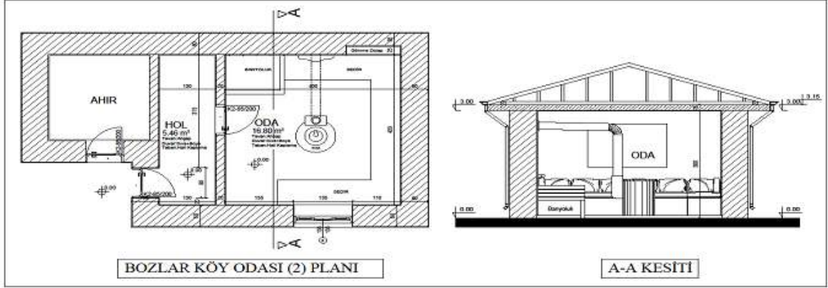
Resim 3.44. Oda Planı
