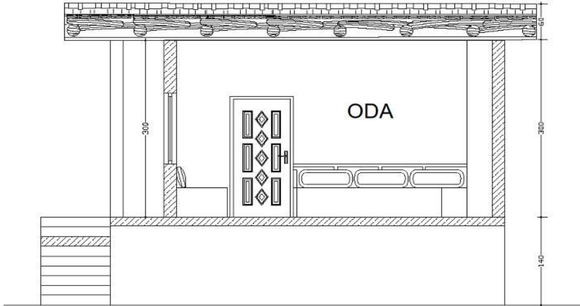
Resim 3.96. K y Odası Kesiti
