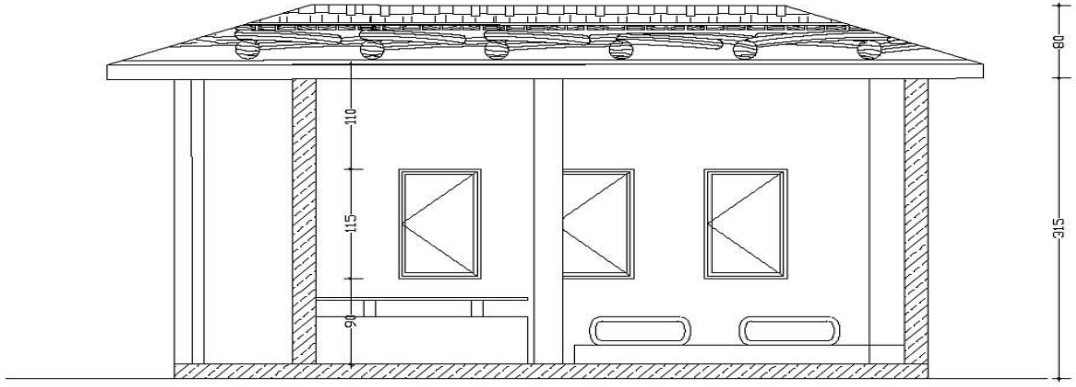
Resim 3.68. Oda Kesiti
