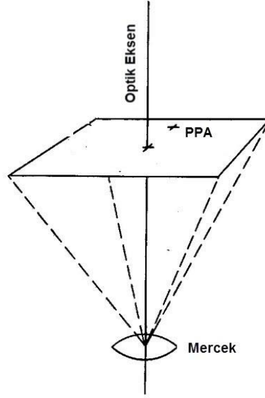
Şekil 4. 16. Optik eksen ve kayıklık değeri (http-6)
