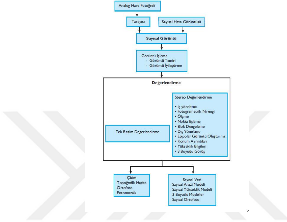
Şekil 4. 4. Fotogrametrik iş akış planı
