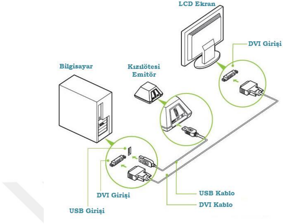
Şekil 5. 4. Stereo sistem donanımları ve bağlantıları ( Http-8 )
