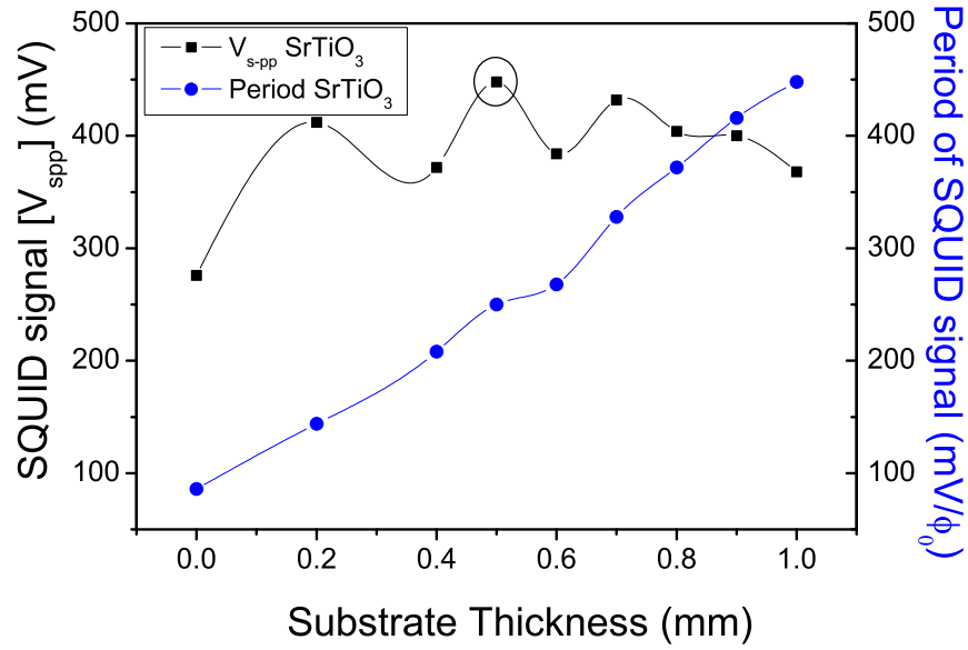
(b) SrTiO_3
