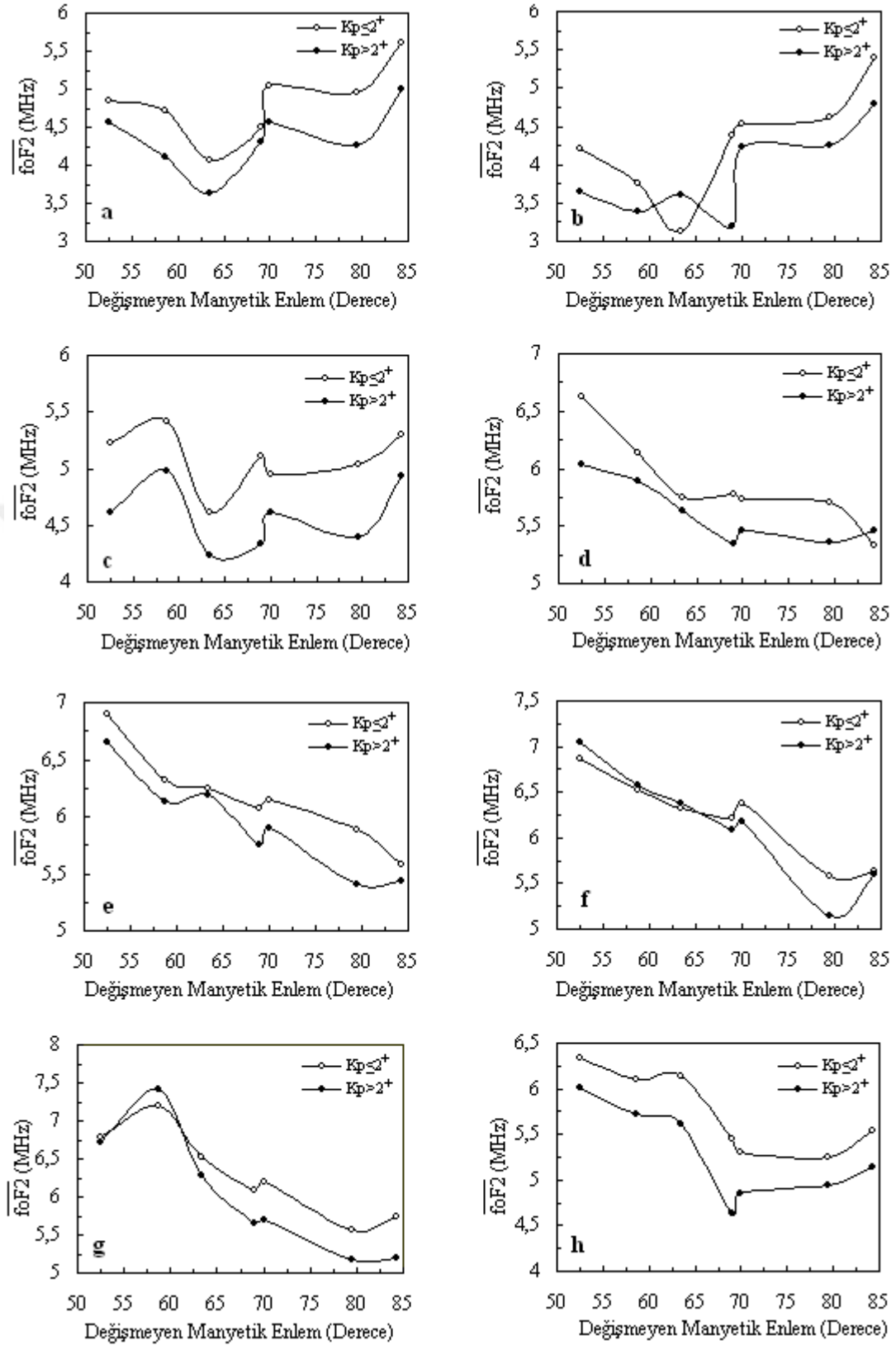
Şekil 4.4. 1972 yılı 21 Haziran döneminde K_p indisinin pasif ve aktif durumlar için farklı istasyonlardan alınan saatlik ortalama f_oF2 değerlerinin değişmeyen manyetik enlem ile değişimi: (a) YZ 00:00 için, (b) YZ 03:00 için, (c) YZ 06:00 için, (d) YZ 09:00 için, (e) YZ 12:00 için, (f) YZ 15:00 için, (g) YZ 18:00 için, (h) YZ 21:00 için
