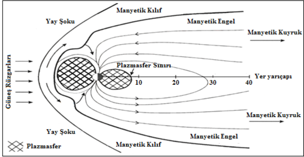
Sekil 2.2. Yer manyetosferinin şematik gösterimi [26]
