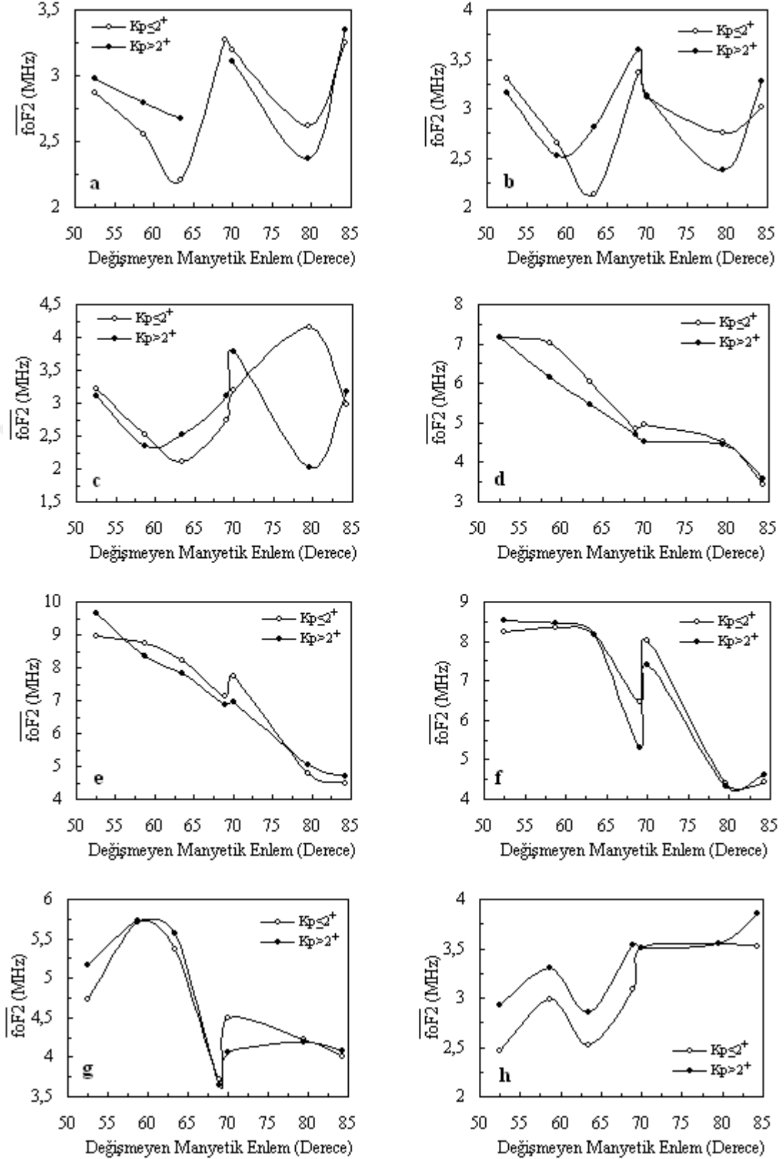
Şekil 4.10. 1971 yılı 21 Aralık döneminde K_p indisinin pasif ve aktif durumlar için farklı istasyonlardan alınan saatlik ortalama f_oF2 değerlerinin değışmeyen manyetik enlem ile değışimi: (a) YZ 00:00 için, (b) YZ 03:00 için, (c) YZ 06:00 için, (d) YZ 09:00 için, (e) YZ 12:00 için, (f) YZ 15:00 için, (g) YZ 18:00 için, (h) YZ 21:00 için
