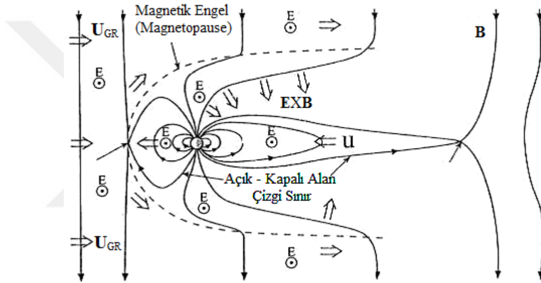
Şekil 2.10. Dünya çevresindeki elektrik ve manyetik alanları ile plazma akımları yönlerinin gösterilimi [4].
