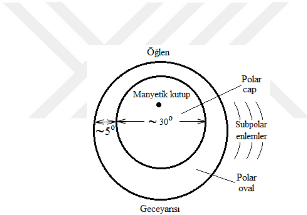
Şekil 2.9. Polar cap ve polar ovalin yapısı [5]
