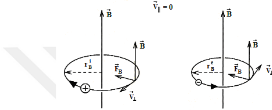
Şekil 2.4. V_{||} = 0 için düzgün bir manyetik alandaki pozitif ve negatif parçacık hareketi [5]
