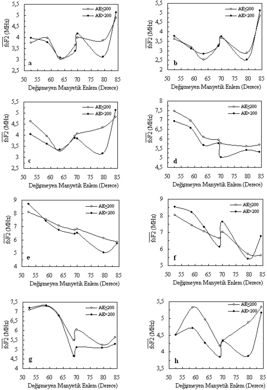
Şekil 4.8. 1972 yılı 23 Eylül döneminde AE indisinin pasif ve aktif durumlar için farklı istasyonlardan alınan saatlik ortalama f_oF_2 değerlerinin değişmeyen manyetik enlem ile değişimi: (a) YZ 00:00 için, (b) YZ 03:00 için, (c) YZ 06:00 için, (d) YZ 09:00 için, (e) YZ 12:00 için, (f) YZ 15:00 için, (g) YZ 18:00 için, (h) YZ 21:00 için
