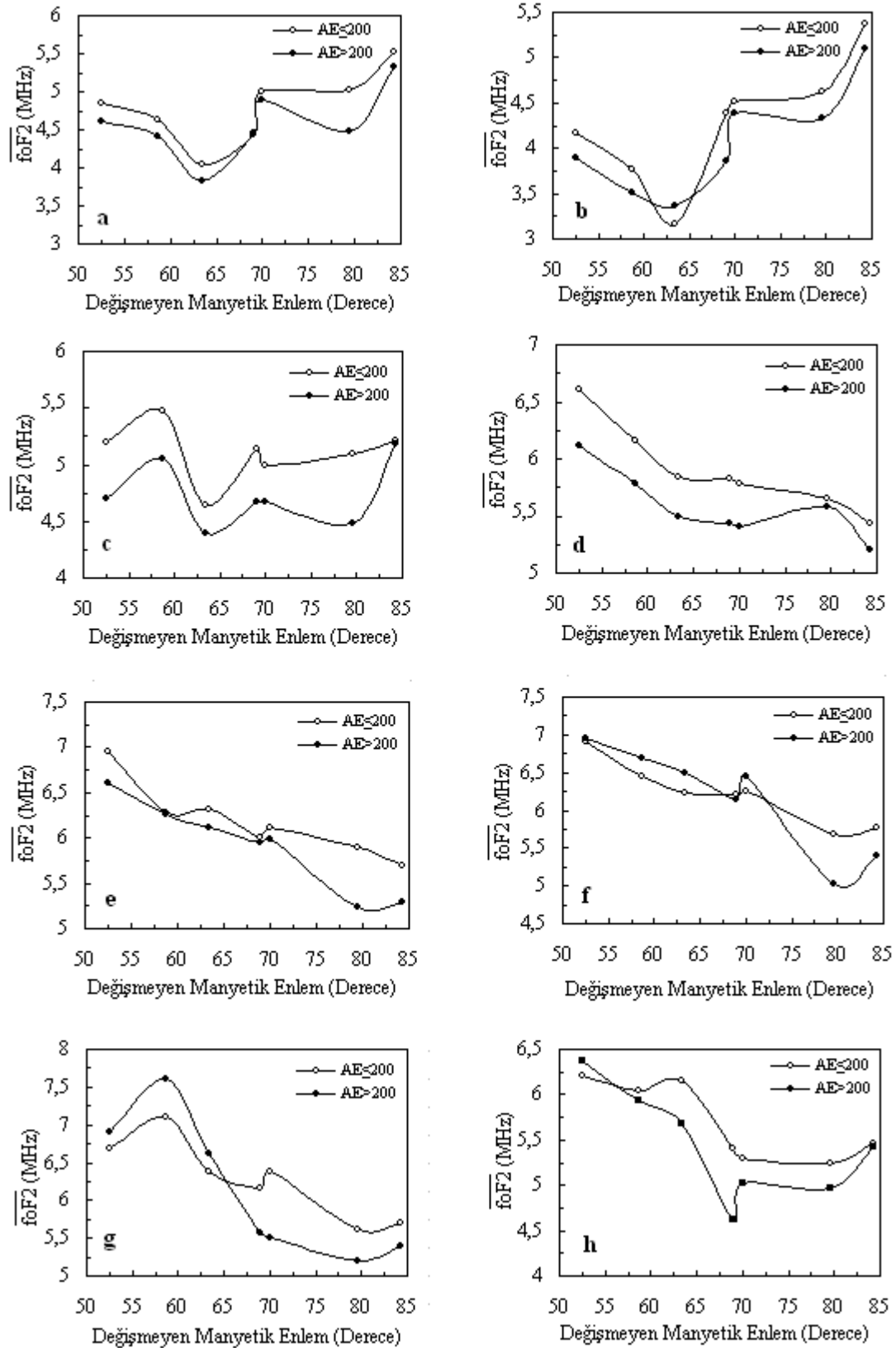
Şekil 4.5. 1972 yılı 21 Haziran döneminde AE indisinin pasif ve aktif durumlar için farklı istasyonlardan alınan saatlik ortalama f_oF_2 değerlerinin değişmeyen manyetik enlem ile değişimi: (a) YZ 00:00 için, (b) YZ 03:00 için, (c) YZ 06:00 için, (d) YZ 09:00 için, (e) YZ 12:00 için, (f) YZ 15:00 için, (g) YZ 18:00 için, (h) YZ 21:00 için
