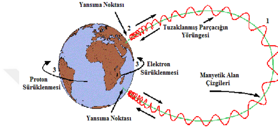
Şekil 2.3. Yüklü parçacıkların Yer'in manyetik alanındaki hareketleri [18]
