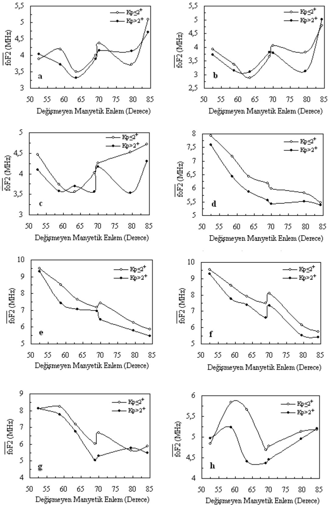
Şekil 4.1. 1972 yılı 21 Mart döneminde K_p indisinin pasif ve aktif durumlar için farklı istasyonlardan alınan saatlik ortalama f_oF_2 değerlerinin değişmeyen manyetik enlem ile değişimi: (a) YZ 00:00 için, (b) YZ 03:00 için, (c) YZ 06:00 için, (d) YZ 09:00 için, (e) YZ 12:00 için, (f) YZ 15:00 için, (g) YZ 18:00 için, (h) YZ 21:00 için
