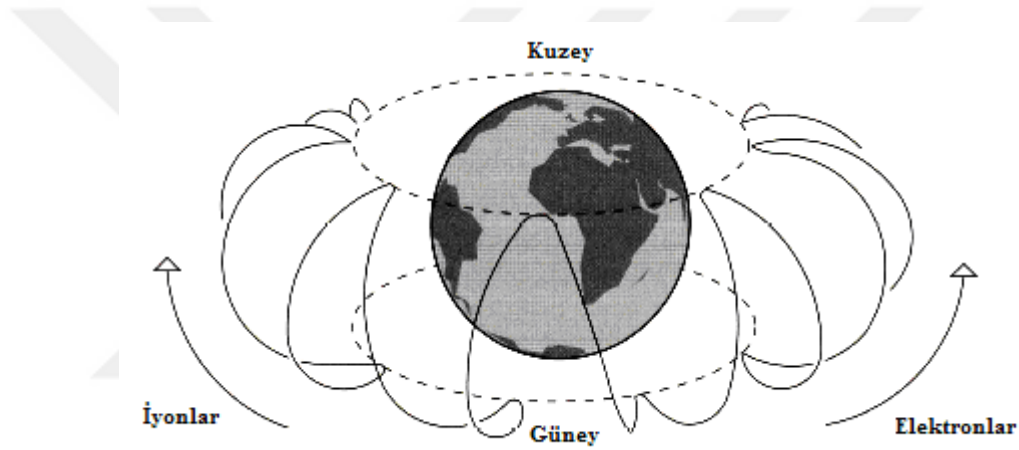
Şekil 2.8. Yüklü parçacıkların farklı yönlerdeki sürüklenme hareketi [5]
