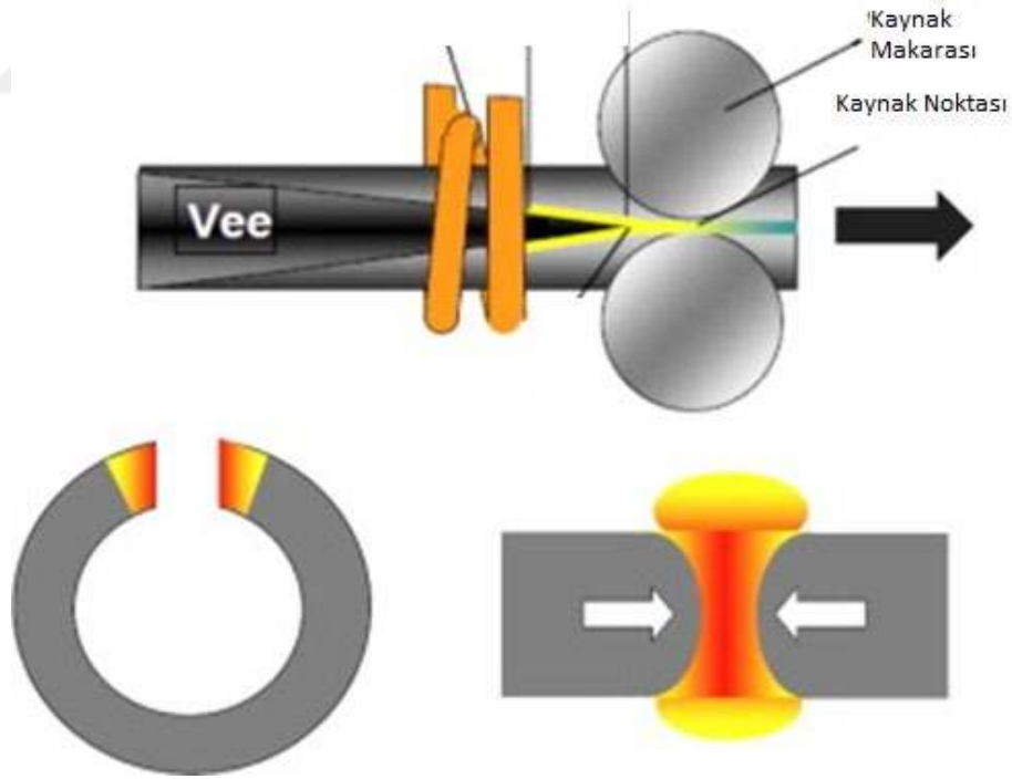
Şekil 2.12. Yüksek frekans kaynağının şematik gösterimi [28].
