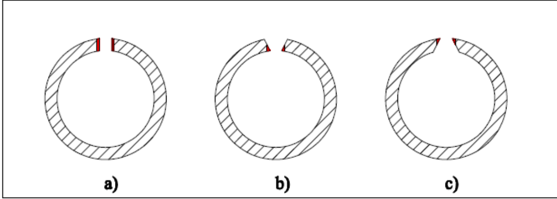
Şekil 2.16. Bandın iki ucu birleşme konumu a) paralel kenar b) içe yakın kenar c) dışa yakın kenar [6].
