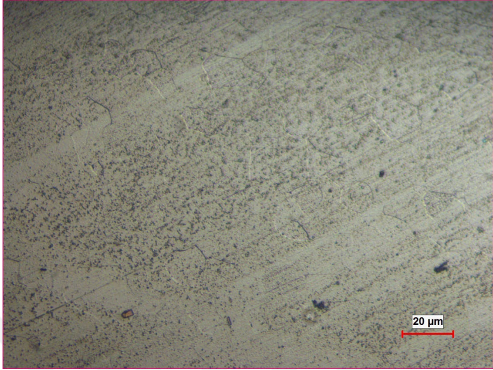
Şekil 6.74. 650°C tavlama sonrası 7114 tip numune ana metal mikroyapı görüntüsü.
