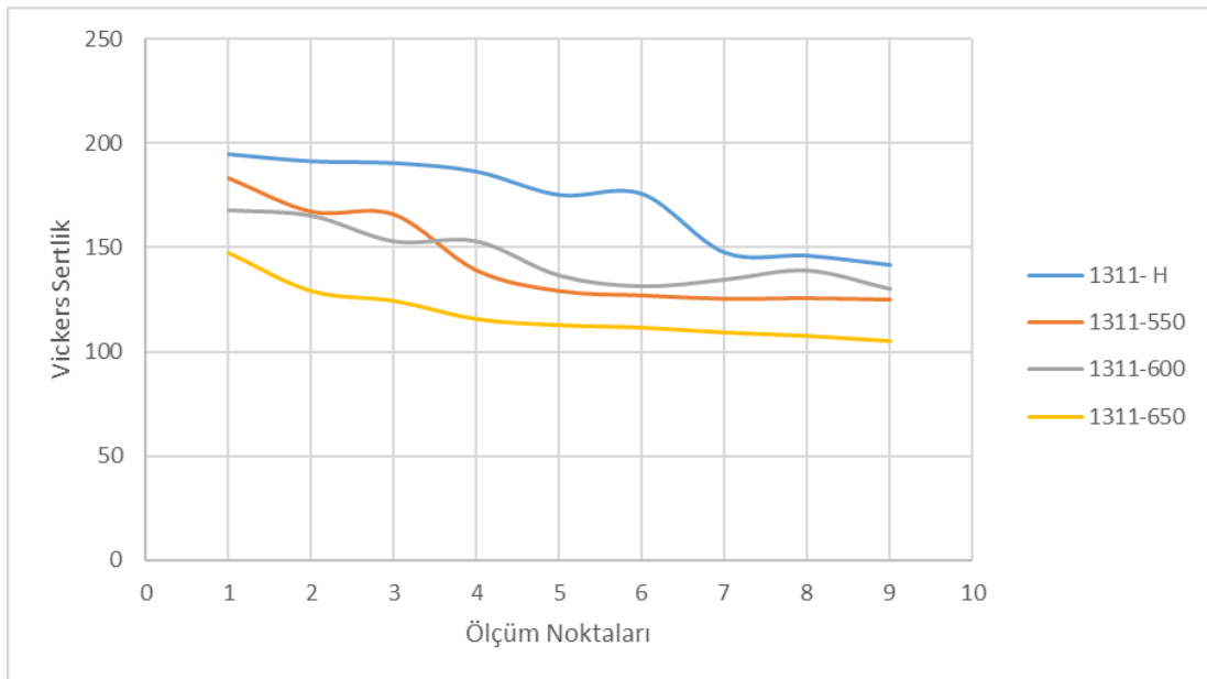
Şekil 6.6. 1311 tipi çelik mikrosertlik sonuçları.
