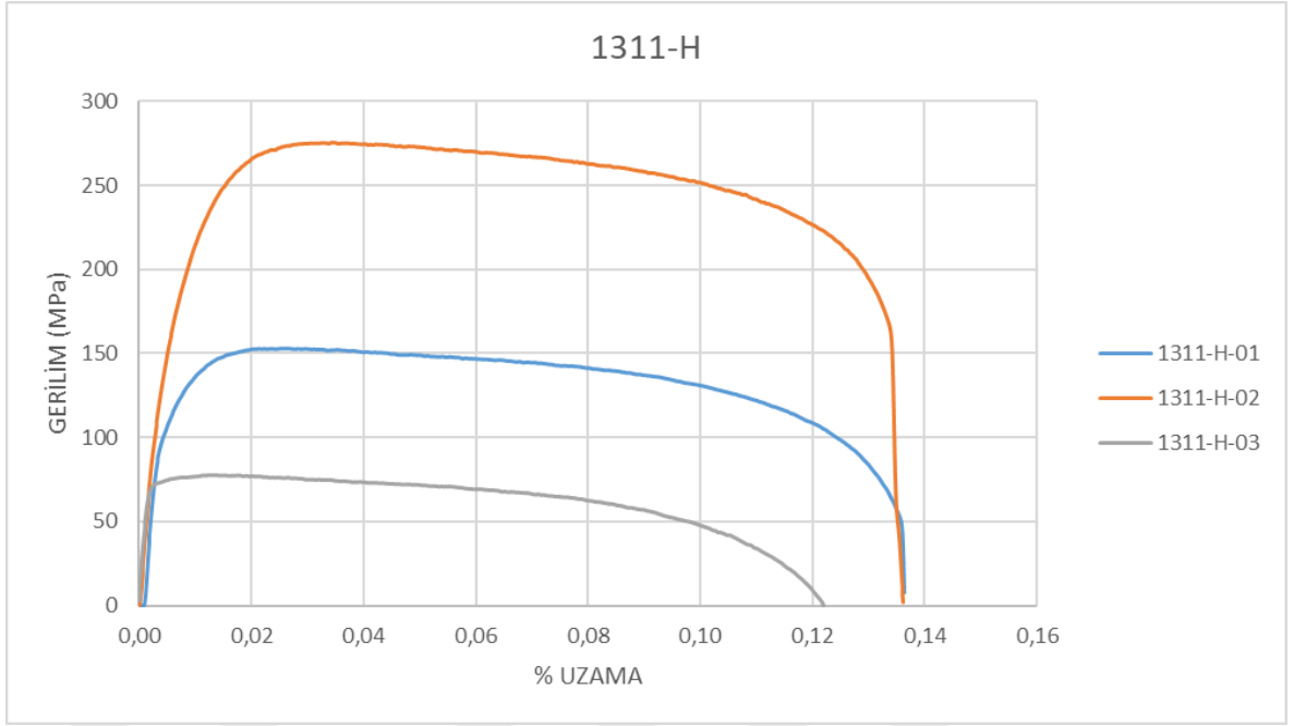
Şekil 6.12. 1311 tipi çeliklerin üretim sonrası çekme testi sonuçları.
