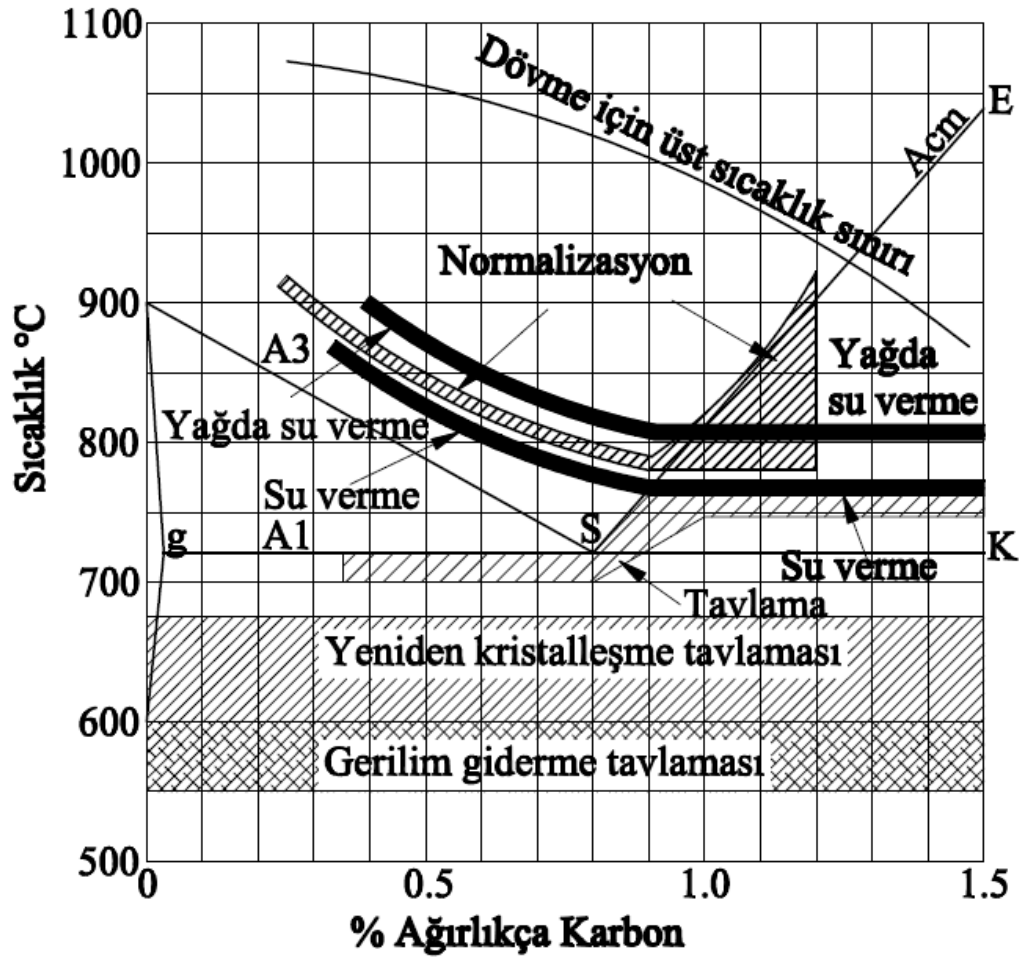
Şekil 4.1. Çeliklere uygulanan ısıtıl işlem alanlarının demir karbon denge diyagramı üzerinde gösterilişi [50].
