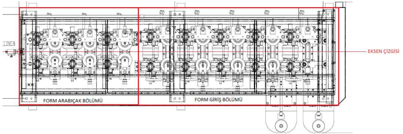
Şekil 2.7. Form ünitesi üst görünüş ve bölümleri [4].
