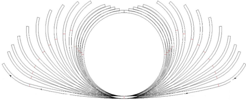
Şekil 2.6. Boru üretim aşamasında çiçek deseninin oluşumu [16].
