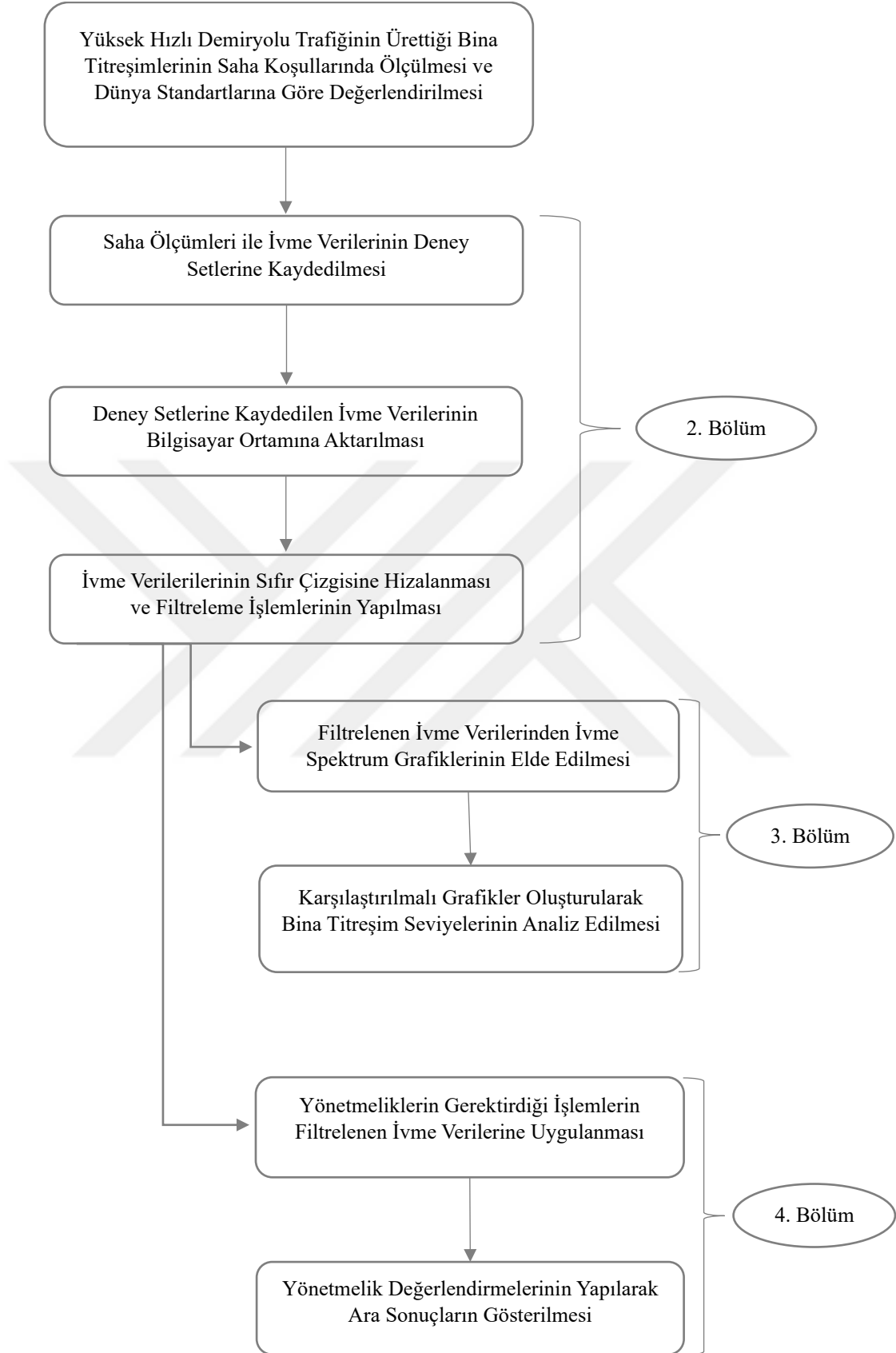
Şekil 2.1. YHT titreşim değerlendirmeleri işlem adımları
