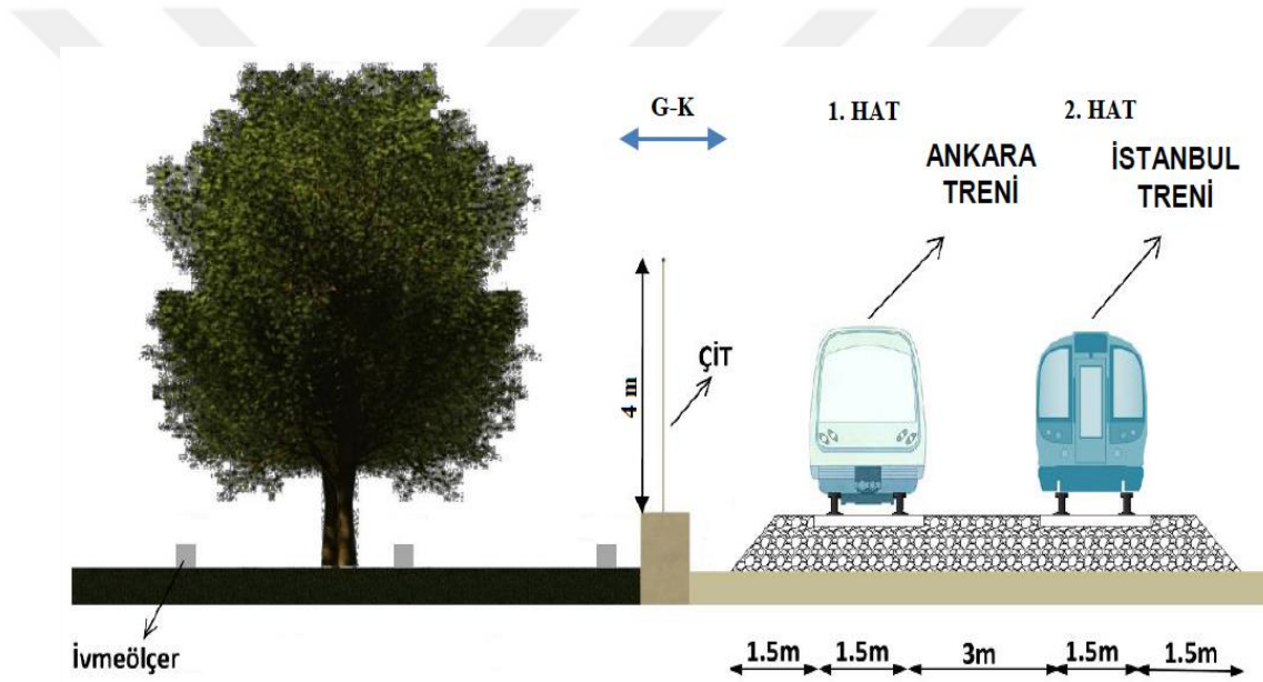
Şekil 2.10. Gebze/GTÜ Kampüs test sahasının yandan görünümü
