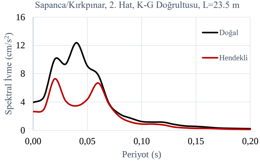
Şekil 3.19. Sapanca/Kırkpınar mevkinde 2. hat (İstanbul) geçişi için L=23.5 m K-G doğrultusunda doğal ve hendekli zemin ivme tepki spektrumlarının karşılaştırılması
