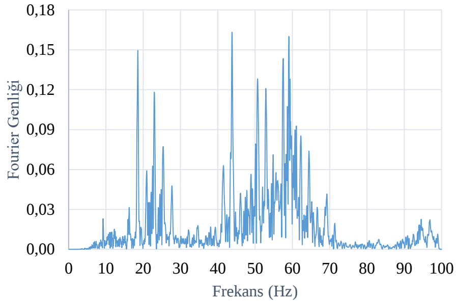
(b) D-B Doğrultusu
