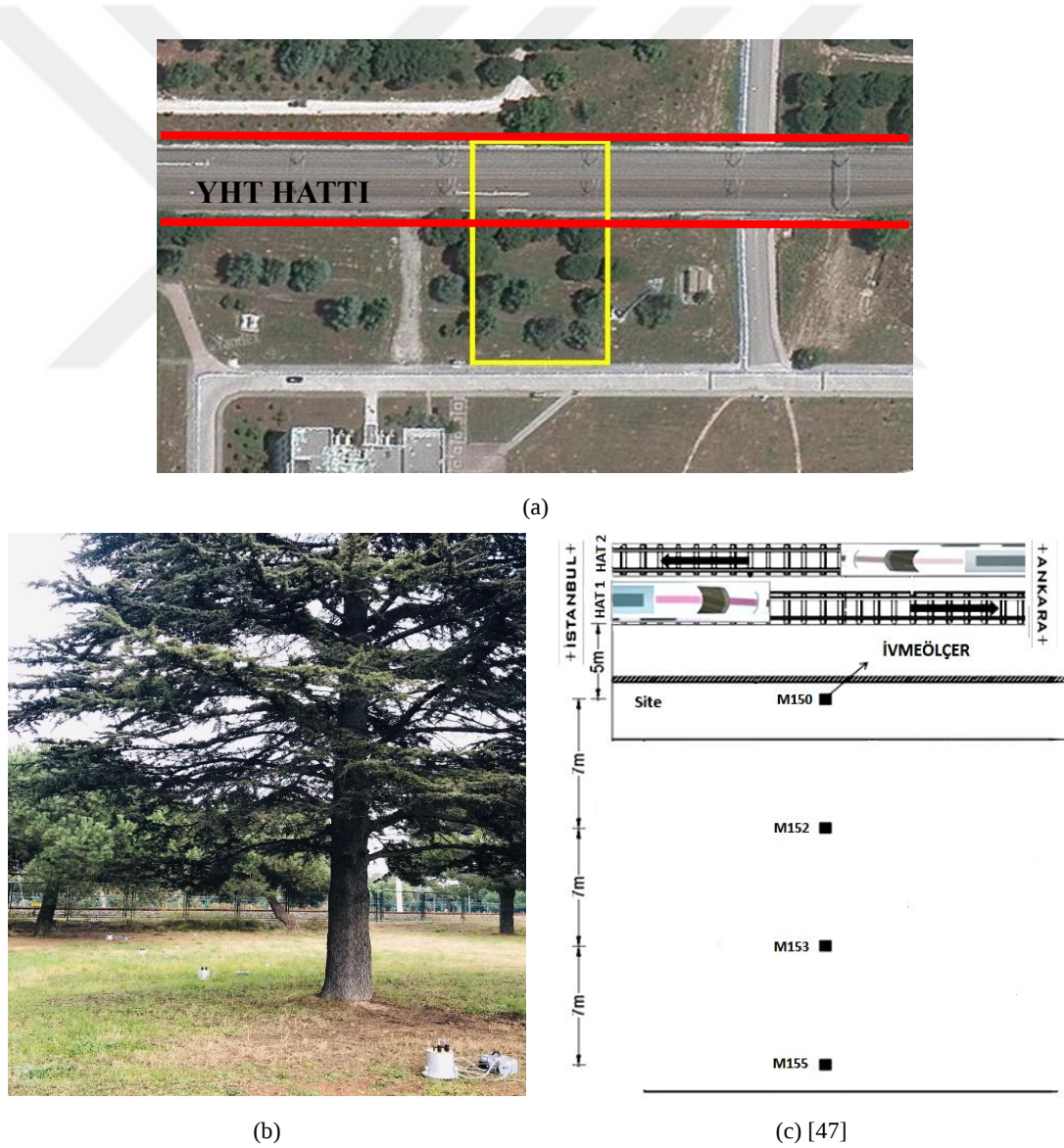
Şekil 2.9. Gebze/GTÜ Kampüs test alanı uydü (a) ve saha görüntüsü (b), ivmeölçer yerleşim planı (c)
