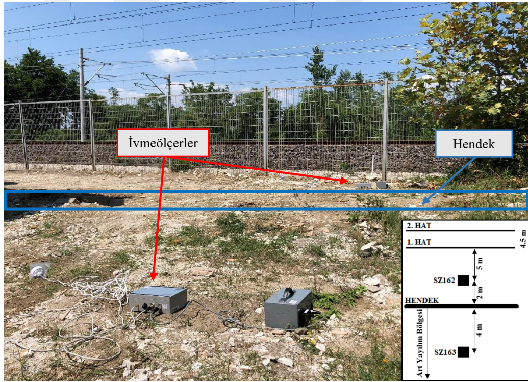
Şekil 3.11. Sapanca/Kırkpınar test sahasında bulunan hendeğin konumu
