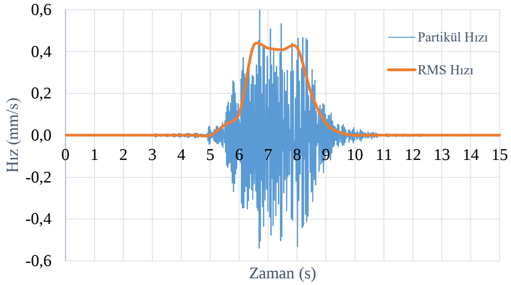
(b) D-B Doğrultusu Şekil 4.5 (Devamı)
