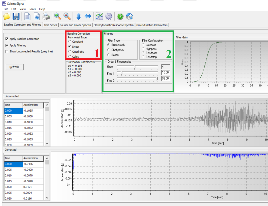
Şekil 2.15. İvme verisinin sıfır çizgisine hizalanması ve filtrelenmesi
