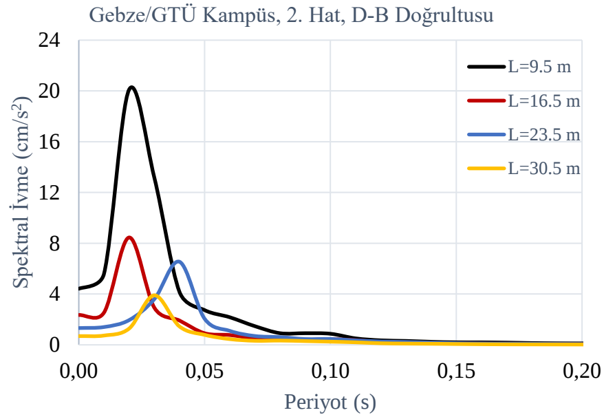
Şekil 3.33. Gebze/GTÜ Kampüs mevkinde 2. hat (İstanbul) geçişi için D-B doğrultusunda ivme tepki spektrumlarının karşılaştırılması
