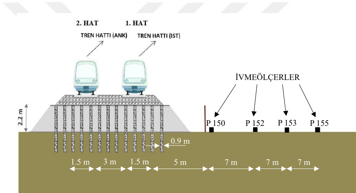
Şekil 2.12. Pamukova/Yenice test sahasının yandan görünümü
