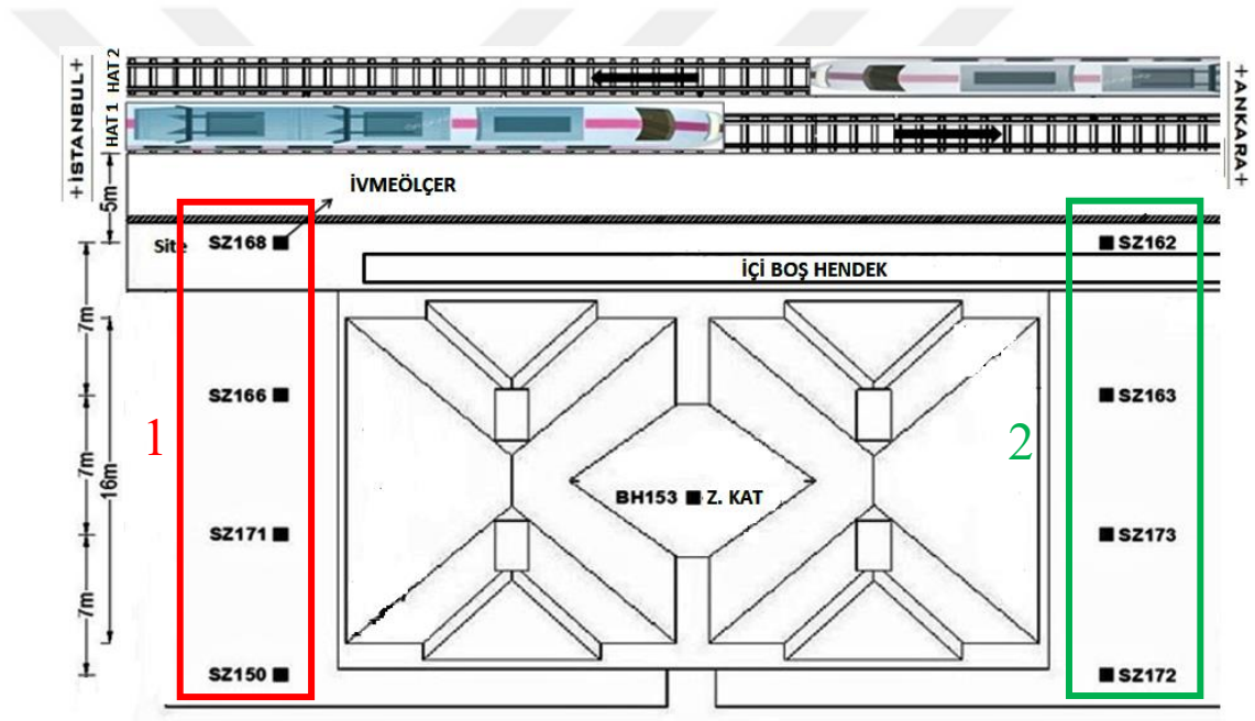
Şekil 2.6. Sapanca/Kırkpınar test alanı ivmeölçer yerleşim planı [47]
