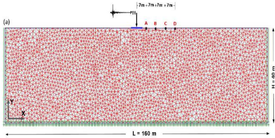
Şekil 1.11. Sahadaki ivmeölçerlerin oluşturulan modelde temsil edildiği noktalar [48]
