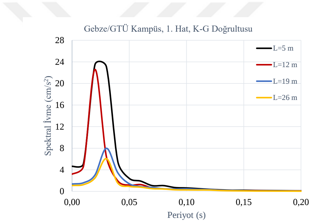
Şekil 3.30. Gebze/GTÜ Kampüs mevkinde 1. hat (Ankara) geçişi için K-G doğrultusunda ivme tepki spektrumlarının karşılaştırılması
