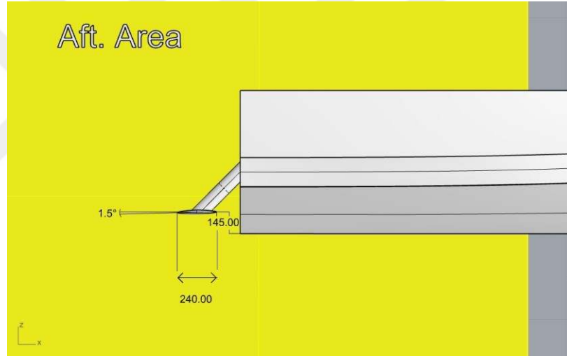
 ekil 2.20. Optimize edilmi  k   b lgesindeki kanadın kord uzunlu u, h cum a ısı ve derinli inin g sterimi
