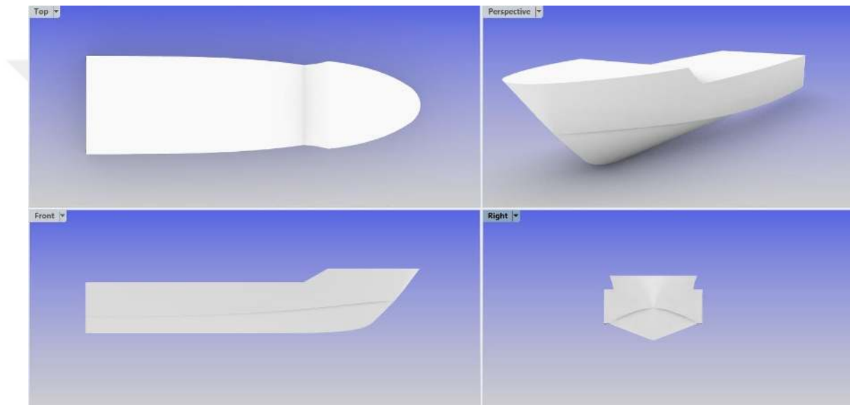
Şekil 2.8. Form-A tipi kayıcı teknenin görünüşü
