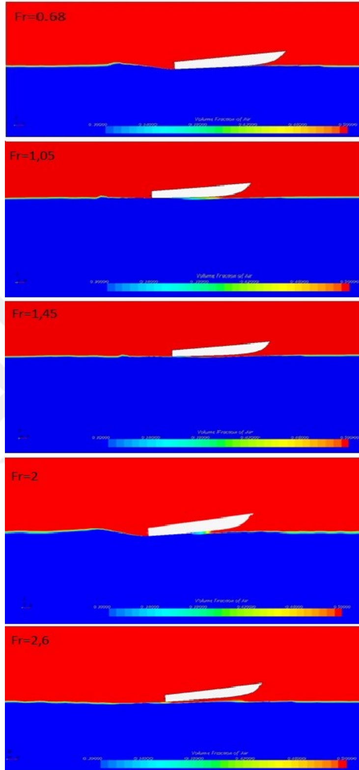
Şekil 2.33. Gövde kış kanat eklenmiş Form B'deki hacim fraksiyonu skaler ekran görüntüleri
