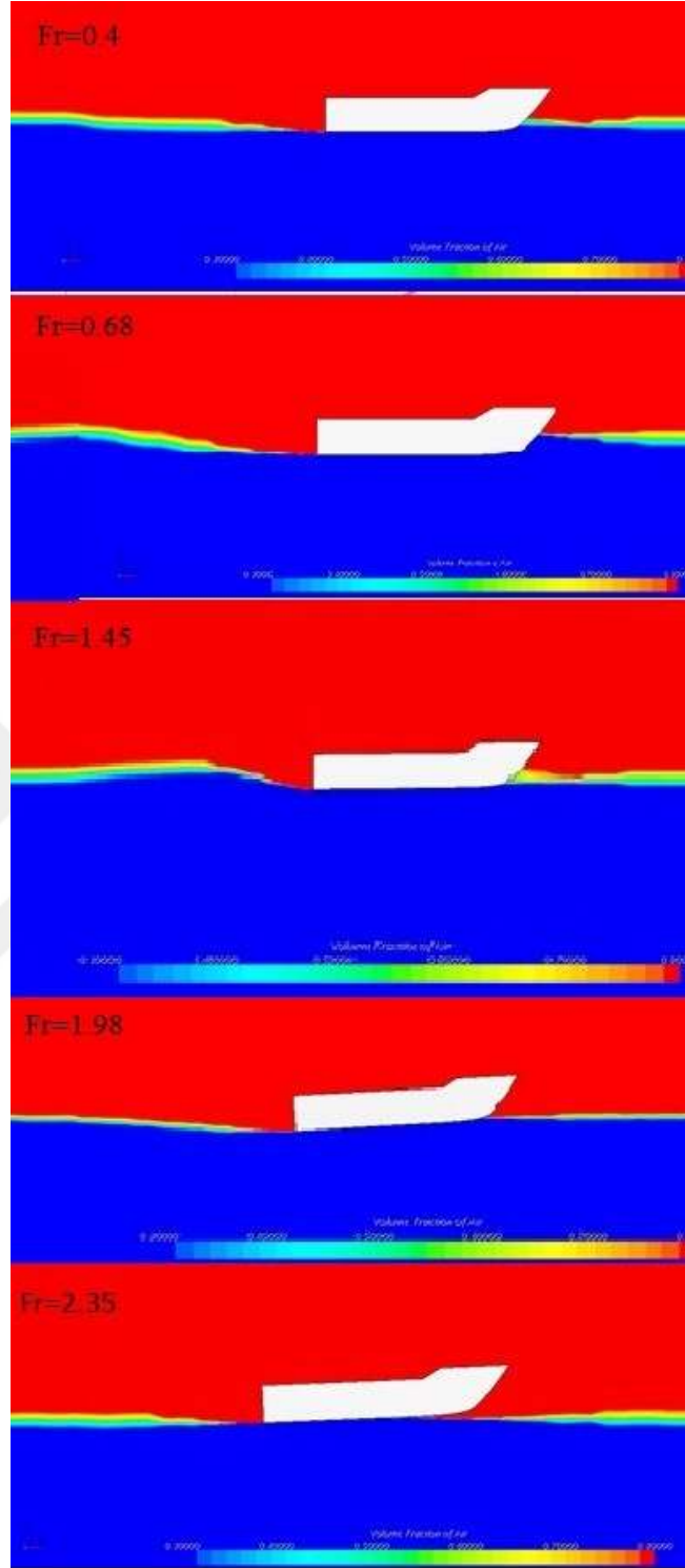
Şekil 2.13. Form A tipi kayıcı tip tekne için Froude hızlarındaki hacim fraksiyonu skaler ekran görüntüleri
