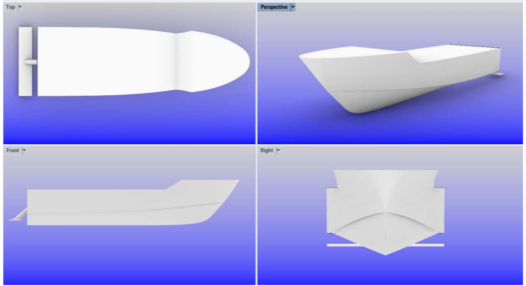
Şekil 2.15. Gövde kıç kanadı eklenmiş 3 boyutlu Form A modelinin görüşleri
