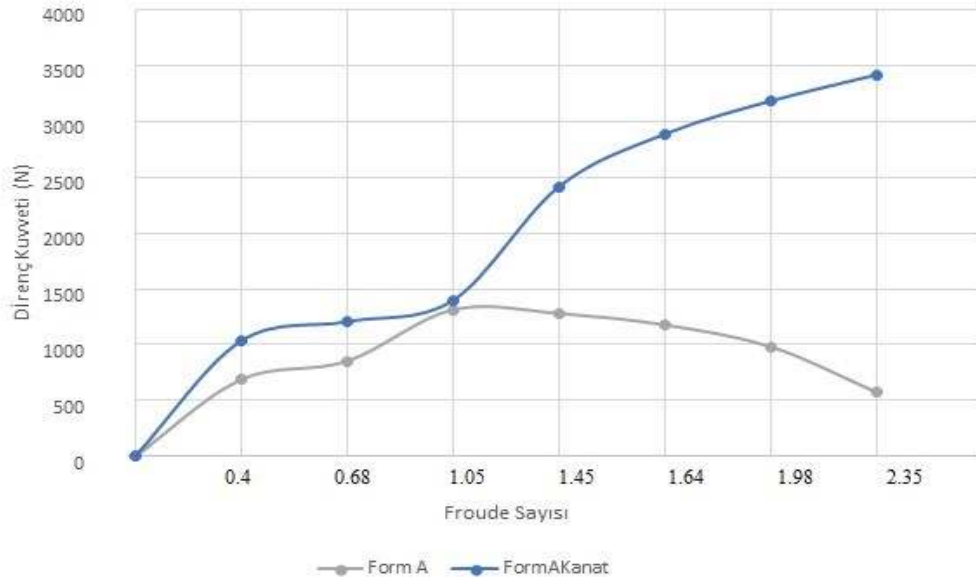
řekil 2.19. Form A tipi sadece tekne ve tekne ile kanat eklenmiř halinin Froude hızlarına göre direnç değıřimi grafiğı
