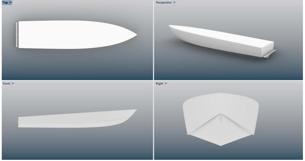
Şekil 2.32. Gövde kış kanadı eklenmiş üç boyutlu Form B modelinin görünüşleri
