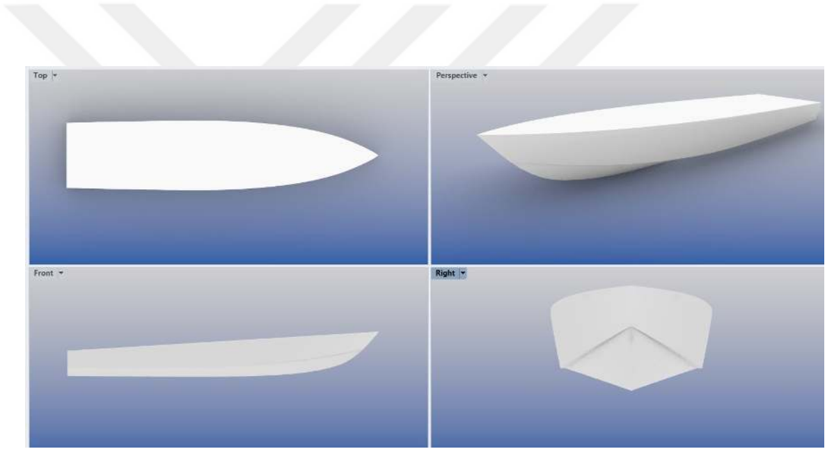
Şekil 2.24. Form-B tipi kayıcı teknenin görünüşü
