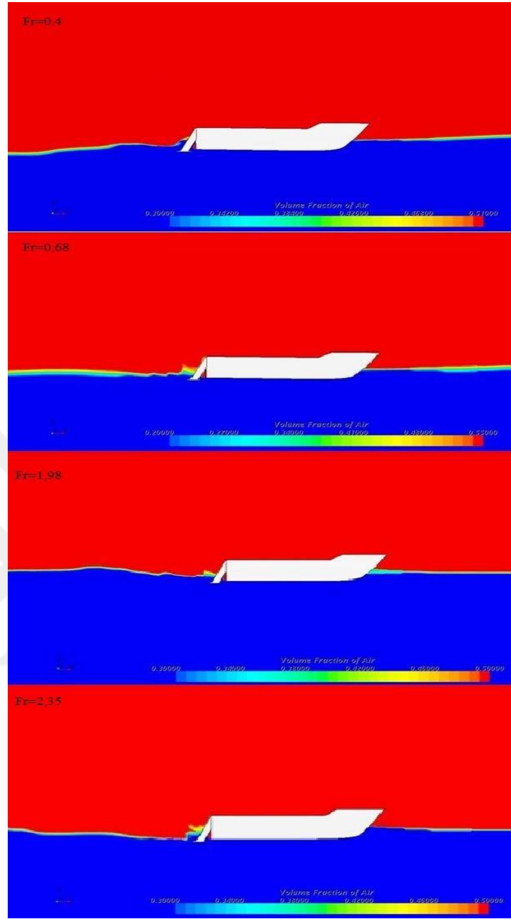
Şekil 2.17. Gövde kıç kanat eklenmiş Form A'daki hacim fraksiyonu skaler ekranları
