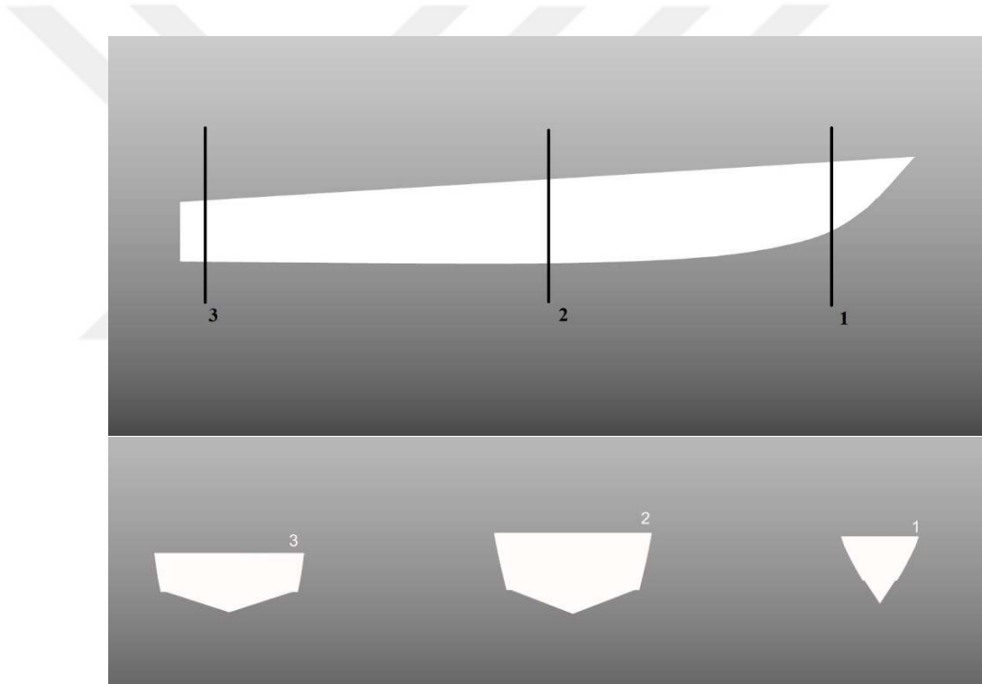
ekil 2.23. Form-B tipi kayıcı teknenin  farklı dzlemdeki kesitlere gre llen kalkıntı aılarının gsterimi ( \beta_3 = 17.9^\circ , \beta_2 = 21.1^\circ , \beta_1 = 56.6^\circ )
