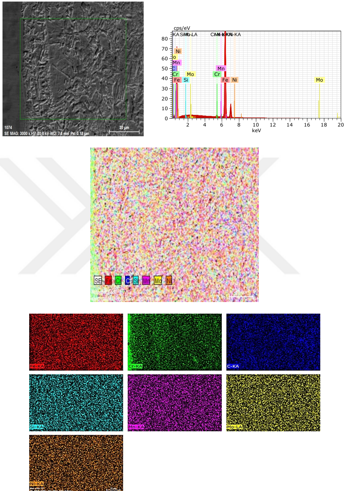
Şekil 4.29 S1 numunesinin YKBDD tarafı elementel haritalandırma analiz sonuçları
