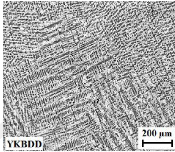
Şekil 4.6 YKBDD'nin mikroyapı fotoğrafı
