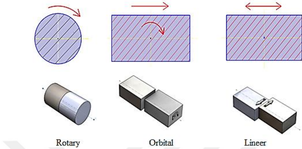
Şekil 1.2 Sürtünme kaynağı için ara yüzey üzerinden ısı üretimi karşılaştırması siyah oklarla gösterilmiştir
