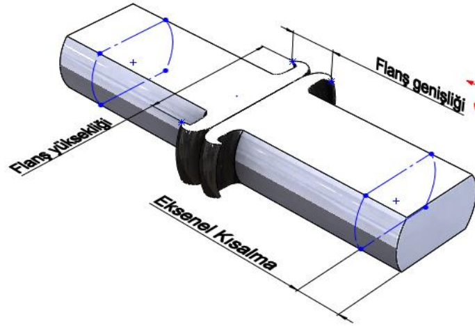
Şekil 4.4 Deney numunelerinin flanş geometrisi ve boyca kısılma miktarına ait özellikler
