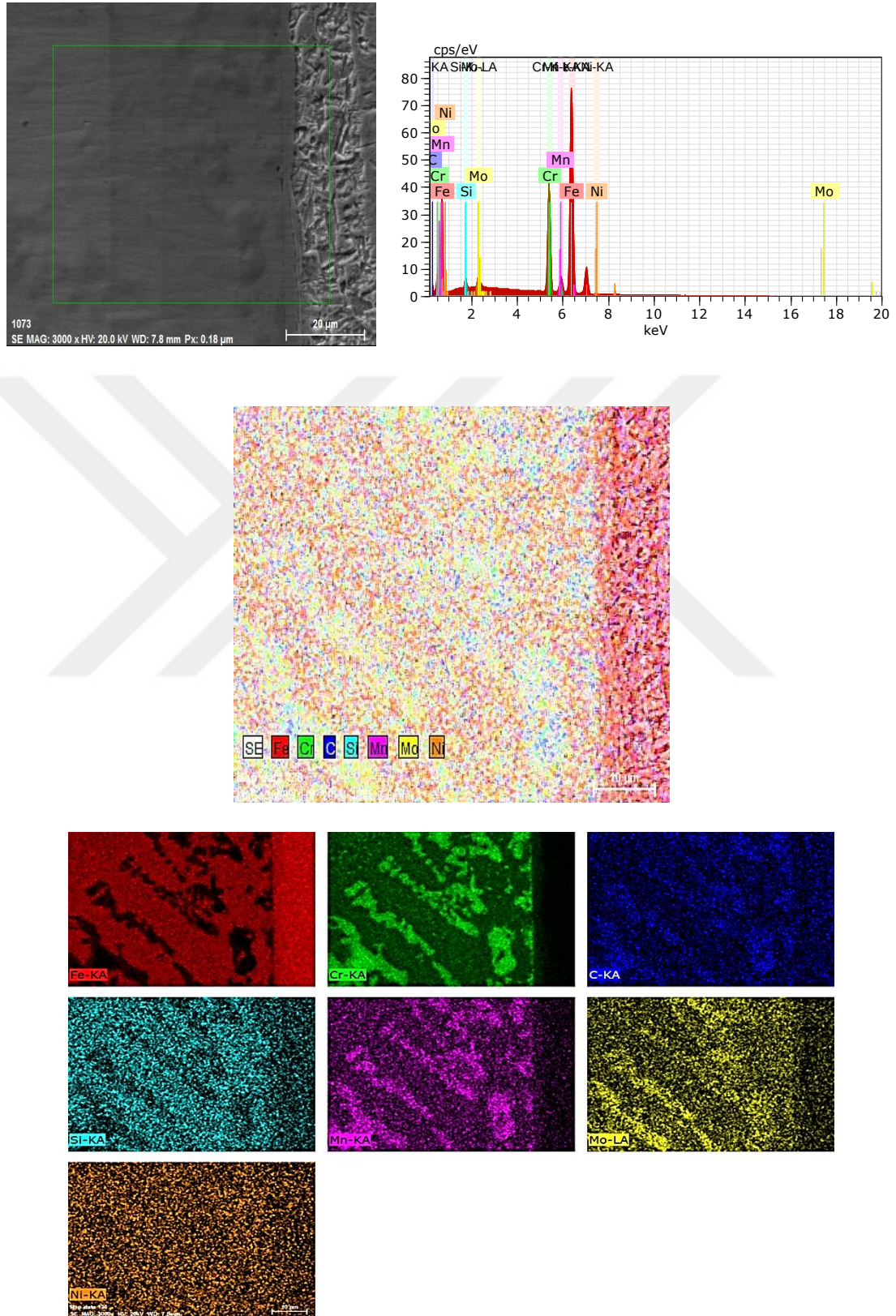
Şekil 4.28 S1 numunesinin AISI1040 tarafı elementel haritalandırma analiz sonuçları
