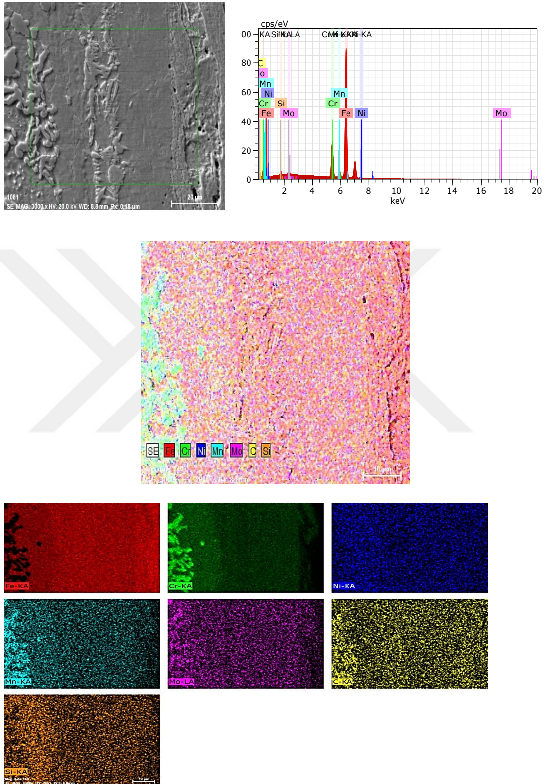
Şekil 4.31 S5 numunesinin AISI1040 tarafı elementel haritalandırma analiz sonuçları
