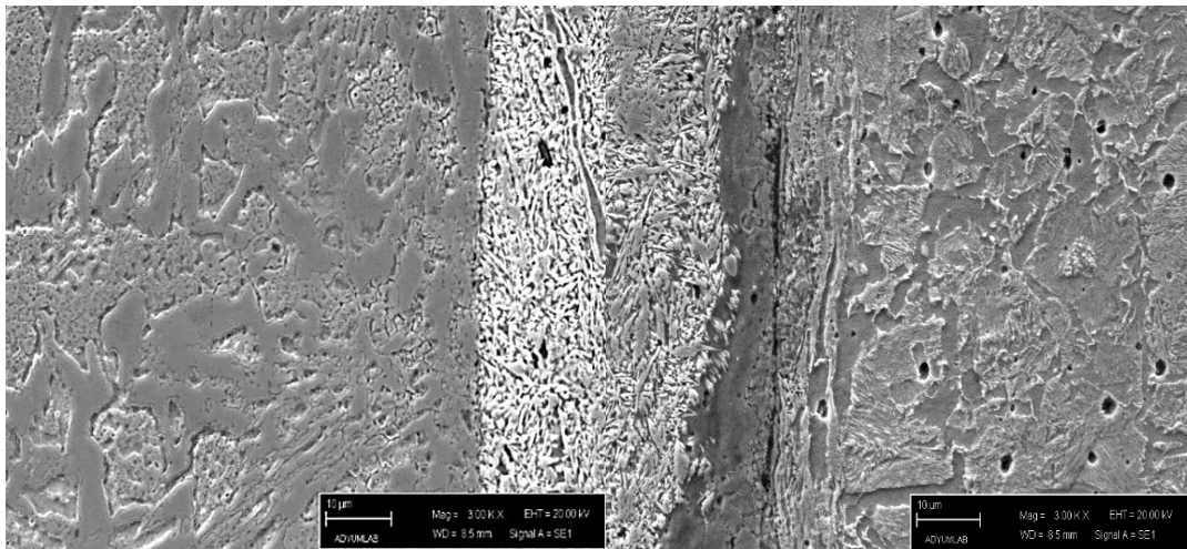
Şekil 4.14 S3 no'lu numunenin genel SEM görüntüsü
