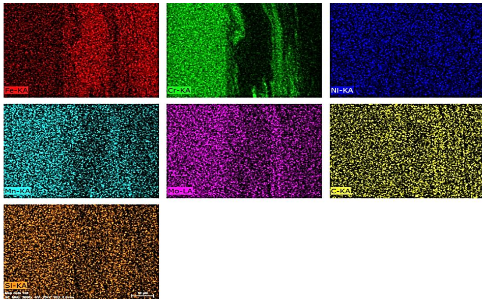
Şekil 4.30 S5 numunesinin kaynak metali elementel haritalandırma analiz sonuçları
