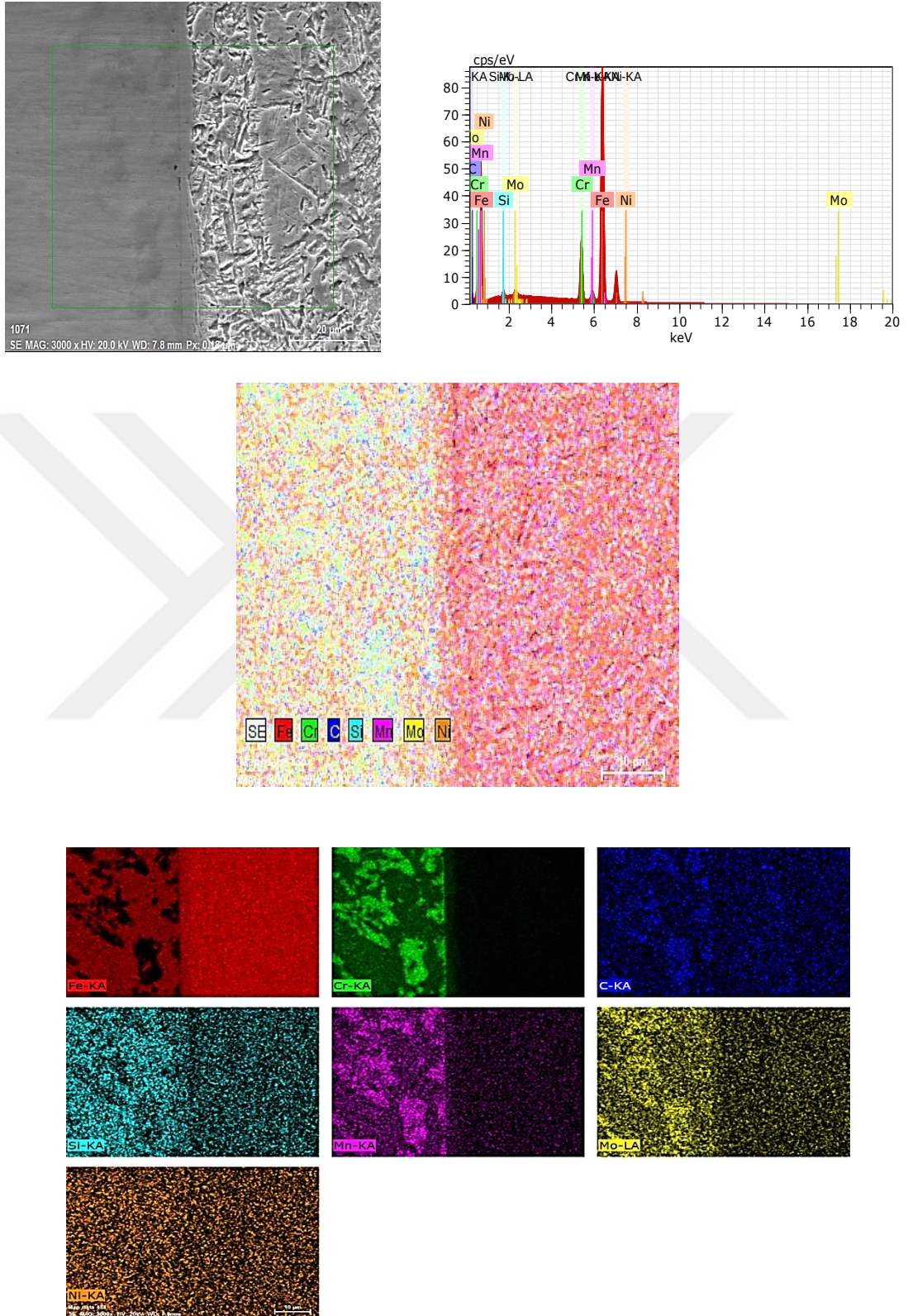
Şekil 4.27 S1 numunesinin kaynak metali elementel haritalandırma analiz sonuçları
