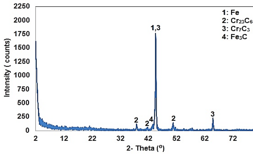
Şekil 4.24 S3 Numunesinin X-Işını analiz grafiği
