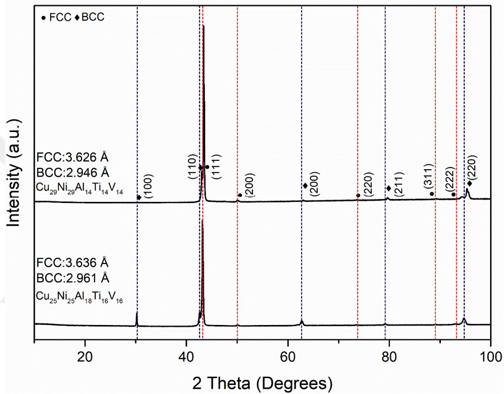
Figure 6.1. XRD pattern of 3 mm Cu 25 Ni 25 Al 18 Ti 16 V 16 , and Cu 29 Ni 29 Al 14 Ti 14 V 14 LWHEA rods
