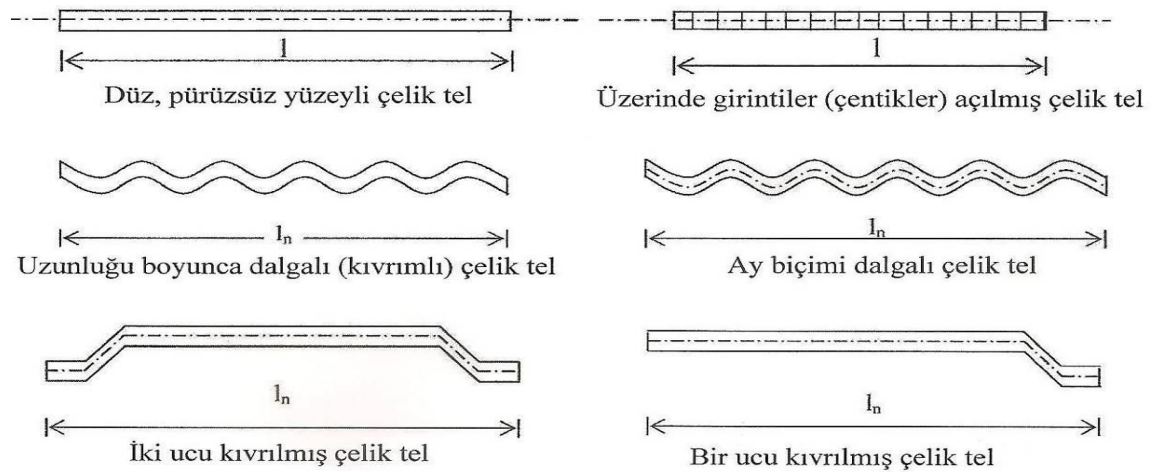
Şekil 2.3. Çelik liflere ait şekiller (TS 14889-1, 2006)
