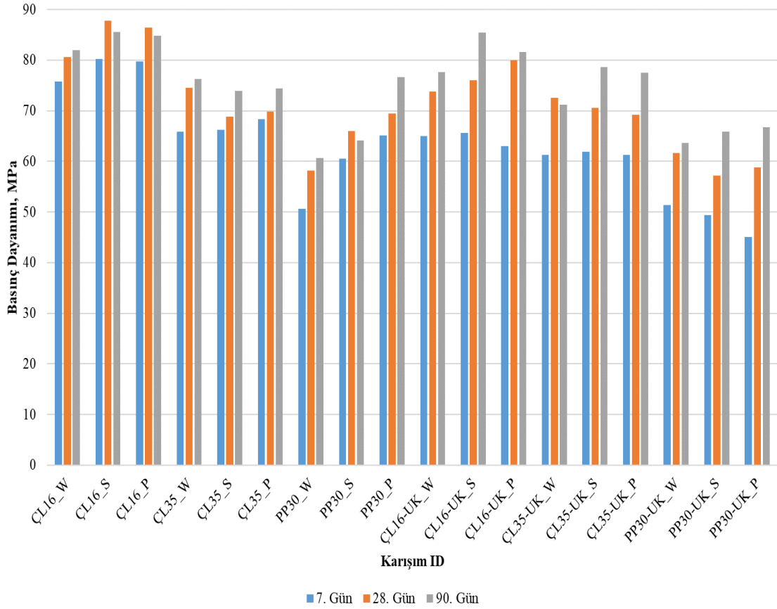
Şekil 4.1. Kür yaşına göre karişım basınç dayanımı değerleri
