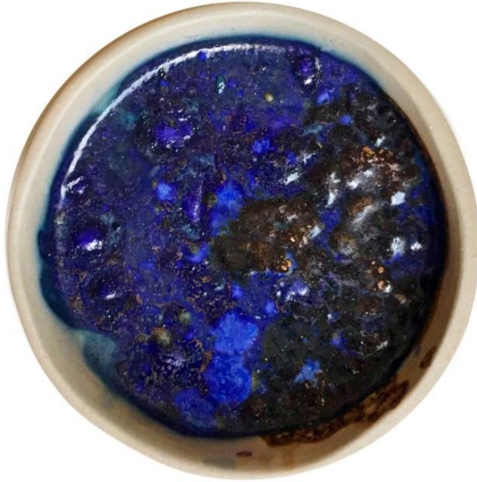
Görsel 5.17. Uygulama 9, %60 Sarımsak Külü - %40 Saydam Frit + %1 CoO, 9 x 9 x 2cm, 1200°C, 2020 (Ereshova, 2020)
