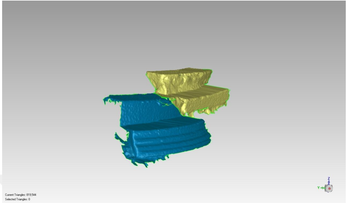
Şekil 8.17. Ağ model
