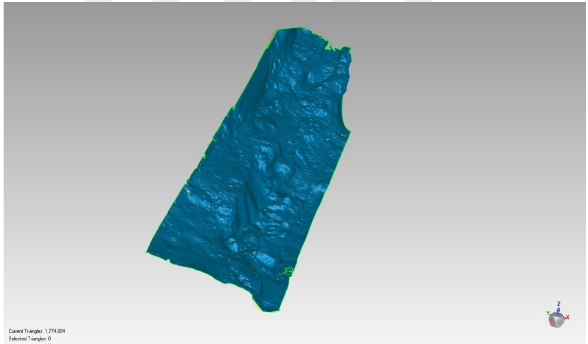
Şekil 8.8. Ağ model
