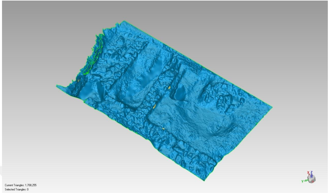
Şekil 8.3. Ağ model
