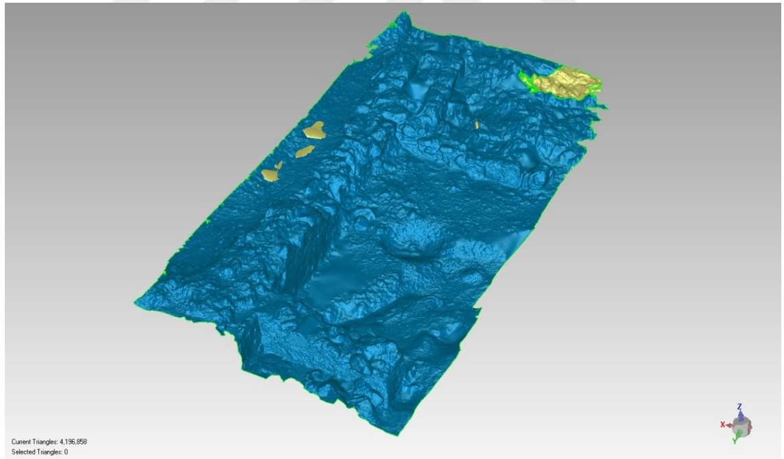
Şekil 8.12. Ağ model
