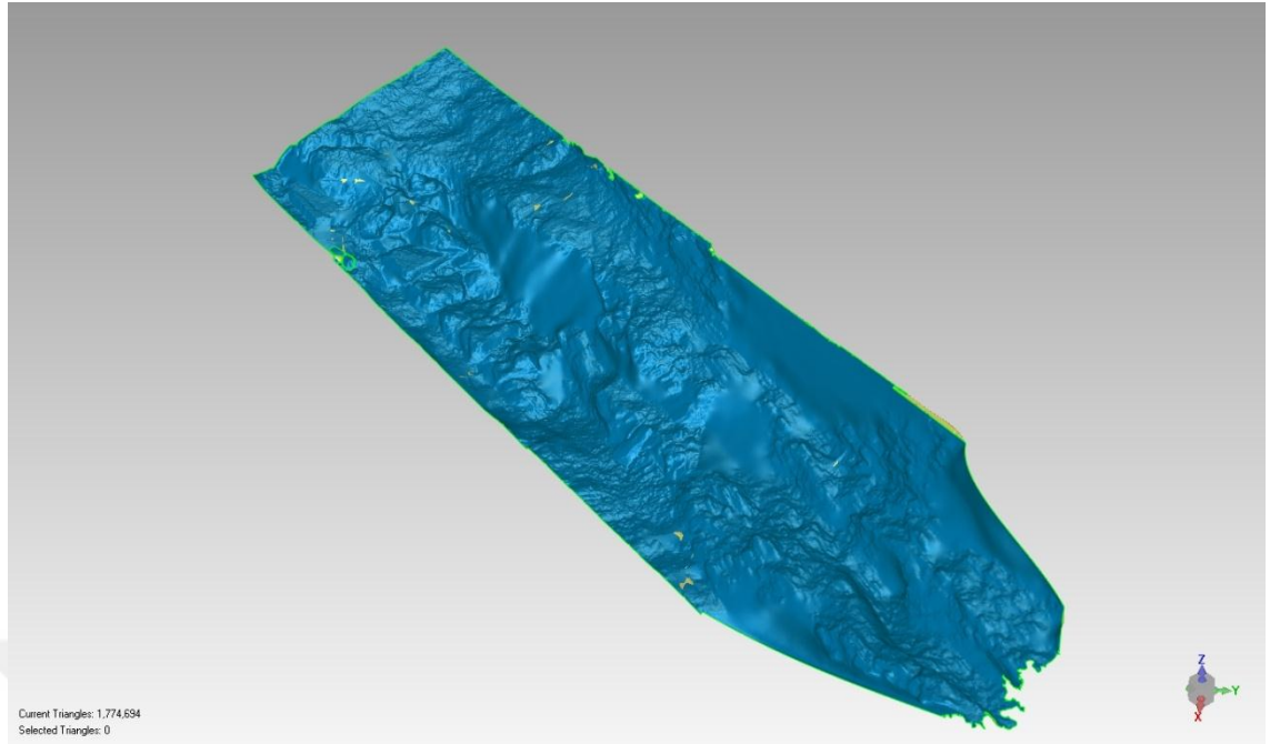
Şekil 8.7. Ağ model
