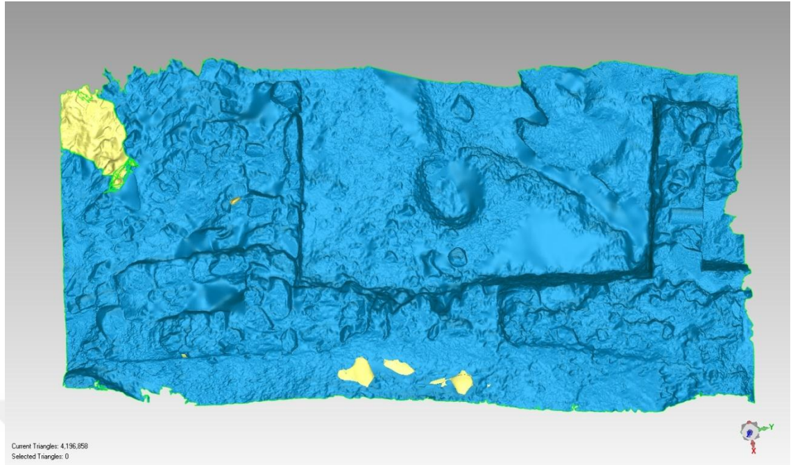
Şekil 8.9. Ağ model
