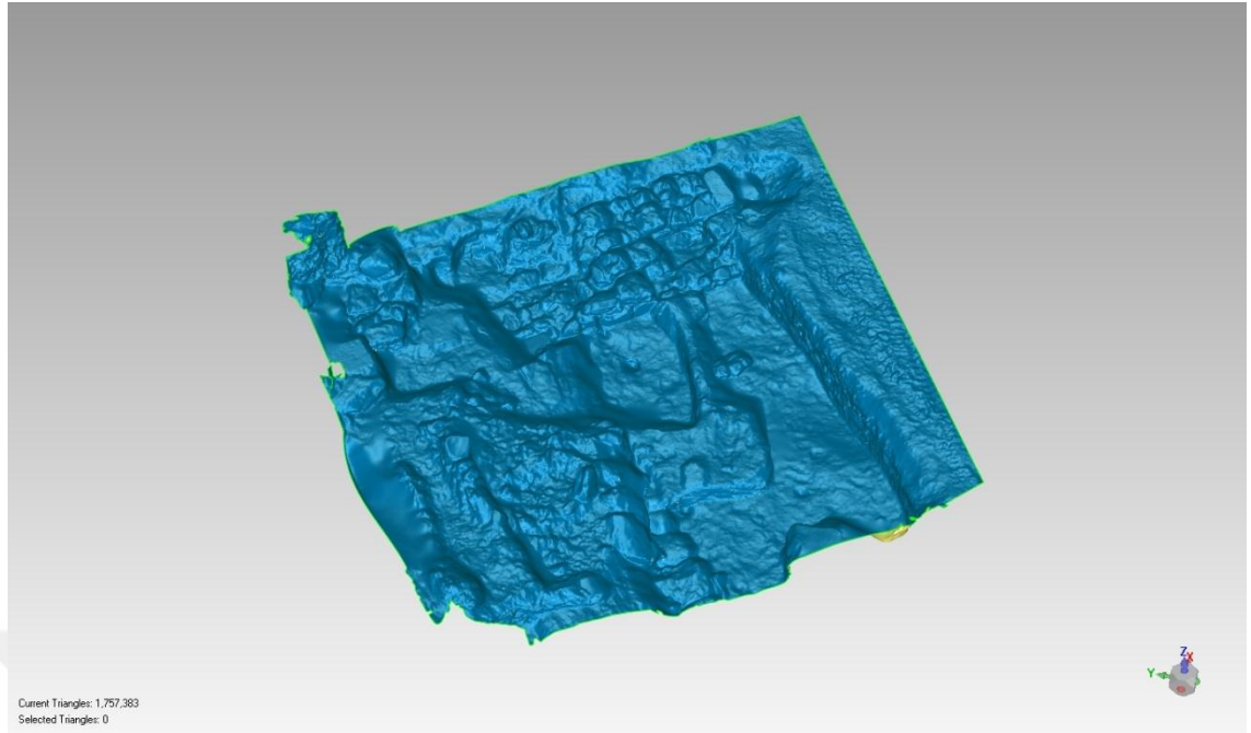
Şekil 8.19. Ağ model
