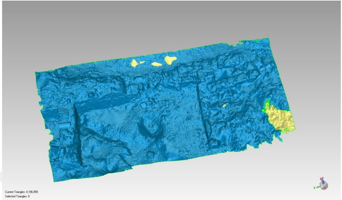
Şekil 8.11. Ağ model
