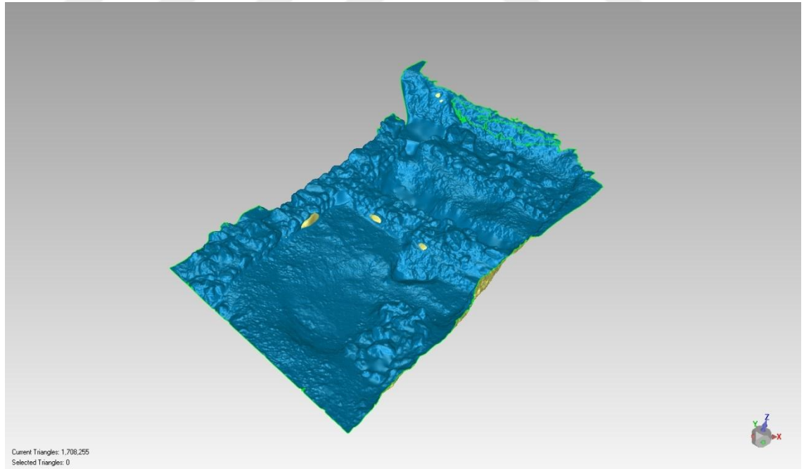
Şekil 8.2. Ağ model
