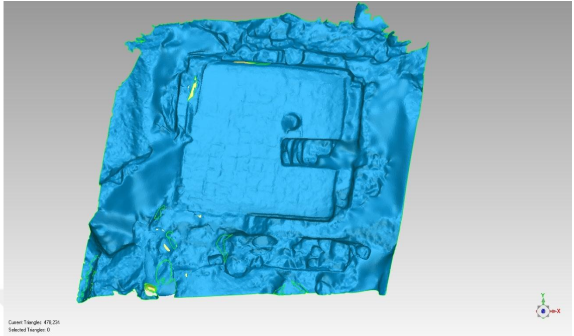
Şekil 8.13. Ağ model
