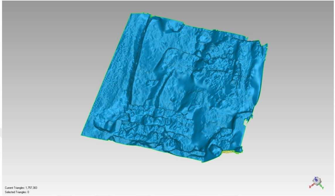
Şekil 8.1. Ağ model
