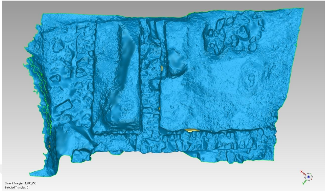
Şekil 8.5. Ağ model
