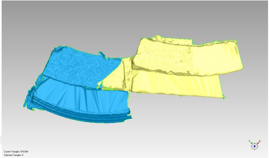
Şekil 8.15. Ağ model
