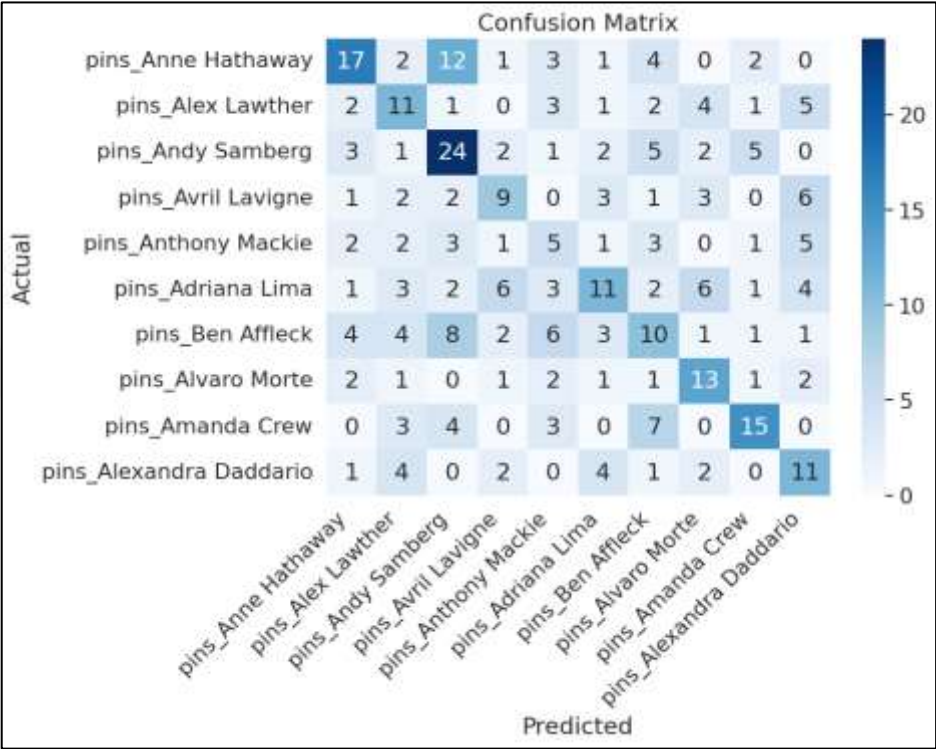
Figure 4.28: CM od DT.
