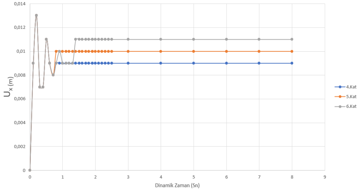
Şekil 3. 11. 4-5-6. kat deformasyonu
