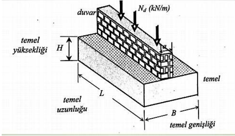
Şekil 1. 2. Duvar altı temel
