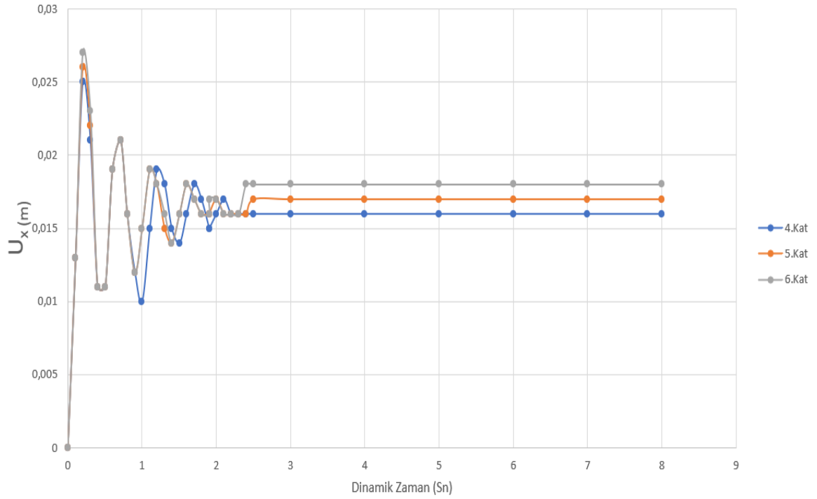
Şekil 3. 3. 4-5-6. katlar deformasyonları
