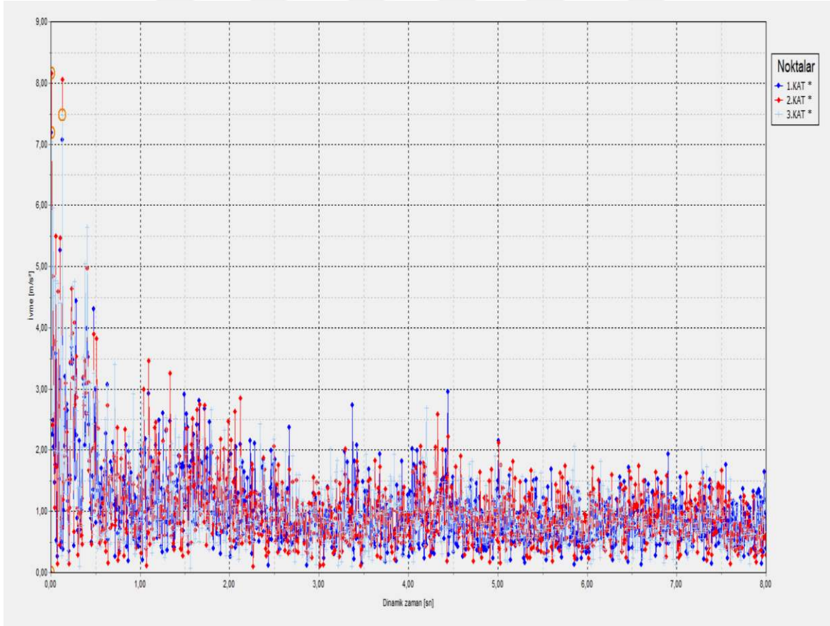
Şekil 3. 5. 1-2-3. katlar ivmesi
