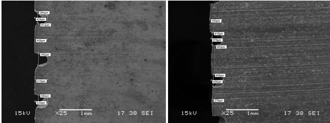
Şekil 4.8. Cu [407] [1]ve Al [407] [1] SEM ölçüm görseli
