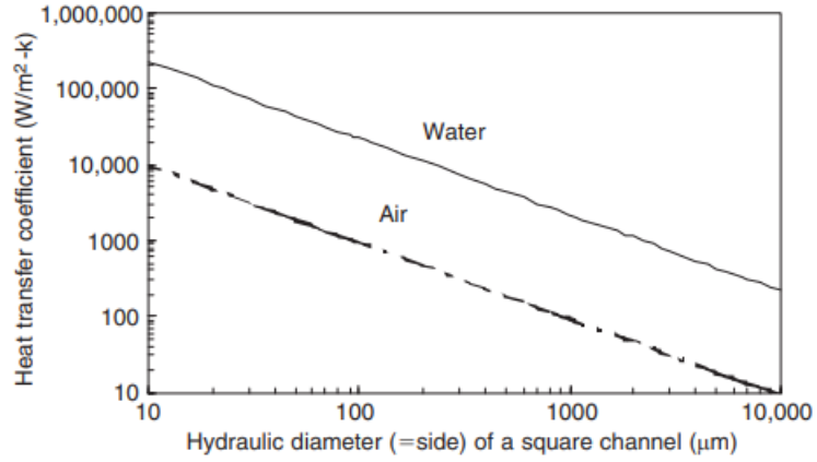
Şekil 3.2. Tam gelişmiş laminar hava ve su akışı için ısı transfer katsayısının kanal boyutu ile değişimi, Kandlikar (2005).
