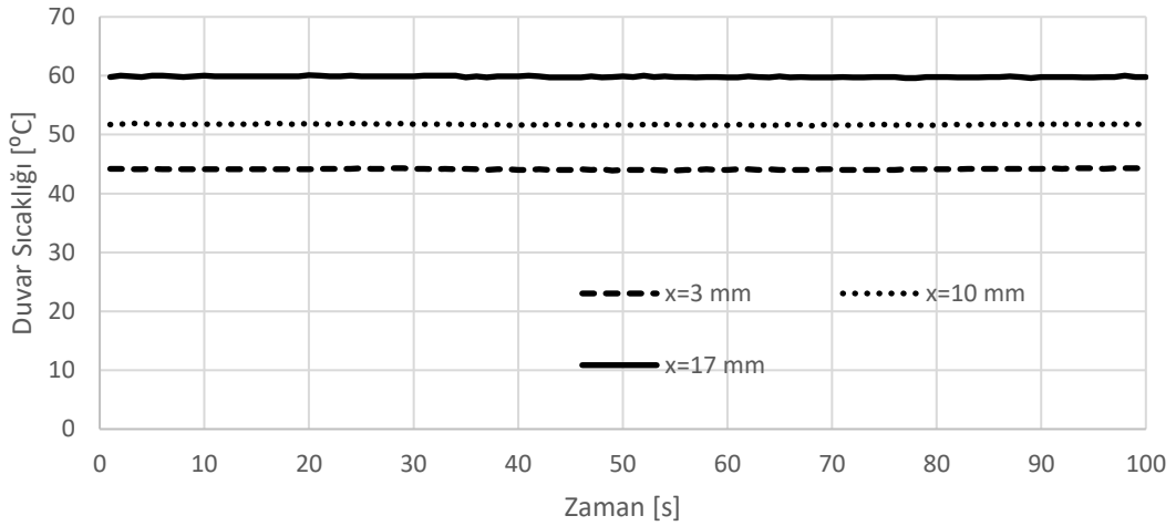
Şekil 5.1. G=412 \text{ kg/m}^2\text{s} için x=3, 10 ve 17 \text{ mm} 'de eksenel yönde Cu[502][0,4] duvar sıcaklıkları.
