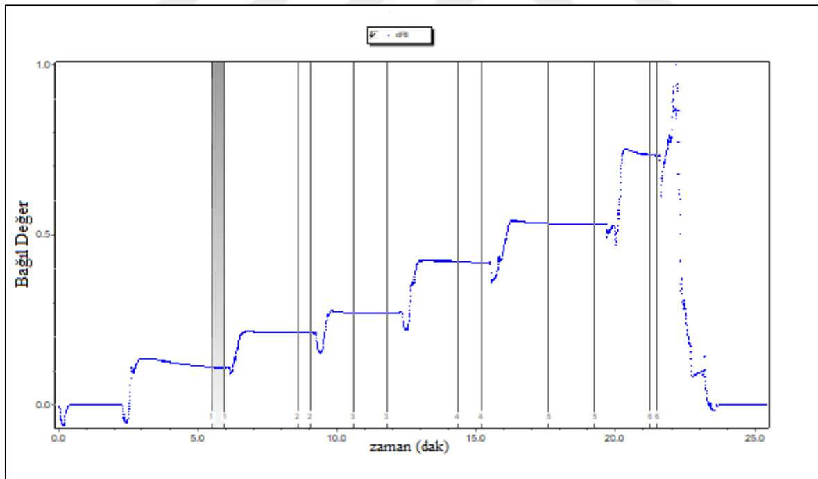
Şekil 2. Hiyalüronik asit kırılma indisi ( dn/dc ) grafiğinde belirlenen piklerin gösterimi
