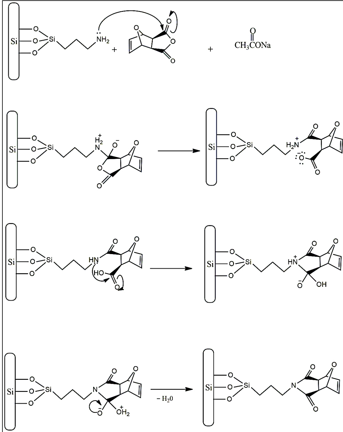
Şekil 4.3. EHD monomerinin Si-APTES yüzeyine bağlanma mekanizmasının şematik gösterimi
