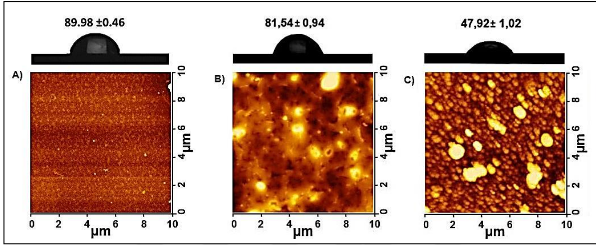
Şekil 4.4. 2D-AFM görüntüleri (altta) ve 4 \mu L su damlacıklarının fotoğrafları (üstte). (a) Si-EHDA, (b) Si-poli(EHDA) ve (c) Si-poli(EHDA)-HA
