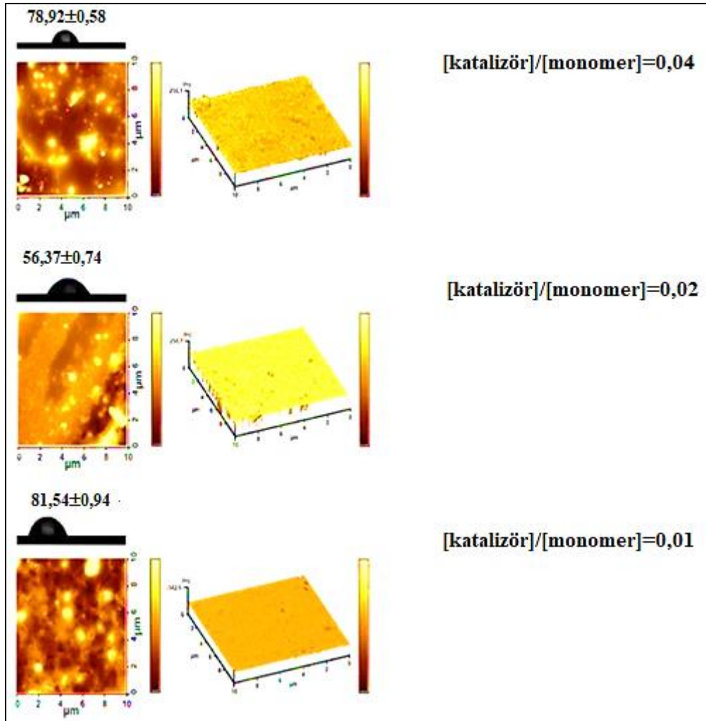
Şekil 4.10. Farklı [katalizör]/[monomer] oranlarında sentezlenen poli(EHDA) fırçalarının 3- ve 2-boyutlu AFM ve su damlacıklarının görüntüleri
