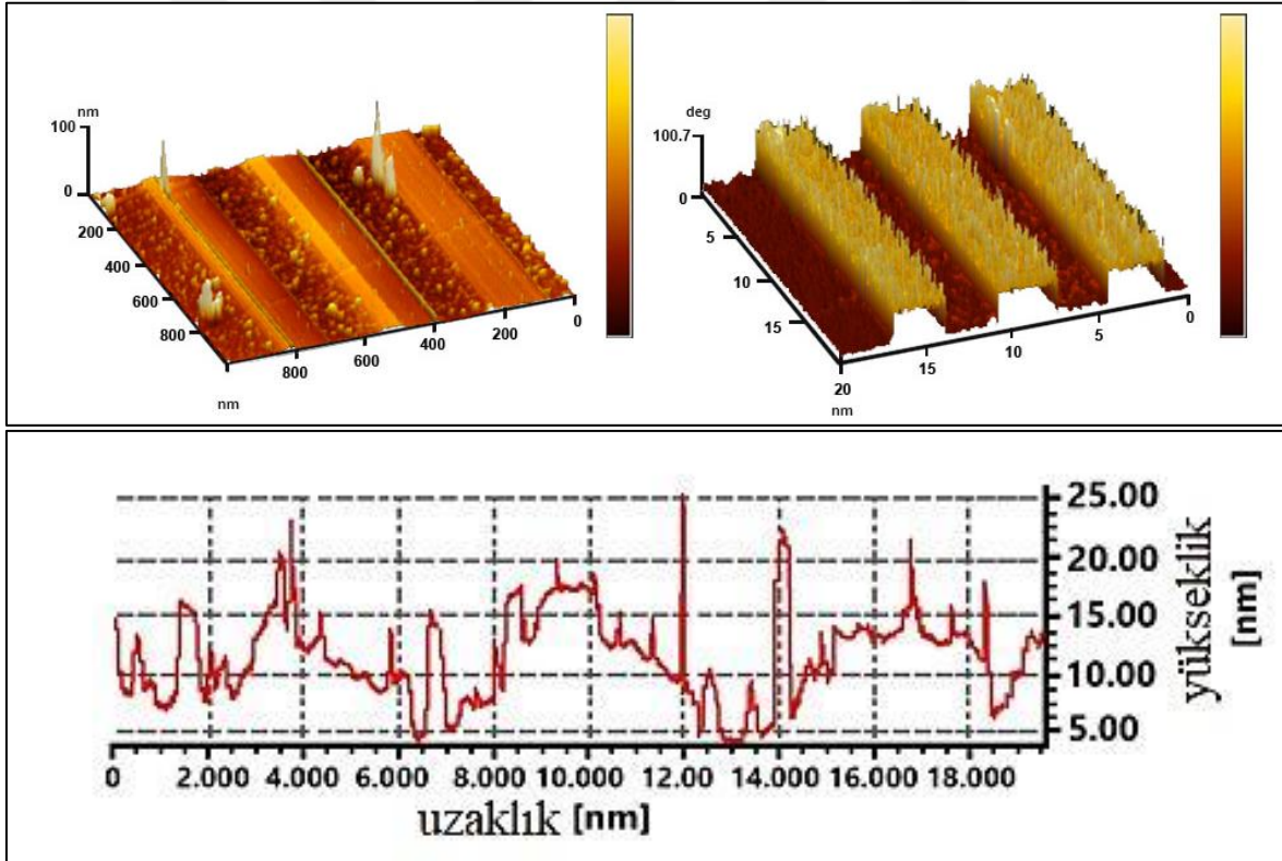
Şekil 4.24. Nano desenlenmiş Si-EHDA yüzeyin 3D-AFM (a) topolojik ve (b) faz görüntüleri
