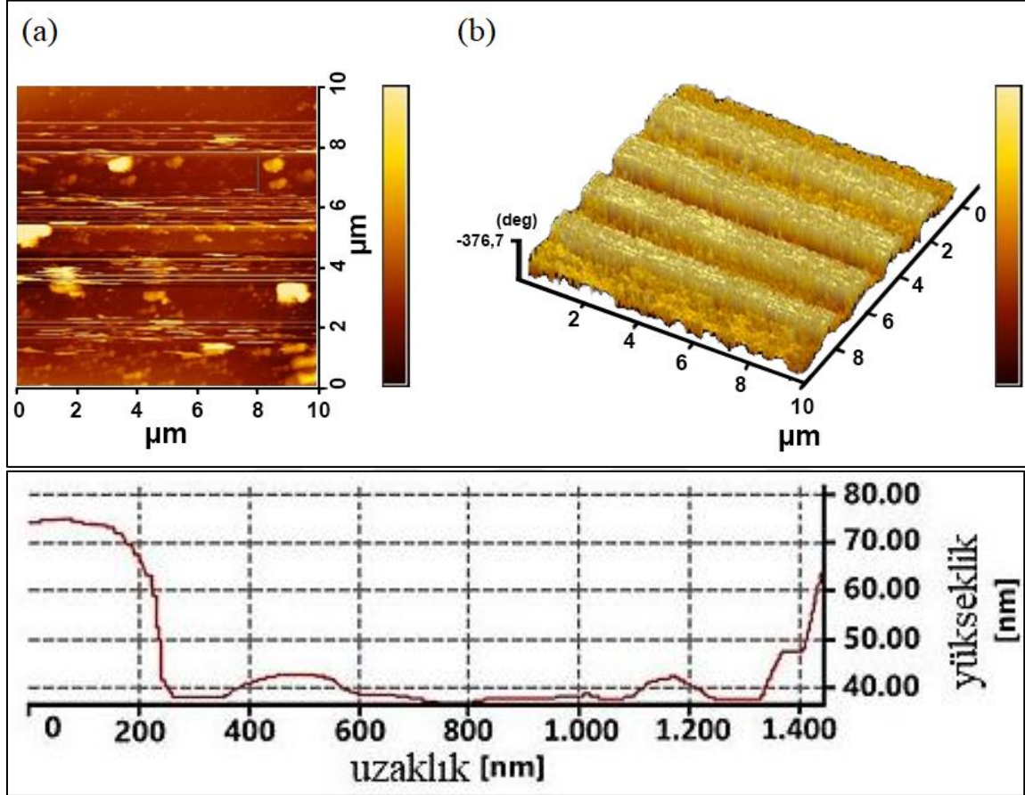
Şekil 4.30. AFM nanolitografi yöntemiyle Si-poli(EHDA)-HA yüzeyinde 4 çizgi çiziminin AFM (a) topolojik ve (b) faz görüntüleri
