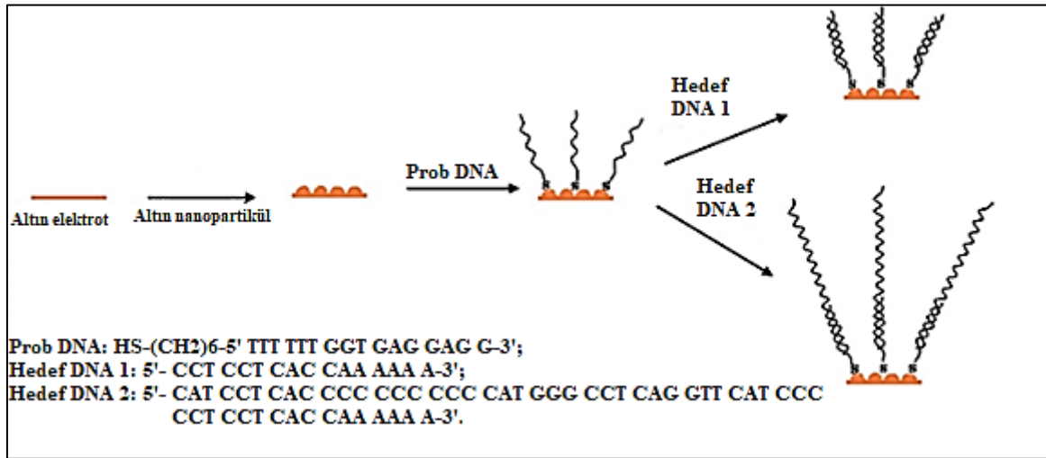
Şekil 2.36. Modifiye edilmiş SsDNA probu ile üretilen altın nanopartikül sentezinde yer alan adımların ve bu nanopartiküllerin farklı hedef DNA ile hibridizasyonlarının şematik gösterimi (Liu,2005)
