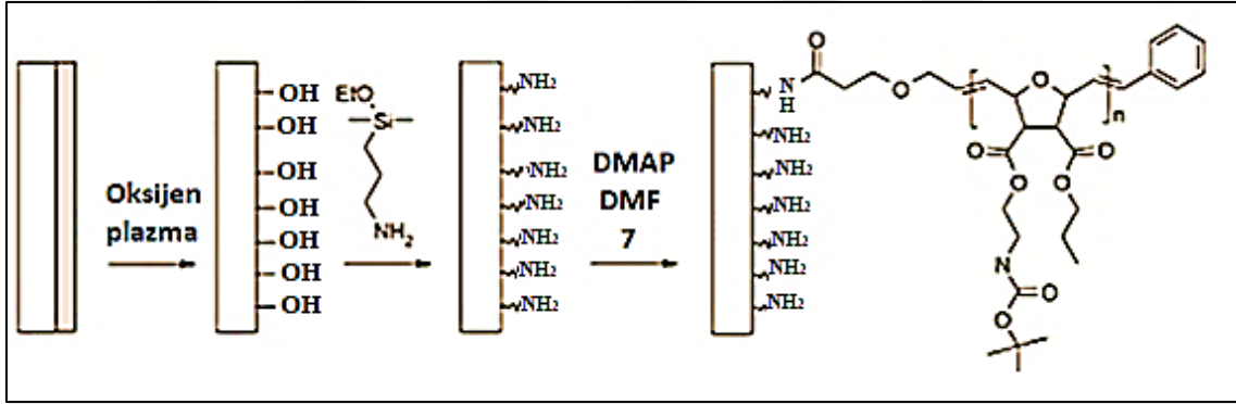
Şekil 2.15. Yüzey fonksiyonlaştırma basamakları (Madkour,2010)
