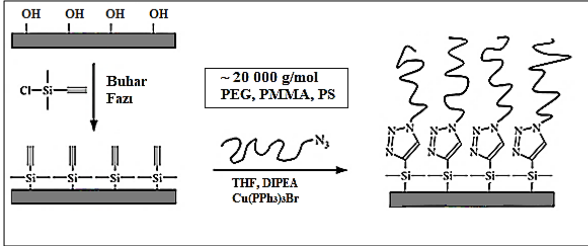
Şekil 2.3. Polimer fırçaların klik kimyası yöntemiyle "Pasifize" silisyum yüzeylere aşılama yönteminin şematik gösterimi (Ostaci, 2008)
