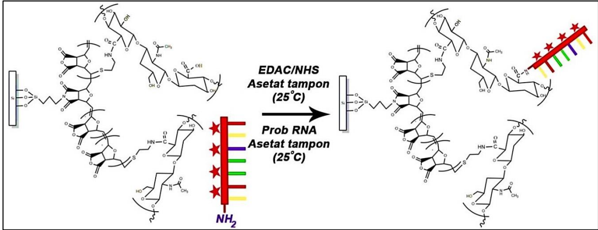
Şekil 4.31. Poli(EHDA)-HA fırçalara tek zincir RNA probunun bağlanmasının şematik görünümü
