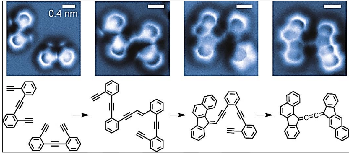
Şekil 2.25. Basamaklı bimoleküler enediyen birleşmesi ve siklizasyon basamağında ara ürünlerin deneysel gözlemi (Riss, 2016)
