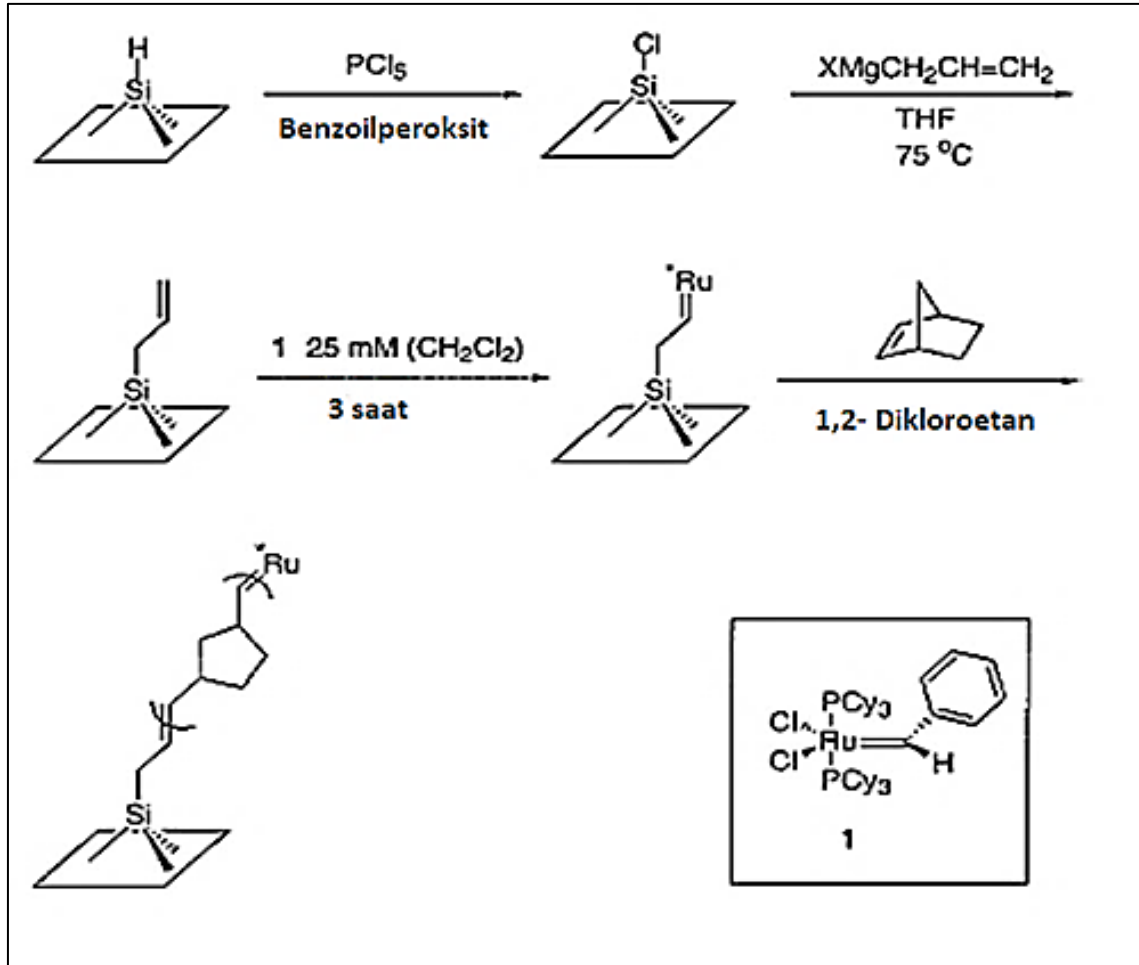
Şekil 2.16. Yüzey modifikasyon süreci ( Juang, 2001)
