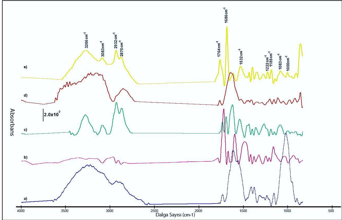
Şekil 4.18. HA ve Si-poli(EHDA)-HA fırçaların GA-FTIR spektrumları. a) HA ve (b) [katalizör]/[monomer]=0,09 , (c) [katalizör]/[monomer]=0,04 , (d) [katalizör]/[monomer]=0,02 , (e) [katalizör]/[monomer]=0,01
