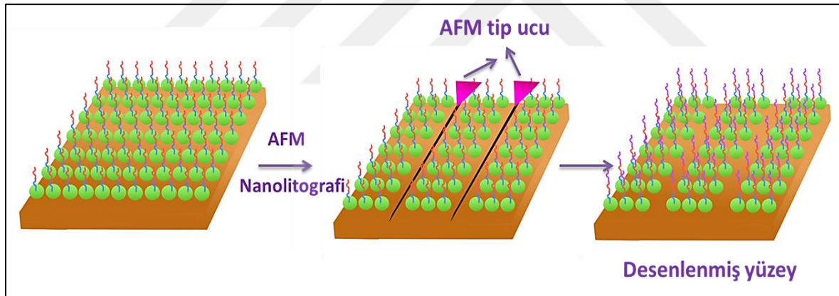
Şekil 4.22. AFM ile uygulanan nanolitografi işleminin şematik gösterimi
