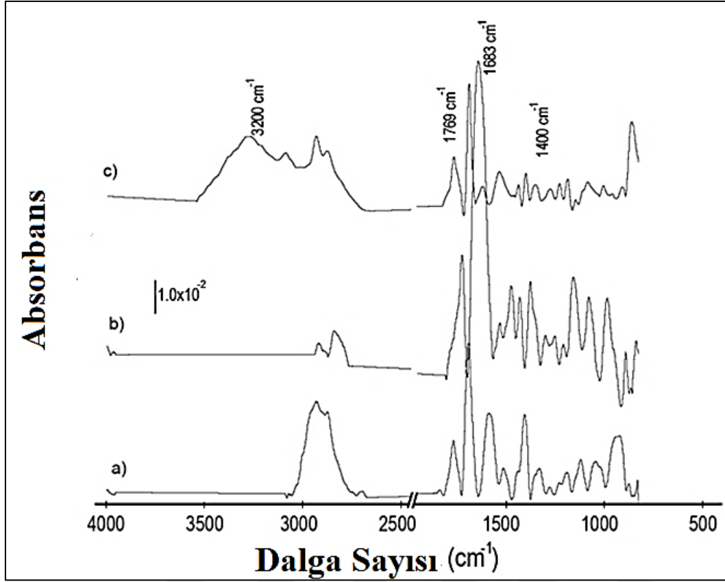
Şekil 4.6. GA-FT-IR spektrumları (a) Si-EHDA, (b) Si-poli(EHDA) ve (c) Si-poli(EHDA)-HA
