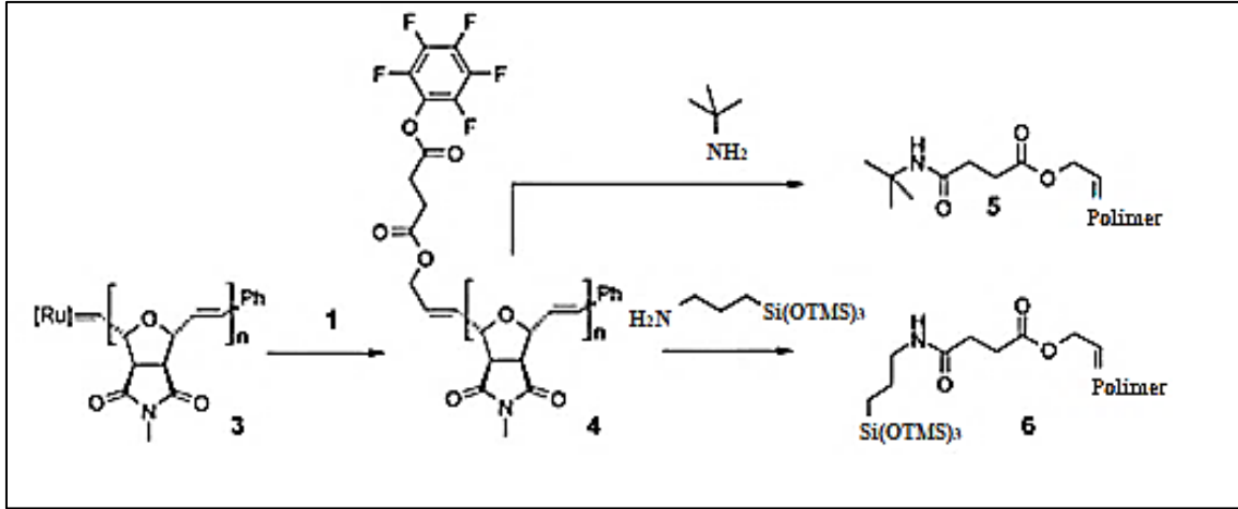
Şekil 2.14. Polimer 3 ve 4'ün polimer-analog tepkimeleri ve son gruplarının fonksiyonlaştırılması (Madkour,2010)
