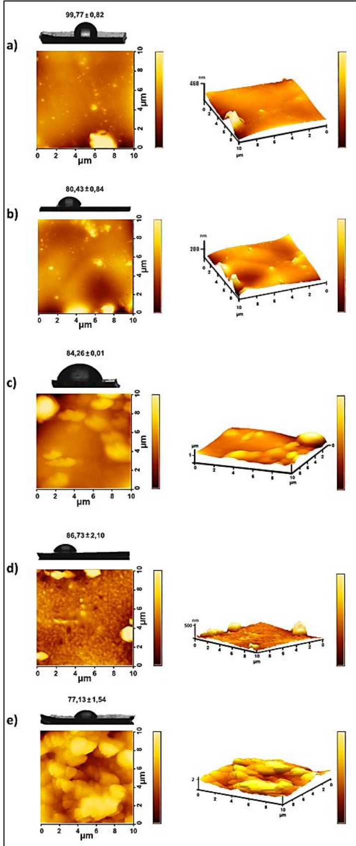
Şekil 4.9. Farklı sürelerde a) 1 sa, b) 3 sa, c) 6 sa, d) 16 sa ve e) 24 sa hazırlanan poli(EHDA) fırçaların 2- ve 3-boyutlu AFM, yükseklik dağılım ve su damlacığı görüntüleri
