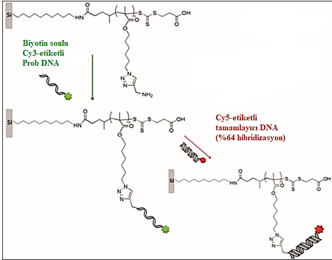
Şekil 2.38. Mikro-desenli poli(AHMA) fırçaların oluşturulması ve DNA hibridizasyonunda kullanımın basamaklı üretim sürecinin şematik gösterimi (Çimen, 2015)
