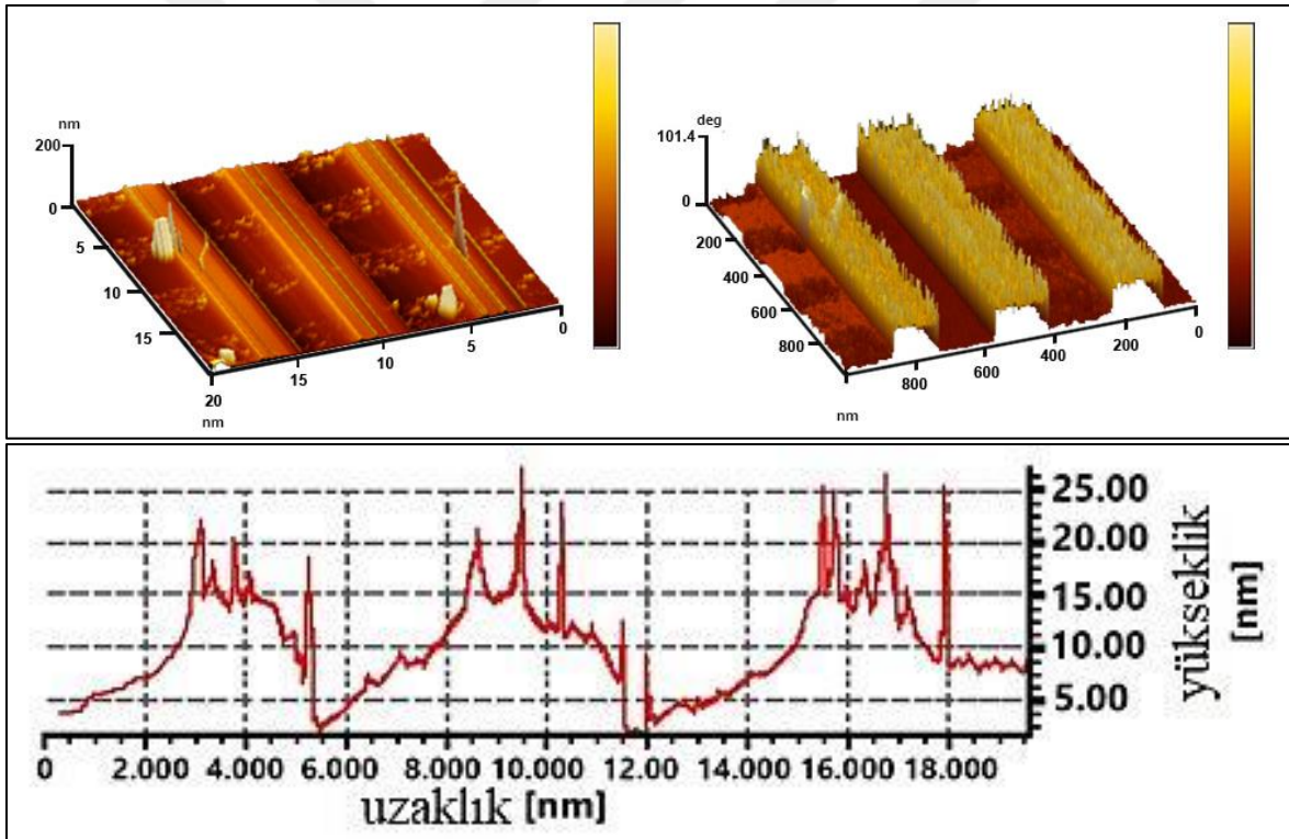
Şekil 4.26. AFM nanolitografi yöntemiyle yüzeyde yatay 3 çizgi çizimi üzerine dikey 3 çizgi çiziminin 3D-AFM (a) topolojik ve (b) faz görüntüleri
