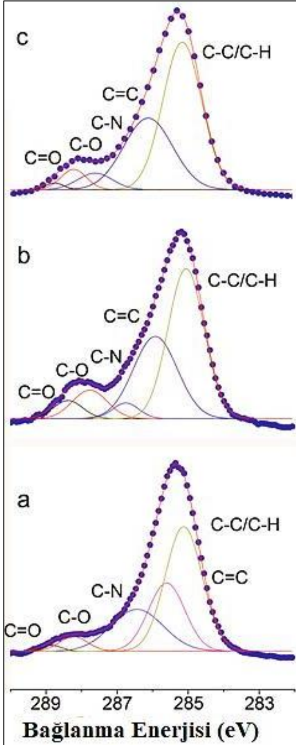
Şekil 4.5. C1s kısmi taramalı XPS spektrumları (a) Si-EHDA, (b) Si-poli(EHDA) ve (c) Si-poli(EHDA)-HA
