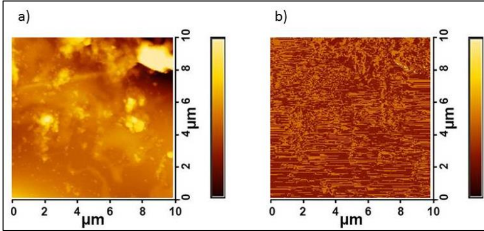
Şekil 4.36. Poli(EHDA)-HA-probRNA-DNA yüzeyinin 2D-AFM (a) topolojik ve (b) faz görüntüleri
