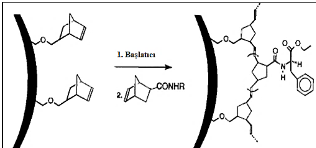
Şekil 2.29. Bileşik III'ün PS-DVB (Gözenekli polistiren/divinil benzen kopolimerleri) yüzeye aşılması ve ROMP'un gerçekleştirilmesi (Buchmeiser, 2000)
