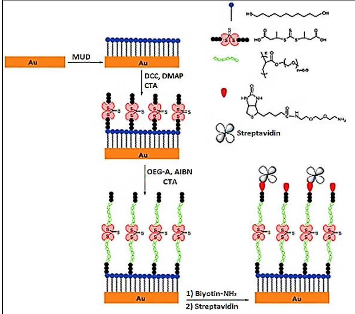
Şekil 2.41. Streptavidin immobilize edilmiş poli(OEGA) fırçaların oluşturmanın basamaklı üretim sürecinin şematik gösterimi (Zengin, 2012)
