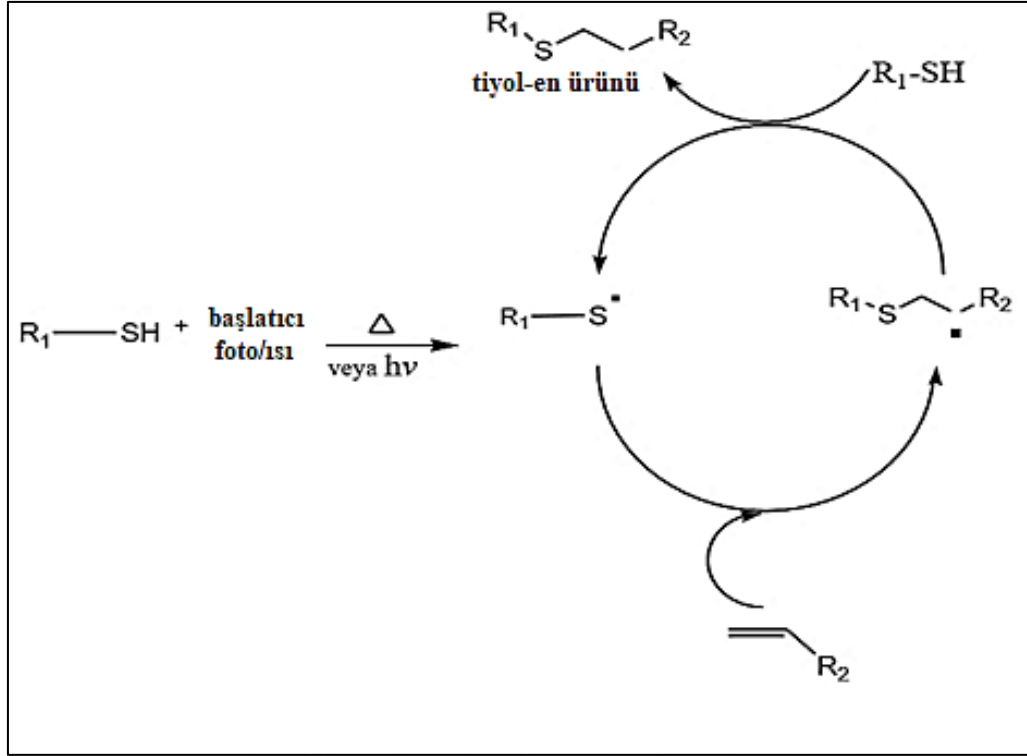
Şekil 2.19. Radikal tiyol-en tepkime mekanizmasının şematik gösterimi (Lowe, 2010)
