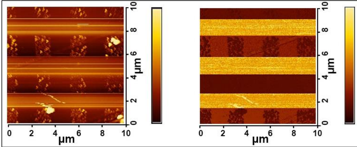
Şekil 4.25. AFM nanolitografi yöntemiyle yüzey üzerinde yatay 3 çizgi çizimi üzerine dikey 3 çizgi çiziminin 2D-AFM (a) topolojik ve (b) faz görüntüleri
