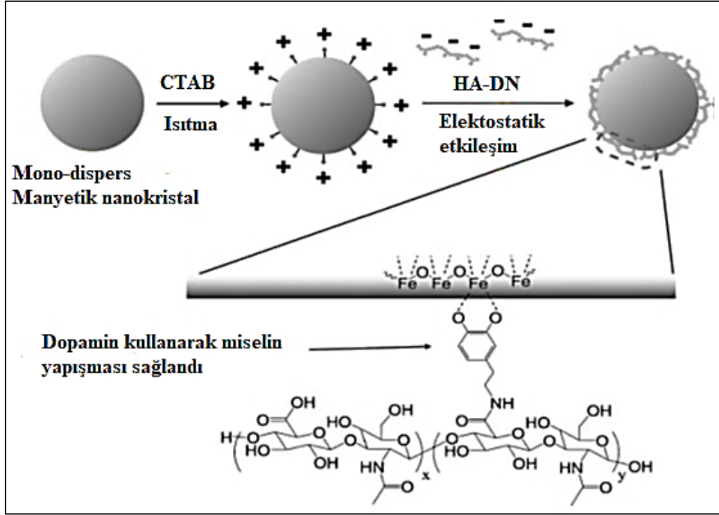
Şekil 2.34. Monodispers mıknatıs nanokristal üzerine homojen HA-DN'nin immobilizasyonu için sentetik süreç (HA-DN/MNC) (Lee, 2008)
