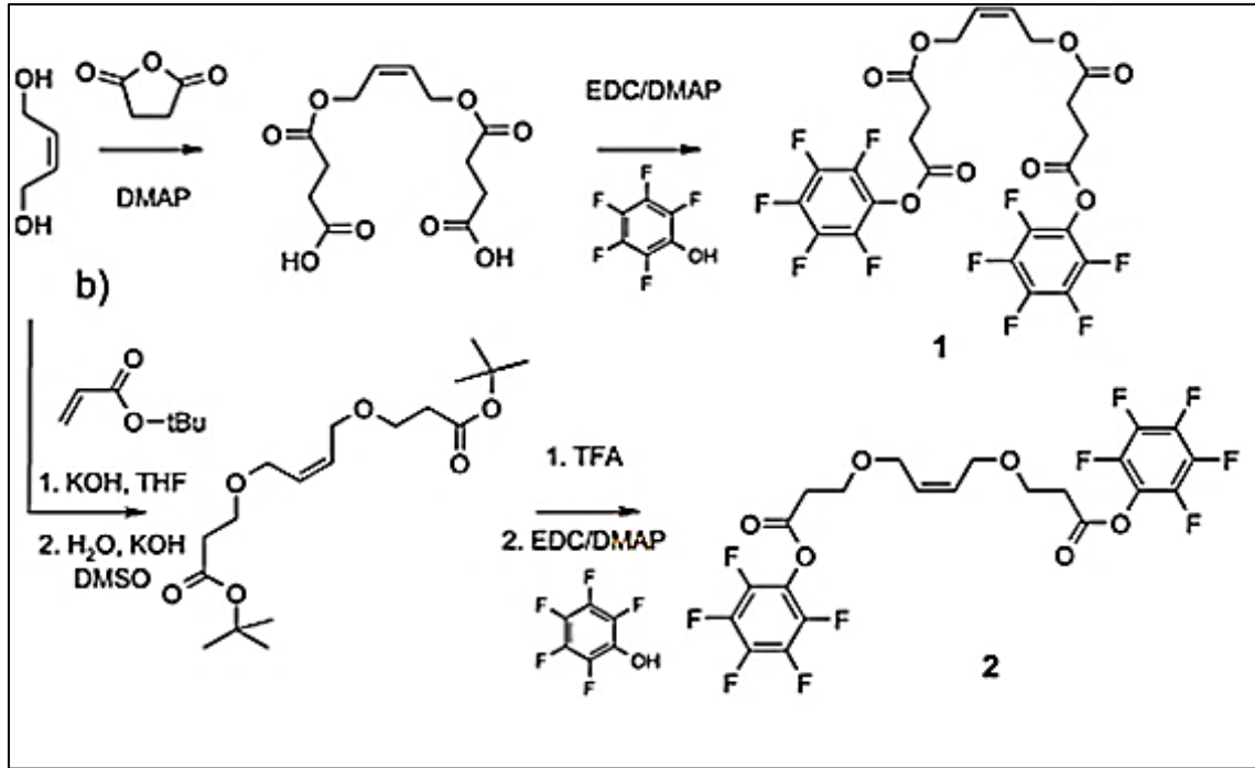
Şekil 2.12. Sonlandırıcı ajan molekülleri 1 ve 2'nin sentezi (Madkour,2010)
