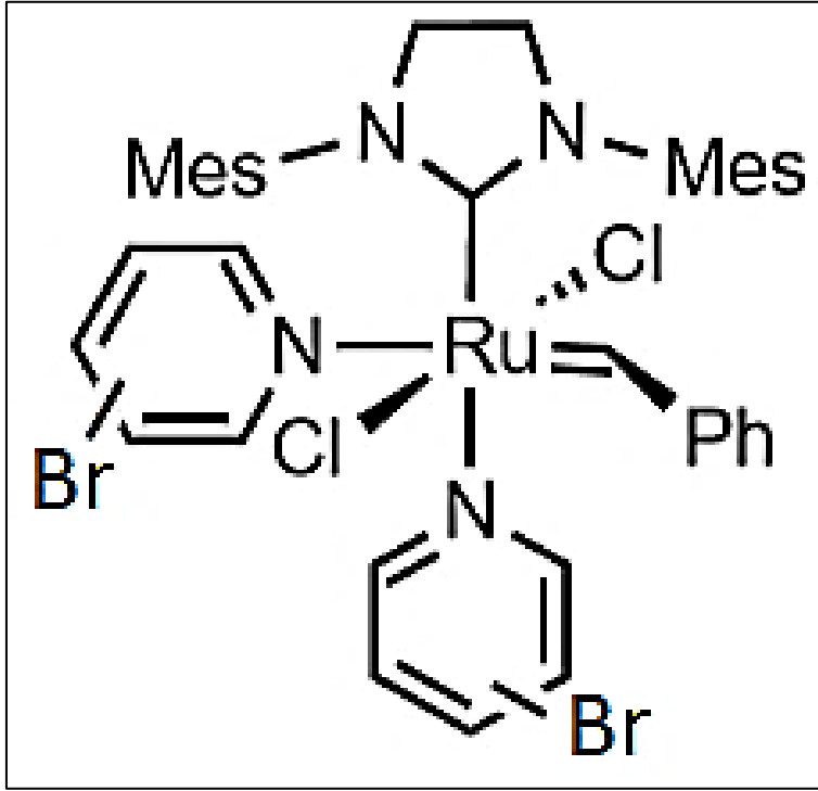
Şekil 4.7. Grubbs III metatez katalisti (Mes=2,4,6-trimetilfenil)
