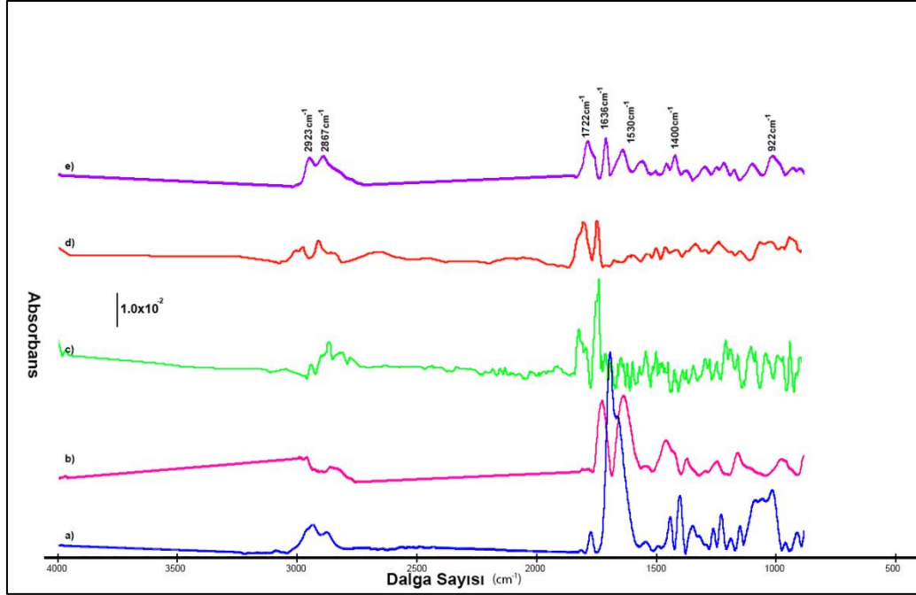
Şekil 4.11. Poli(EHDA)'nın GA-FTIR spektrumları, (a) Çözelti ortamında sentezlenen ve (b) [\text{katalizör}]/[\text{monomer}]=0,09 , (c) [\text{katalizör}]/[\text{monomer}]=0,04 , (d) [\text{katalizör}]/[\text{monomer}]=0,02 , (e) [\text{katalizör}]/[\text{monomer}]=0,01
