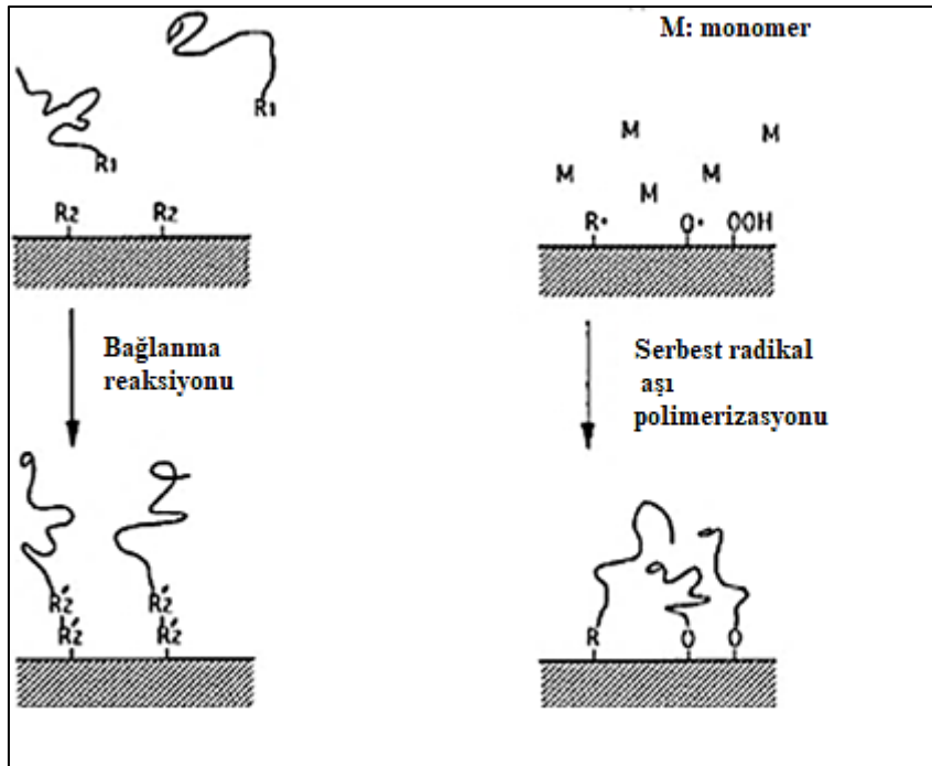
Şekil 2.30. Hazır polimer zincirlerinin bağlanma tepkimesi ve polimer zincirlerinin yüzeyde büyütülmesinin şematik gösterimi (Ikada,1994)
