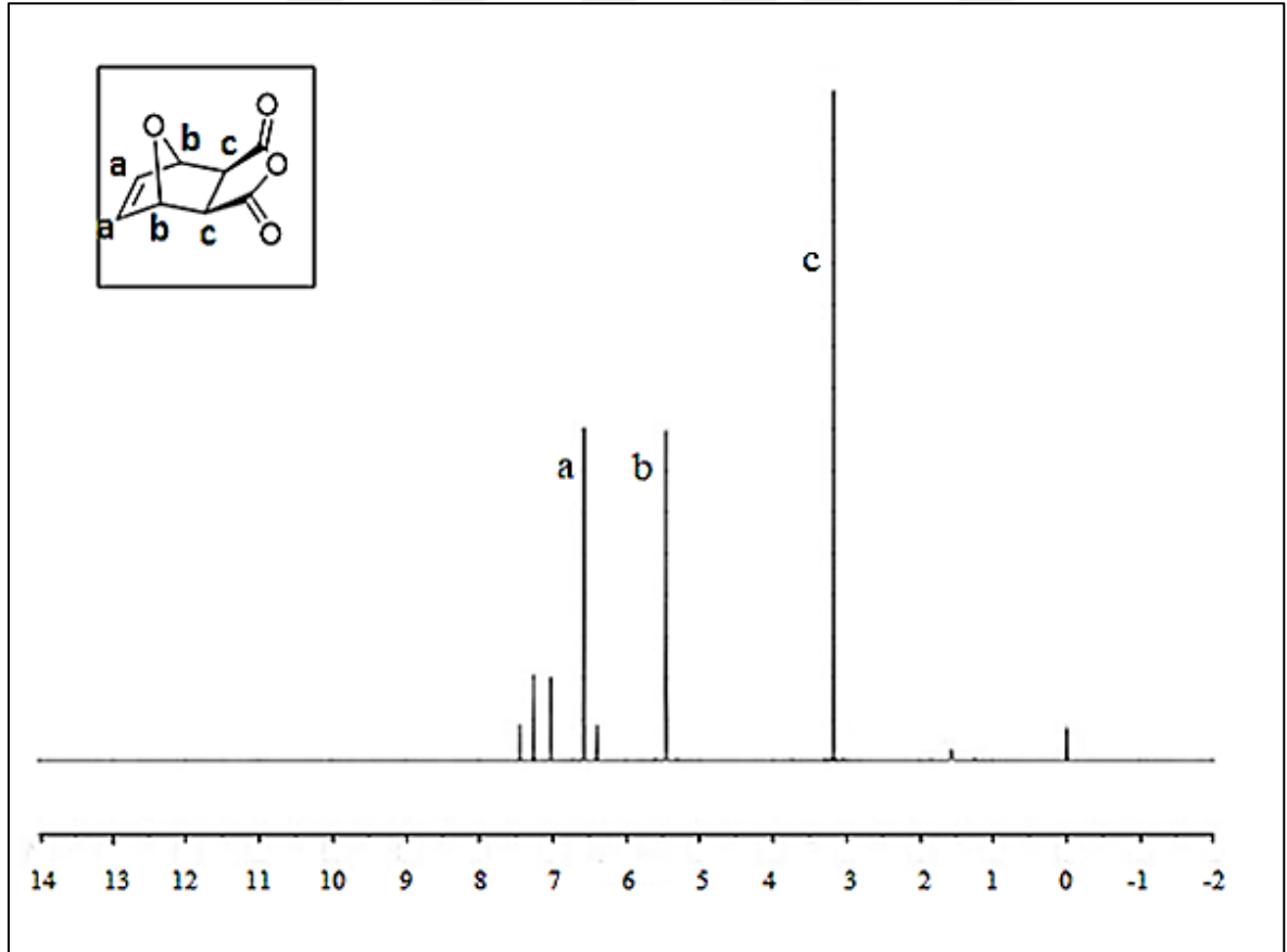
Şekil 4.2. EHDA monomerinin 1 H-NMR spektrumu
