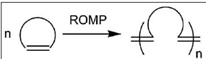
Şekil 2.6. ROMP'un genel gösterimi
