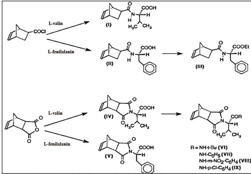
Şekil 2.28. Bileşik I-IX'un sentezi (Buchmeiser, 2000)
