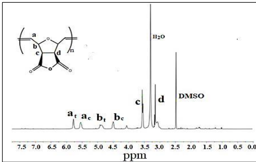
Şekil 4.13. Poli(EHDA)'nın ^1\text{H} -NMR spektrumu (Çözücü:DMSO)
