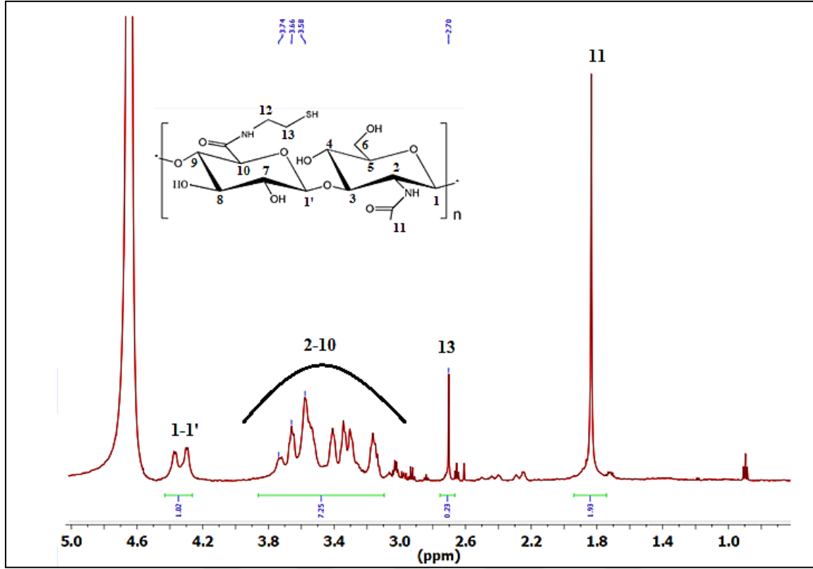
Şekil 4.17. Th-HA'nın ^1\text{H} -NMR spektrumu
