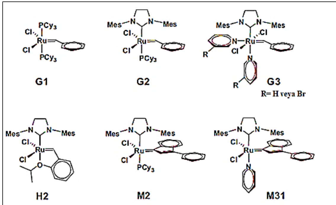
Şekil 2.10. Olefin ROMP’da kullanılan çeşitli Rutenyum esaslı katalizörler
