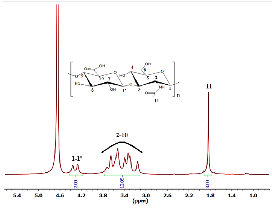
Şekil 4.16. Düşük mol kütleli HA'nın ^1\text{H} -NMR spektrumu
