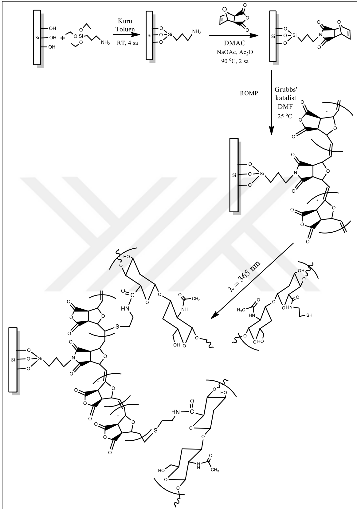
Şekil 4.8. Poli(EHDA)-HA fırçaların yüzeyde başlatılan ROMP ile sentezinin şematik gösterimi
