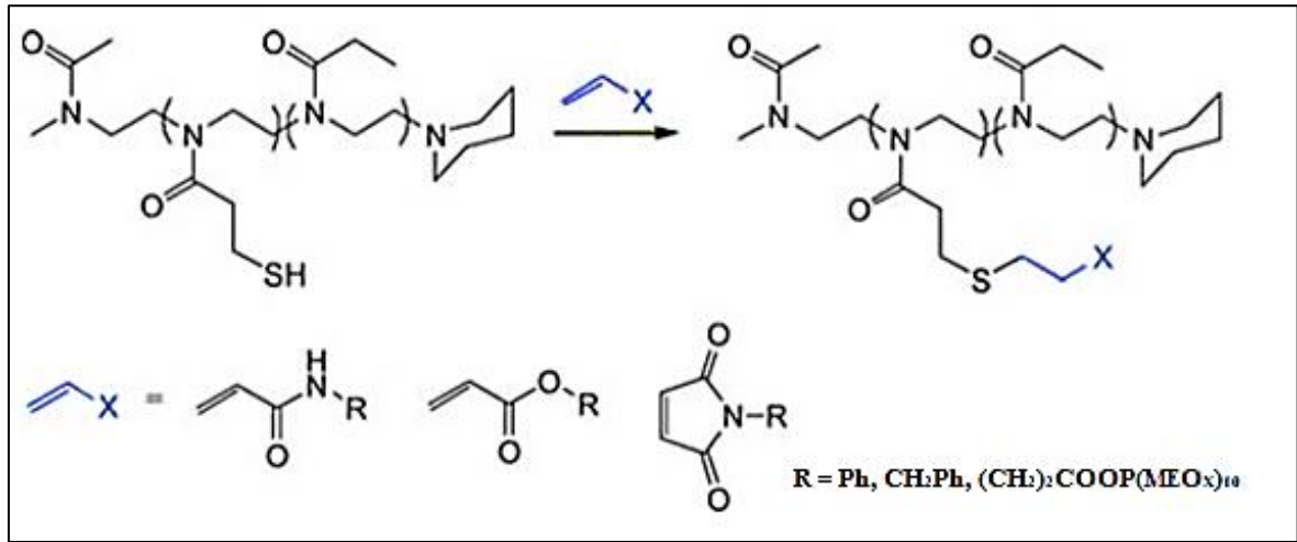
Şekil 2.18. Tiyol-Michael tepkimesi ile yan zinciri modifiye edilmiş poli(2-oksazolin)'lerin sentezi (Cesana,2007)
