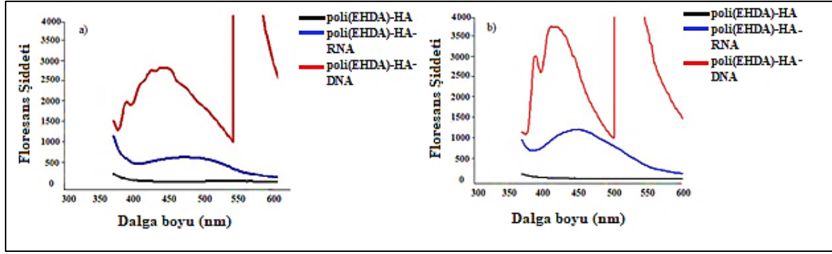
Şekil 4.35. İki farklı [katalizör]/[monomer] oranında a) 0,04, b) 0,02 hazırlanan poli(EHDA)-HA (siyah) poli(EHDA)-HA-probRNA (mavi), Poli(EHDA)-HA-probRNA-DNA (kırmızı) floresans spektrumları
