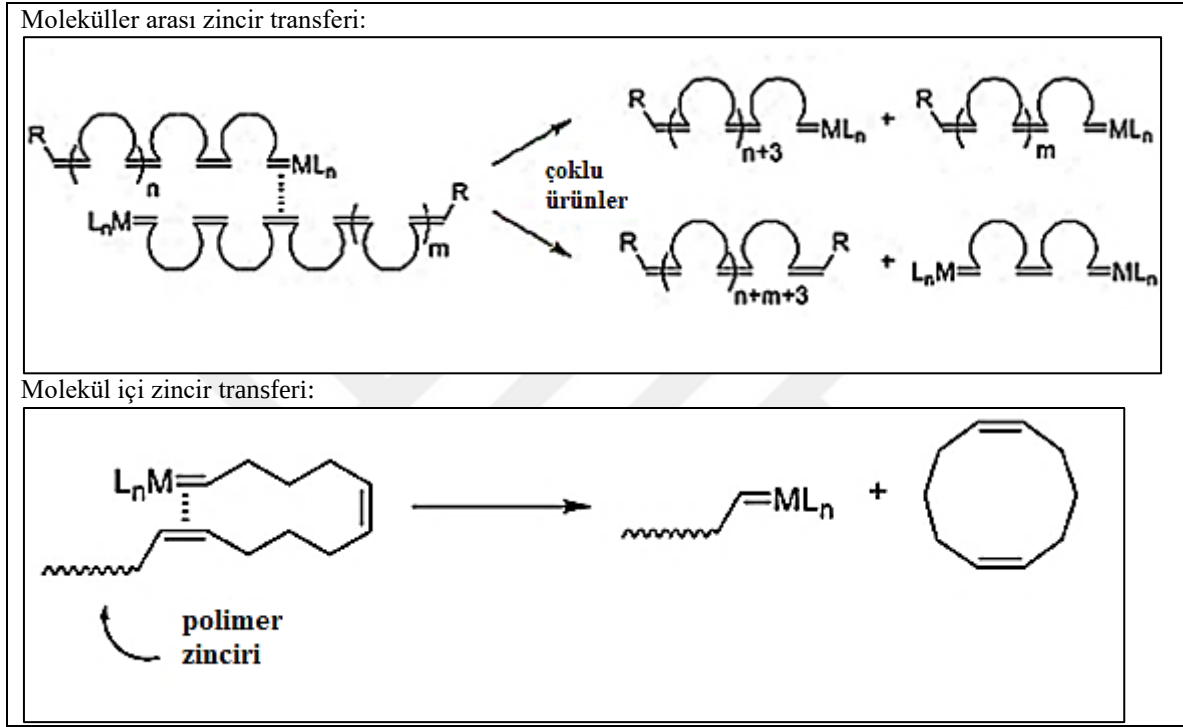
Şekil 2.9. ROMP tepkimelerinde ikincil metatez (moleküller arası zincir transfer ve molekül içi zincir transfer) tepkimelerin örnekleri
