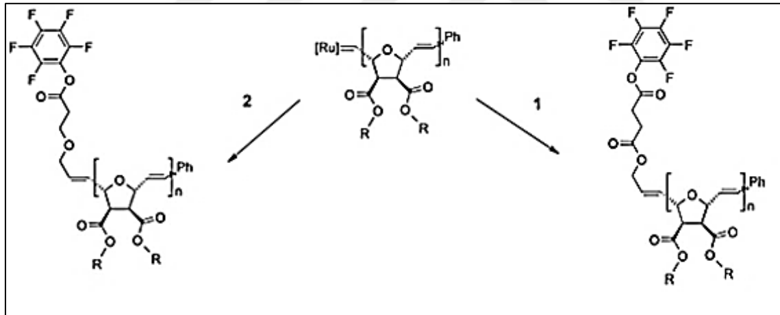
Şekil 2.13. Sonlandırma ajanları 1 (pentafluoroalkil ester) ve 2 (pentafluoroalileter) ile yaşanan ROMP polimerlerinin son gruplarının fonksiyonlaştırılması (Madkour,2010)
