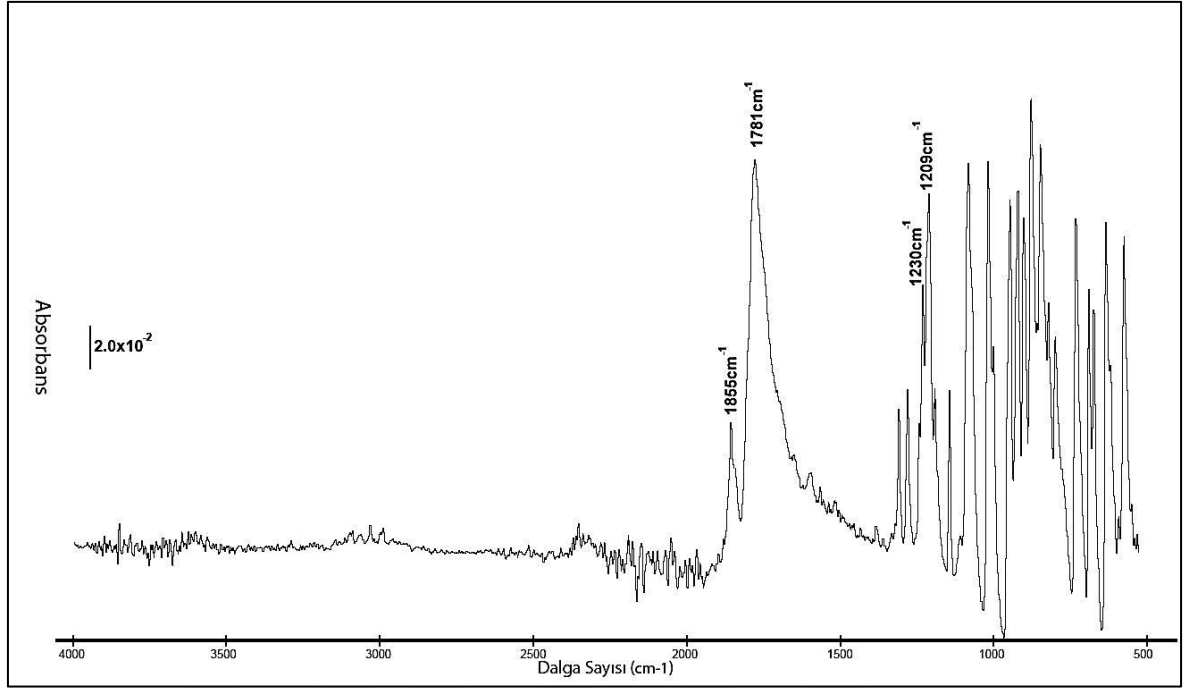
Şekil 4.1. EHDA monomerinin FTIR spektrumu
