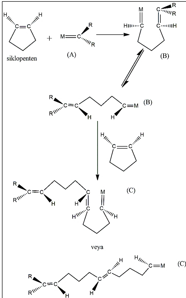
Şekil 2.7. Siklopentenin ROMP basamakları
