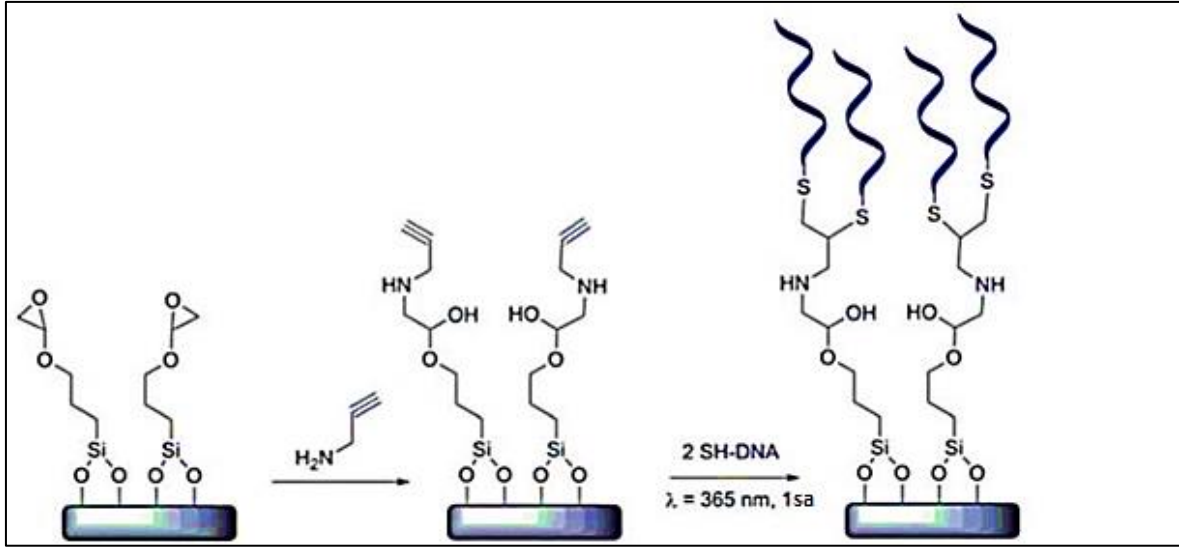
Şekil 2.37. Tiyollenmiş DNA'nın proparjilaminle modifiye edilmiş yüzey üzerine foto-başlatılmış tiyol tepkimesi ile bağlanmasının şematik gösterimi (Escorihuela, 2014)
