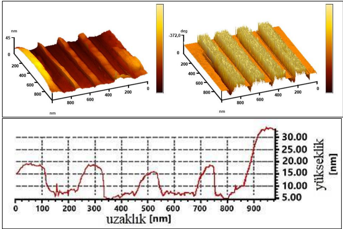
Şekil 4.27. AFM nanolitografi yöntemiyle yüzeyde yatay 3 çizgi çiziminin 3D-AFM (a) topolojik ve (b) faz görüntüleri
