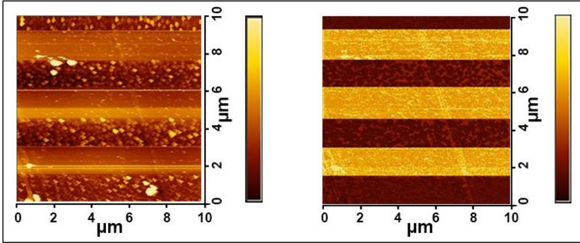
Şekil 4.23. Nano desenlenmiş Si-EHDA yüzeyin 2D-AFM (a) topolojik ve (b) faz görüntüleri
