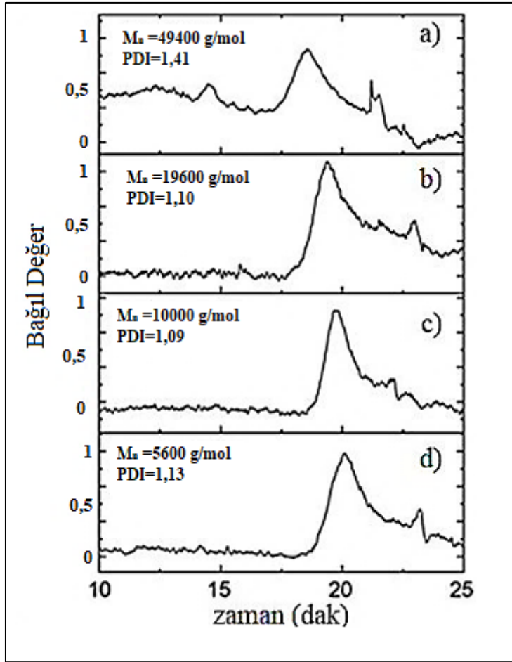
Şekil 4.12. Farklı [katalizör]/[monomer] oranında sentezlenen poli(EHDA)'nın farklı molekül ağırlıklarının GPC kromotogramları. [katalizör]/[monomer] oranları; a) 0,01, b) 0,02, c) 0,04 ve d) 0,09
