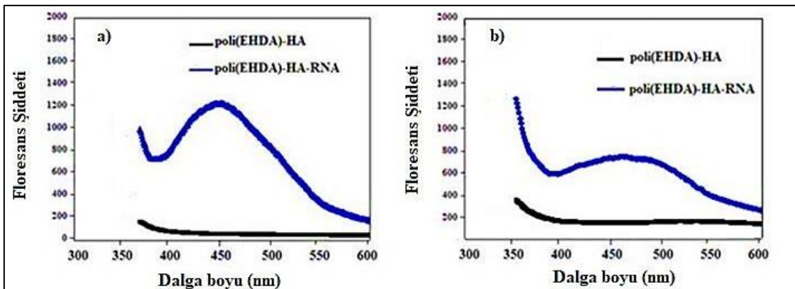
Şekil 4.32. Farklı [katalizör]/[monomer] oranında a) 0,04, b) 0,02 hazırlanan poli(EHDA)-HA (siyah) ve poli(EHDA)-HA-prob RNA (Hoechst 33258 boyasının spektrumu) sistemlerinin floresans spektrumları
