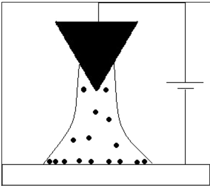
Şekil 2.23. Elektrokimyasal AFM nanolitografinin şematik gösterimi (Mart'ın, 2005)
