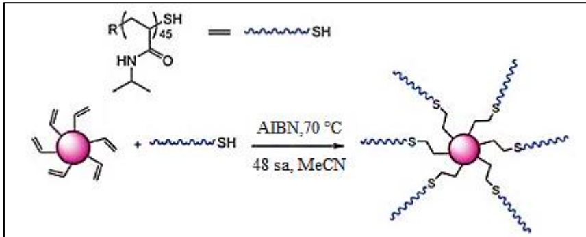
Şekil 2.20. PDVB nanopartiküllerinin radikalik tiyol-en yöntemi yüzey modifikasyonunun genel gösterimi (Goldmann, 2009)
