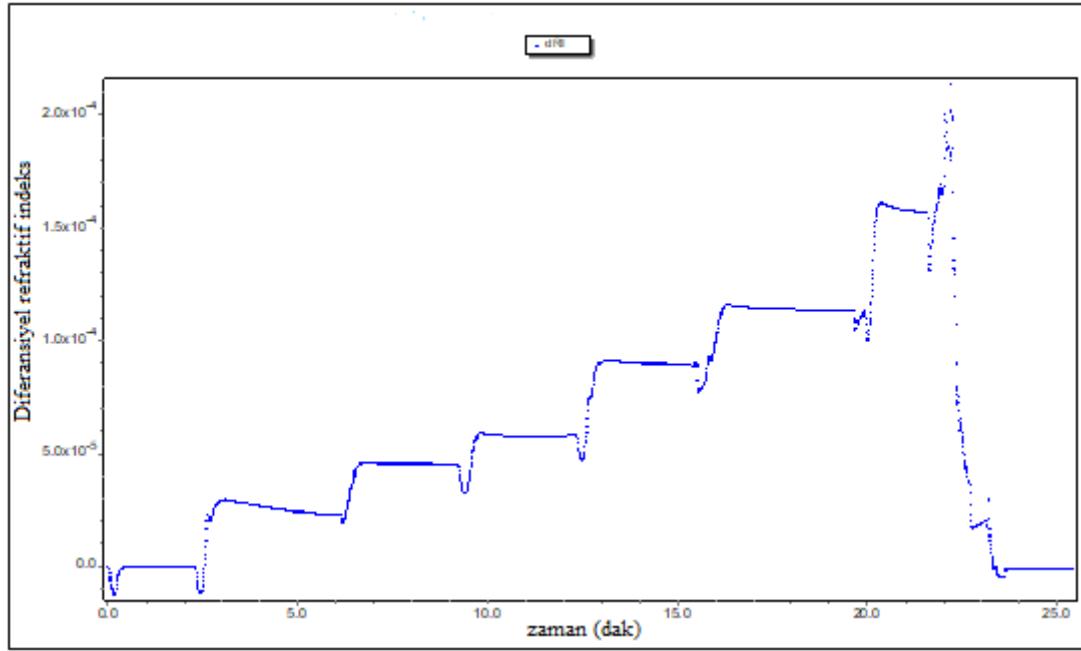
Şekil 1. Hiyalüronik asit kırılma indisi ( dn/dc ) grafiği
