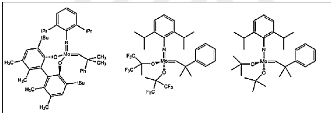
Şekil 2.11. Çeşitli Molibden esaslı Schrock katalizörleri
