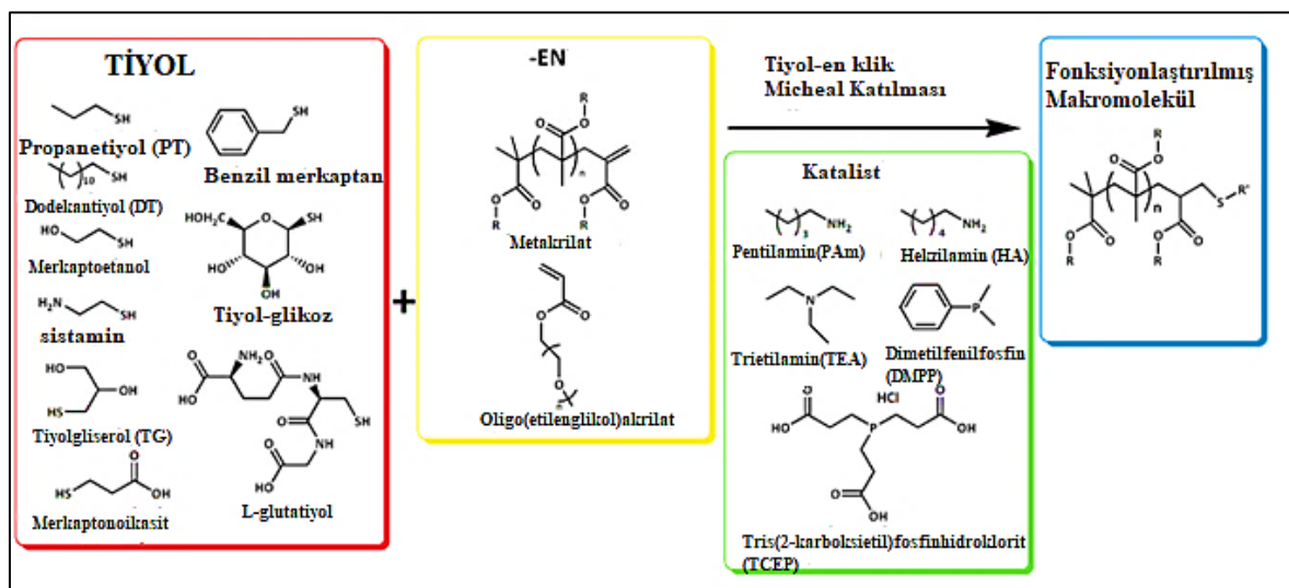
Şekil 2.17. Tiyol-en klik Michael katılma reaksiyonu için kullanılan tiyollerin, katalistlerin şematik gösterimi (Li, 2010)
