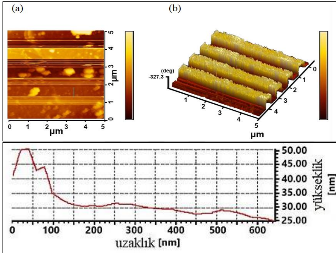
Şekil 4.29. AFM nanolitografi yöntemiyle Si-poli(EHDA) yüzeyinde 4 çizgi çiziminin AFM (a) topolojik ve (b) faz görüntüleri
