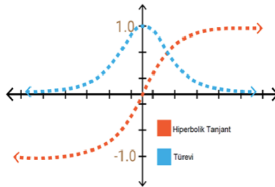
Şekil 2.8. Hiperbolik tanjant fonksiyonu ve türevi.
