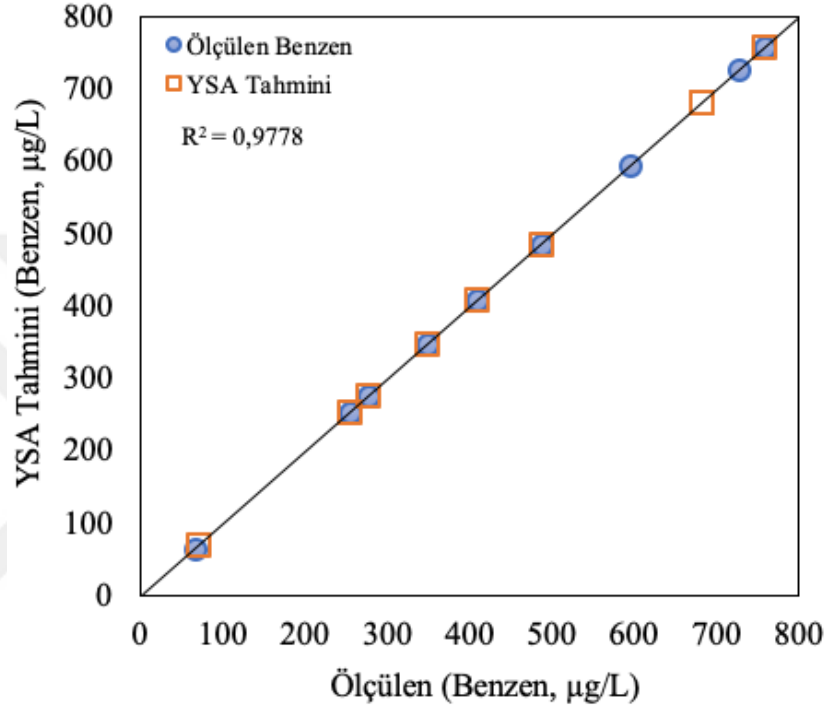
Şekil 4.18. YSA tahmini ve ölçülen benzen değerlerinin karşılaştırılması.
