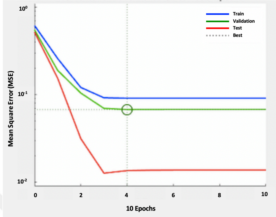
Şekil 4.15. YSA modelinin eğitim, validasyon ve test hataları.
