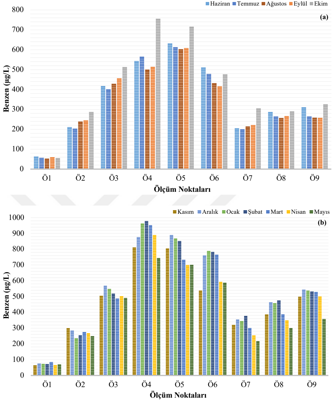
Şekil 4.8. Benzen konsantrasyonlarının (a) kurak ve (b) yağışlı mevsimler için dağılımı.
