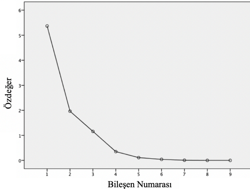
Şekil 4.9. Faktör analizi.
