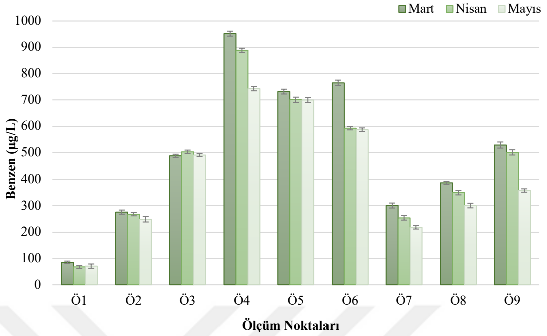
Şekil 4.5. Mart, Nisan ve Mayıs aylarına ait benzen konsantrasyonları.
