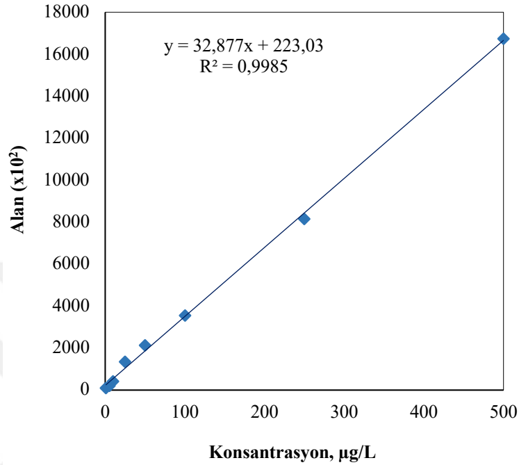
Şekil 3.7. Benzen kalibrasyon grafiği.
