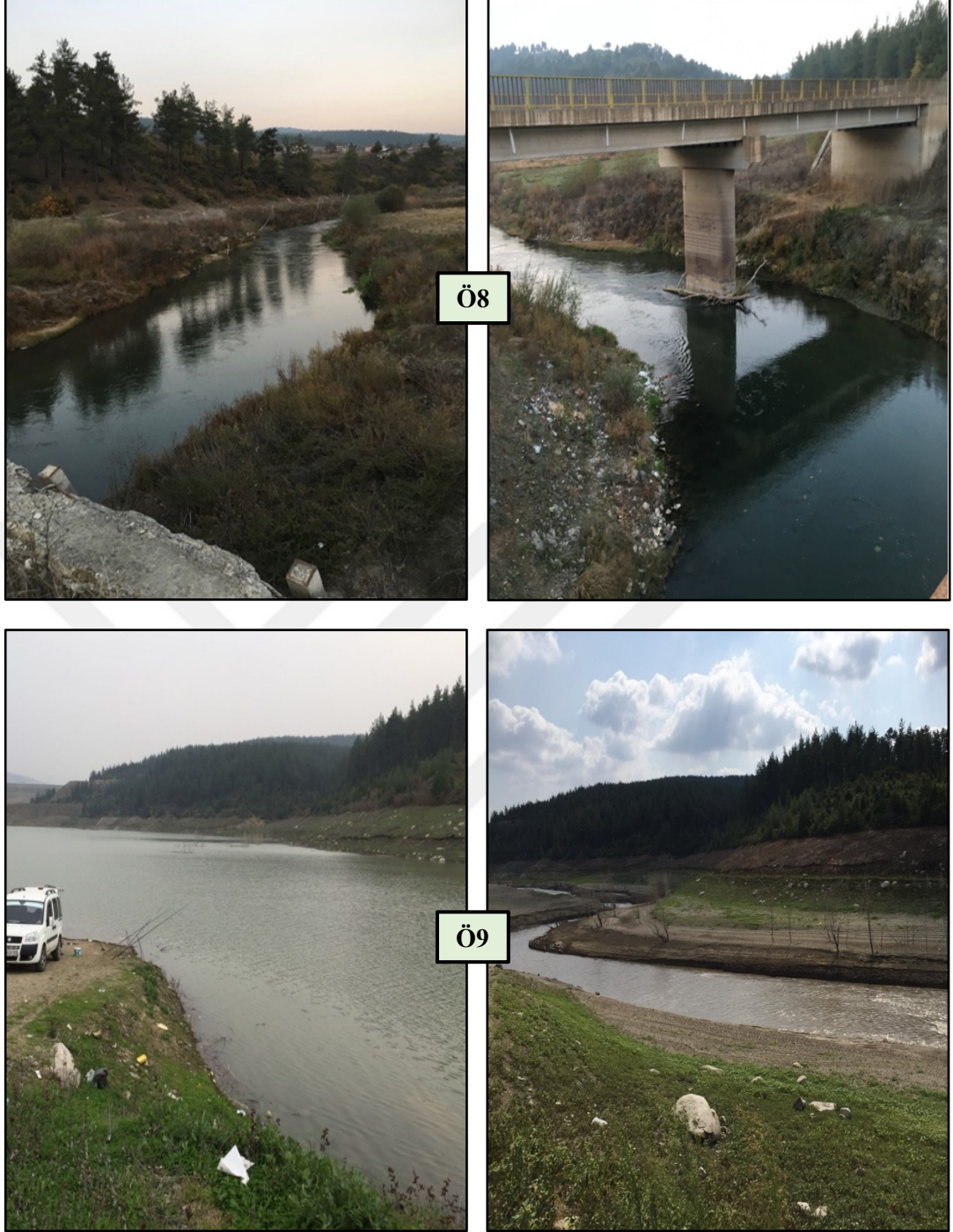
Şekil 3.4 (devam). Numune alma noktalarından görüntüler.
