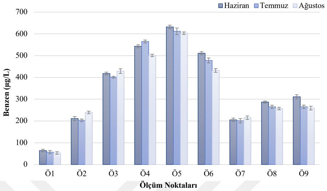
Şekil 4.6. Haziran, Temmuz ve Ağustos ayına ait benzen konsantrasyonları.
