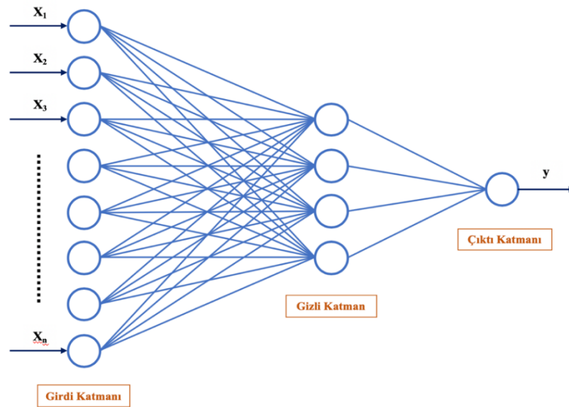
Şekil 2.3. YSA modeli.
