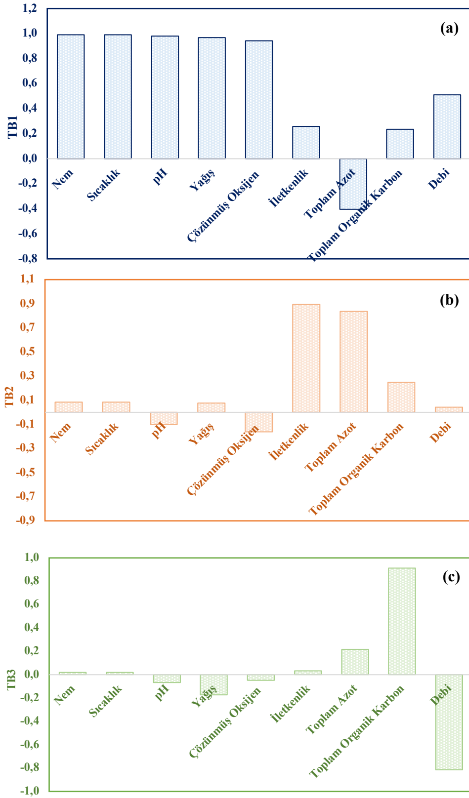
Şekil 4.11. (a) TB1, (b) TB2 ve (c) TB3 için bileşen özdeğerleri.
