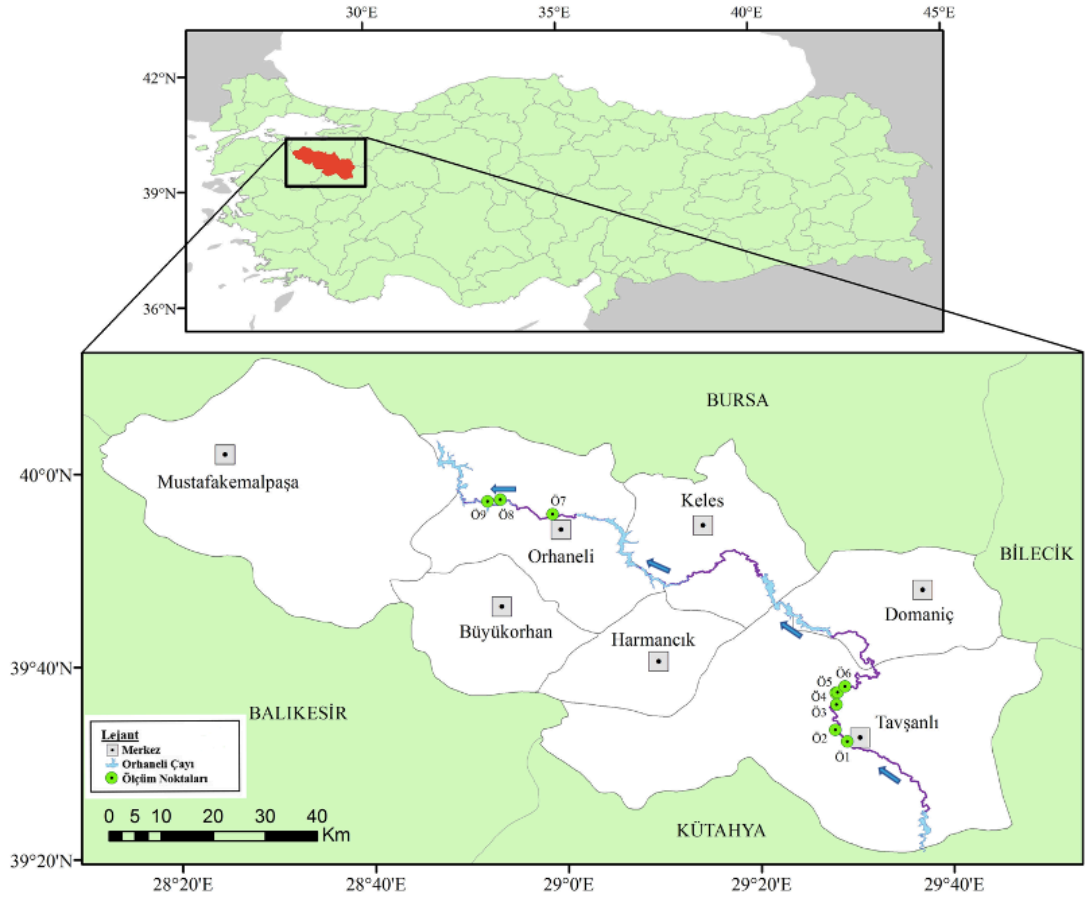
Şekil 3.2. Orhaneli Çayı su yolu gösterimi.
