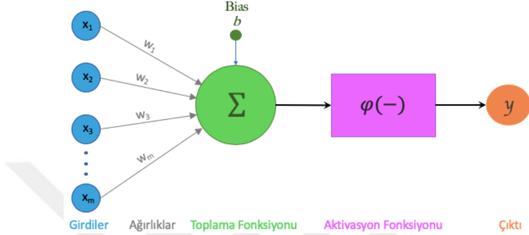
Şekil 2.4. YSA elemanlarının yapısı.
