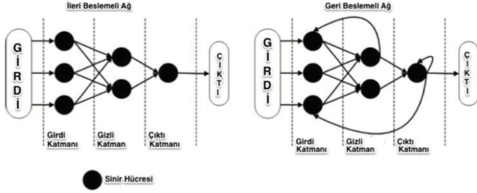
Şekil 2.12. İleri ve geri beslemeli ağ topolojisi.
