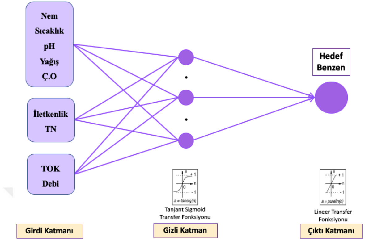
Şekil 3.9. Kullanılan YSA modelinin topolojik yapısı.
