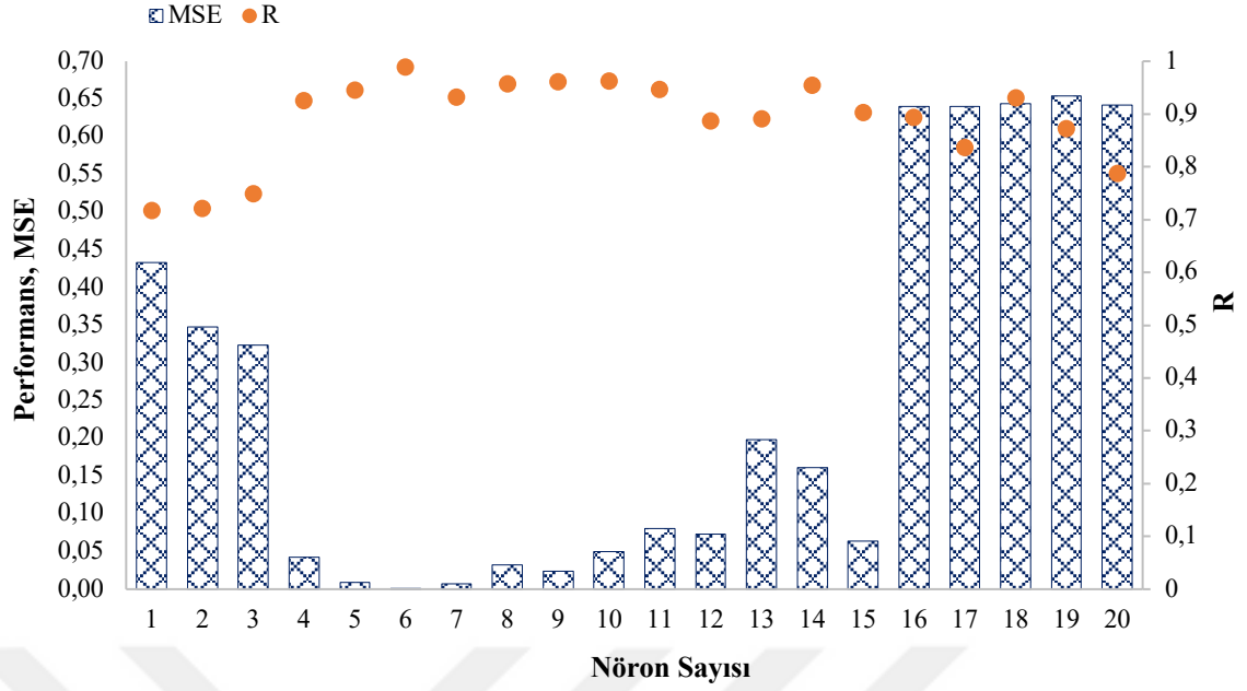
Şekil 4.12. YSA modeline nöron sayısının etkisi.
