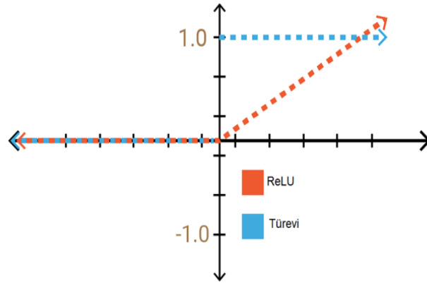
Şekil 2.9. ReLU fonksiyonu ve türevi.
