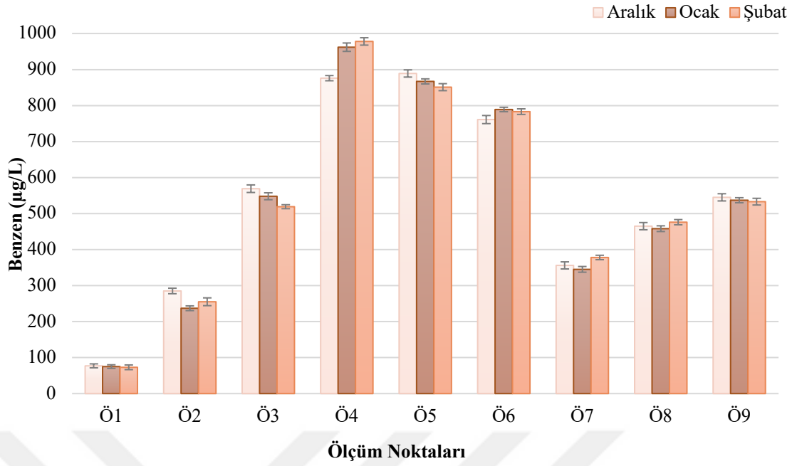
Şekil 4.4. Ocak, Şubat ve Aralık aylarına ait benzen konsantrasyonları.
