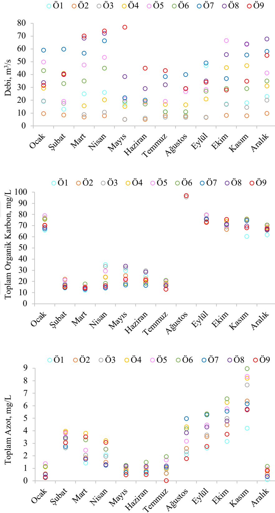
Şekil 4.2 (devam). Orhaneli Çayı çözünmüş oksijen, iletkenlik, pH, debi, toplam azot ve toplam organik karbon ölçümleri.
