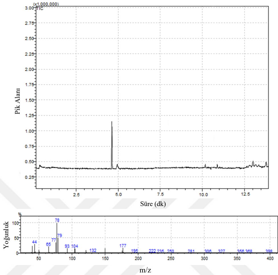
Şekil 3.8. Benzen analizine ait bir kromotogram ve karakteristik iyonları (m/z).
