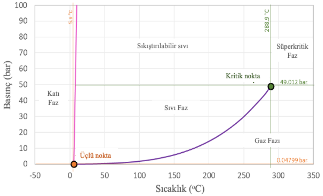
Şekil 2.1. Benzen için faz diyagramı.
