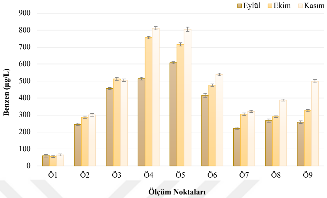
Şekil 4.7. Eylül, Ekim ve Kasım aylarına ait benzen konsantrasyonları.
