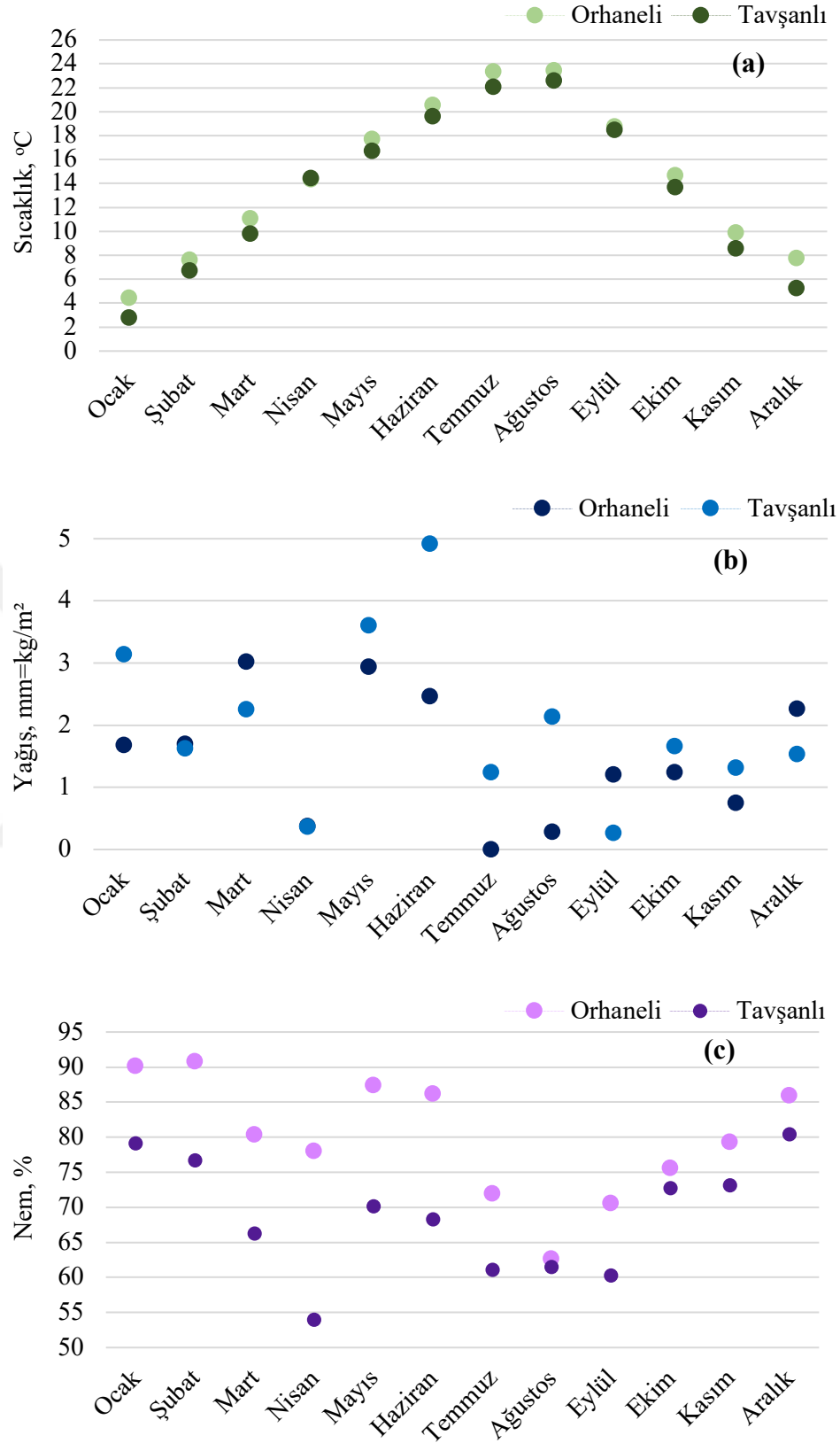
Şekil 4.1. 2018 yılı aylık ortalama (a) sıcaklık, (b) yağış miktarları ve (c) nem.
