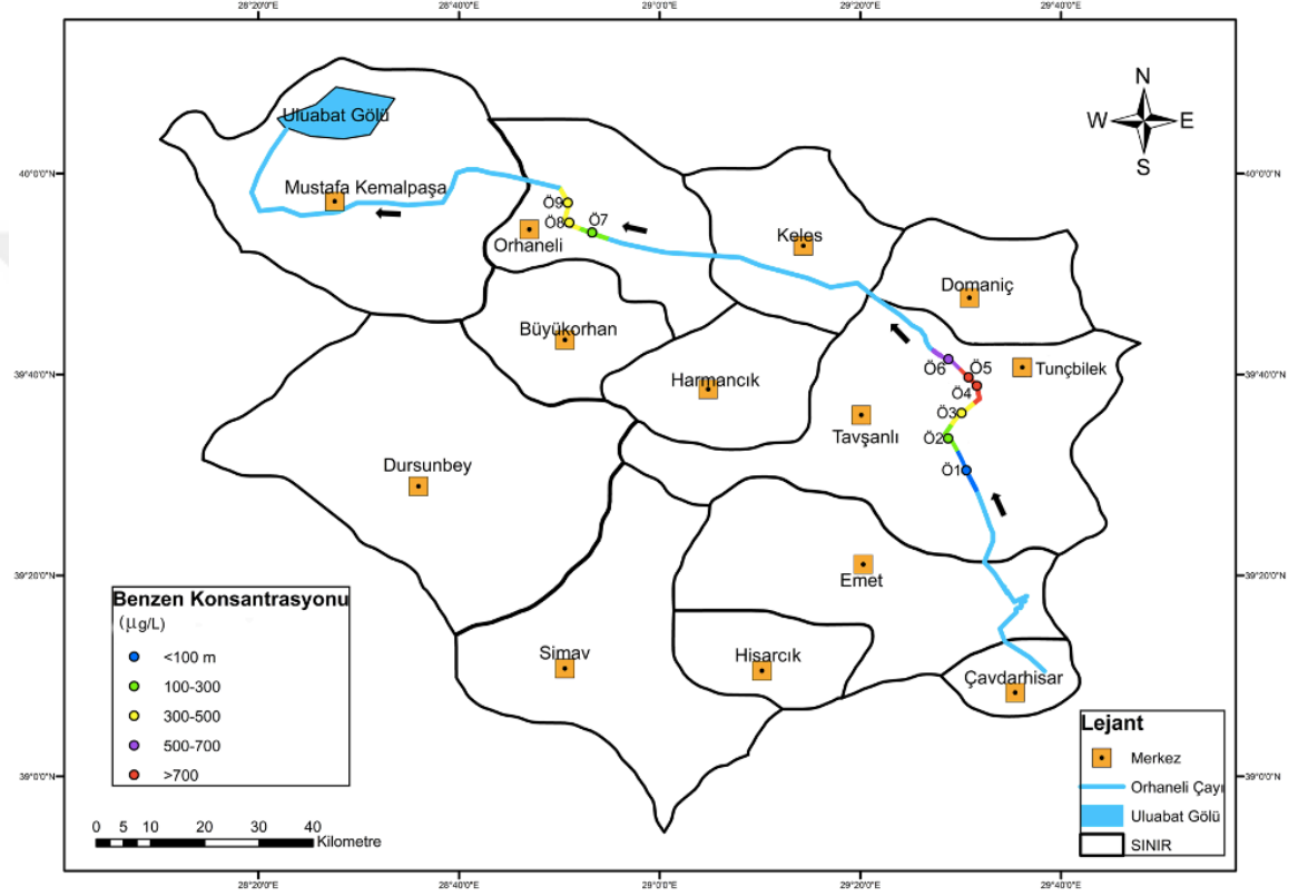
Şekil 4.3. Orhaneli Çayı'ndaki benzen konsantrasyonlarının harita üzerinde gösterimi.
