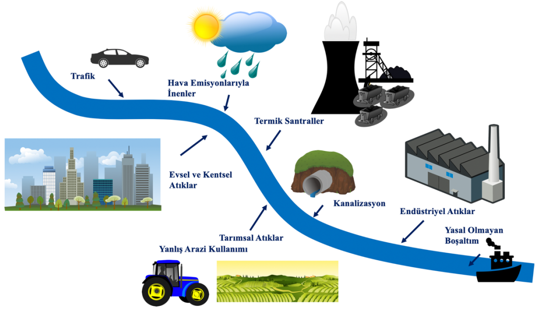
Şekil 1.1. Mikrokirletici kaynakları.
