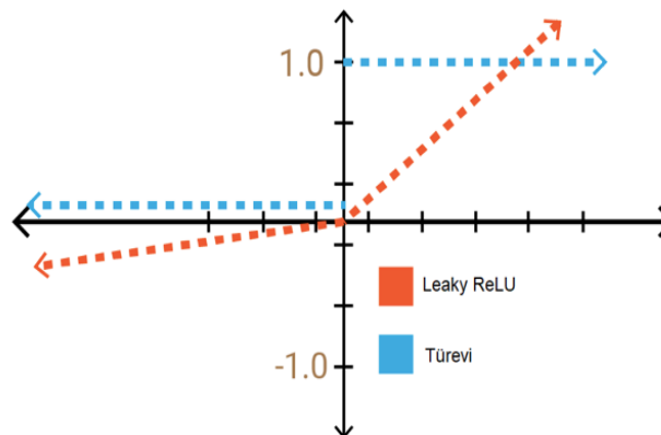
Şekil 2.10. Sızıntı ReLU fonksiyonu ve türevi.
