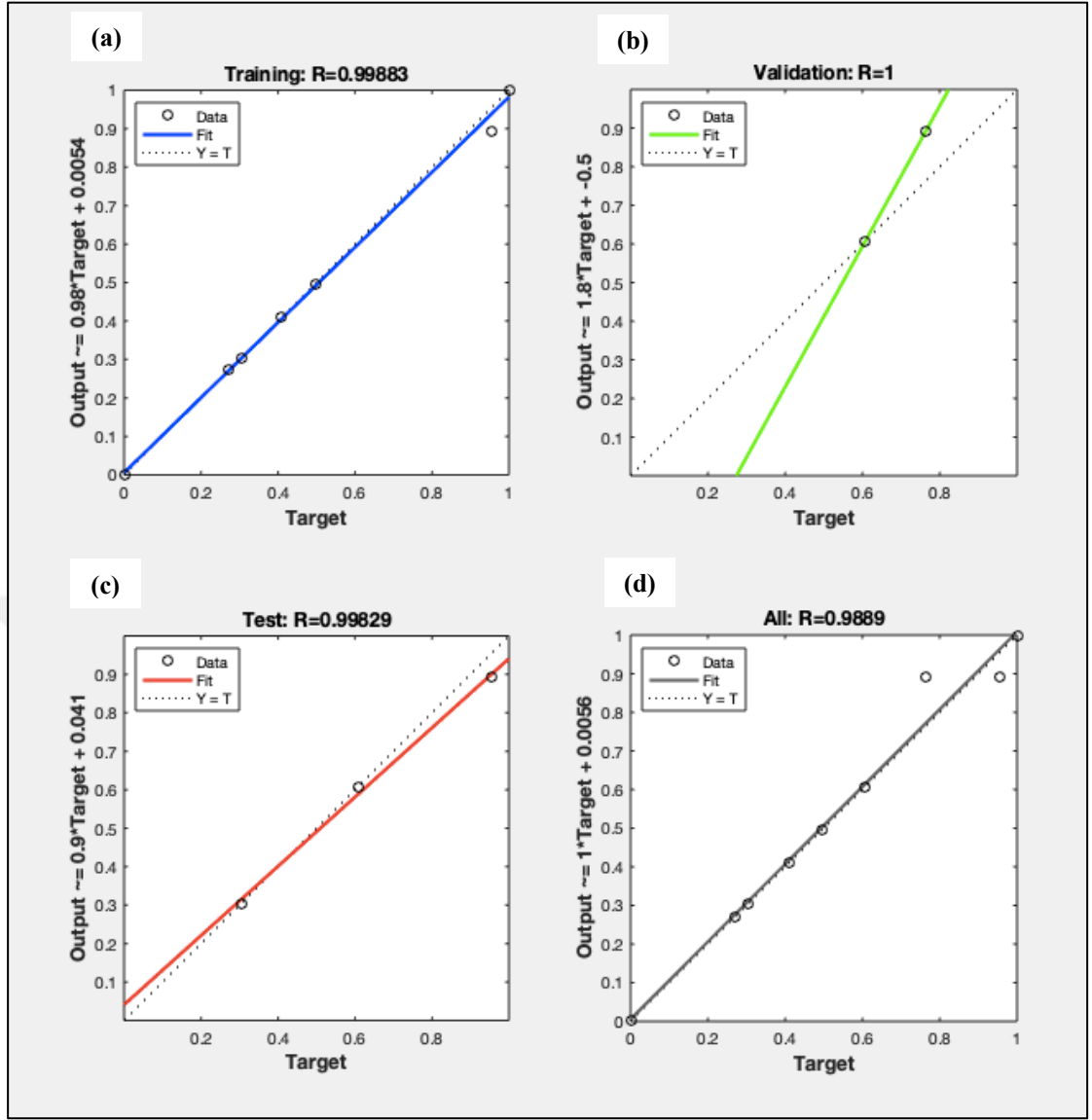
Şekil 4.14. YSA analizi sonucu (a) eğitim, (b) validasyon, (c) test ve (d) genel R korelasyon değerleri.
