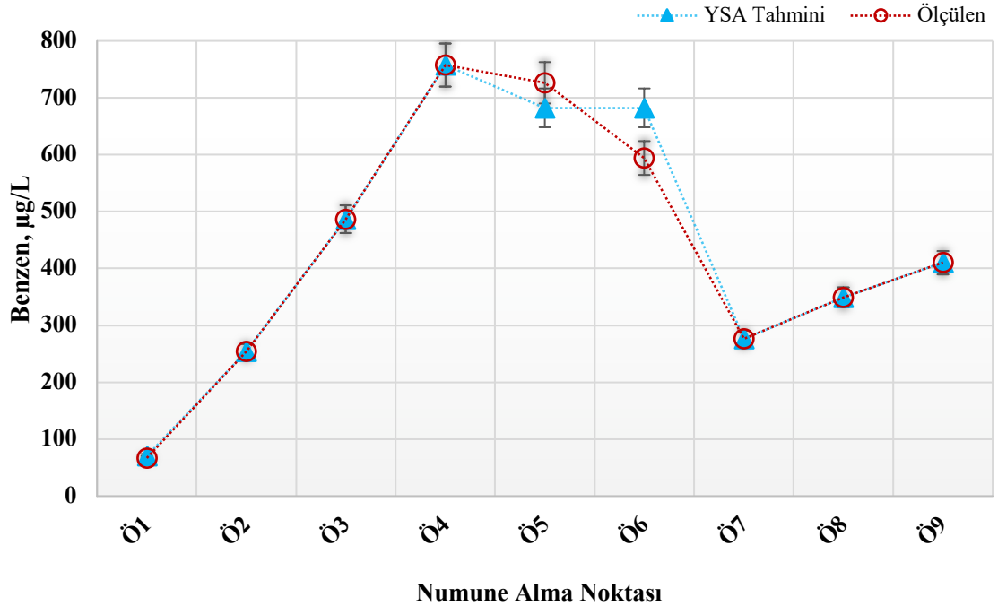
Şekil 4.17. YSA tahmini ve model çıktısı olan benzen konsantrasyonlarının ölçüm noktalarına göre karşılaştırılması.
