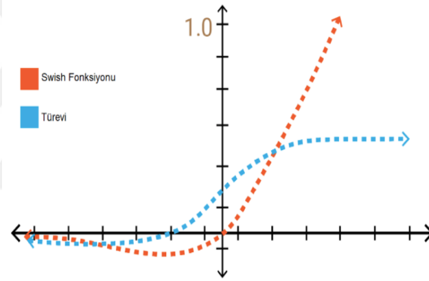
Şekil 2.11. Swish fonksiyonu ve türevi.
