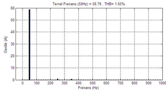
Şekil 6.29. Z kaynağı evriticinin bir fazına ait a) Filtresiz çıkış faz gerilimi b) Filtreli çıkış faz gerilimi c) Çıkış faz akımı ve harmonik spektrumu ( M=1 ve DG=0,45 )
