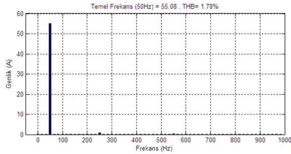
Şekil 6.30. Z kaynak eviricinin bir fazına ait a) Filtresiz çıkış faz gerilimi b) Filtreli çıkış faz gerilimi c) Çıkış faz akımı ve harmonik spektrumu ( M=0,7 ve DG=0,45 )
