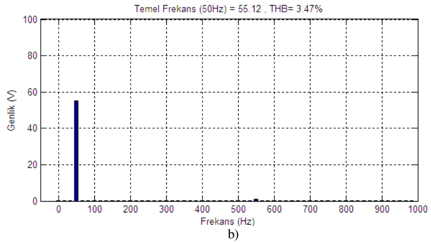
Şekil 6.17. Z kaynak eviricinin bir fazına ait a) Filtreli çıkış faz gerilimi b) Harmonik spektrumu (DG=0,1)
