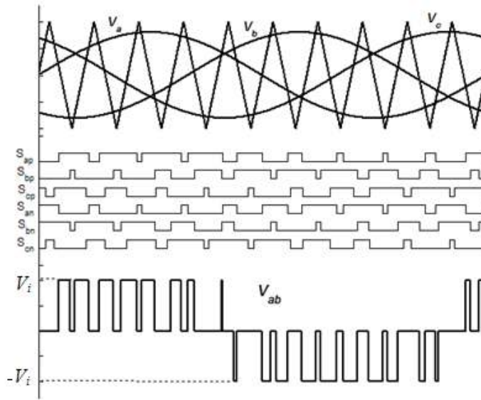
Şekil 4.11. Geleneksel taşıyıcı tabanlı DGM kontrolü
