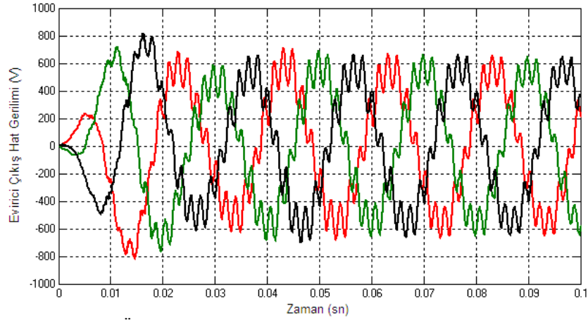
Şekil 6.26. Üç fazlı Z kaynak eviricinin filtreli çıkış hat gerilimi (DG=0,45)
