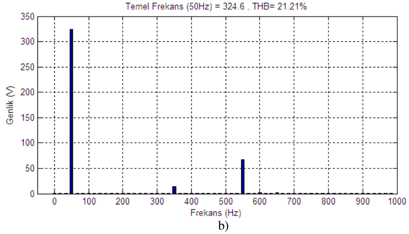
Şekil 6.24. Z kaynak eviricinin bir fazına ait a) Filtreli çıkış faz gerilimi b) Harmonik spektrumu (DG=0,45)
