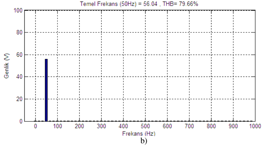
Şekil 6.16. Z kaynak eviricinin bir fazına ait a) Filtresiz çıkış faz gerilimi b) Harmonik spektrumu (DG=0,1)
