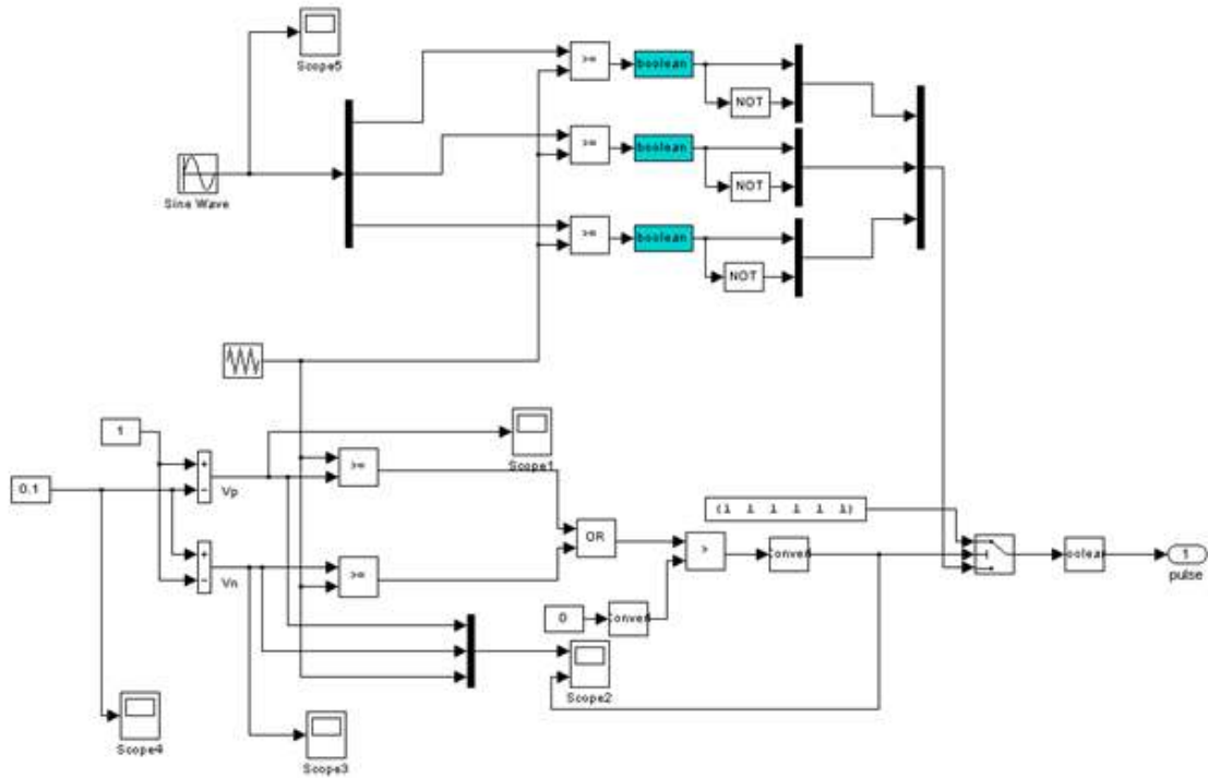
Şekil 6.9. Üç fazlı Z kaynak evirici benzetim modeli
