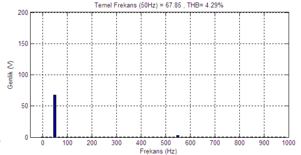
Şekil 6.34. a) Z kaynak eviricinin filtreli çıkış hat gerilimi ve harmonik spektrumu b) Gerilim kaynaklı eviricinin filtreli çıkış hat gerilimi ve harmonik spektrumu ( f_s=10 kHz, DG=0,2 )
