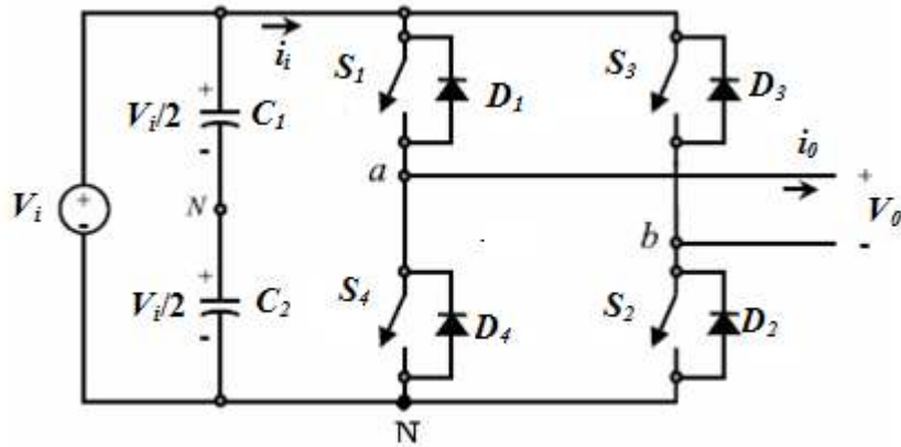
Şekil 2.4. Bir fazlı tam köprü evirici [2].
