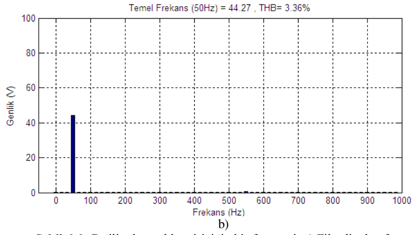
řekil 6.6. Gerilim kaynaklı eviricinin bir fazına ait a) Filtreli ıkıř faz gerilimi b) Harmonik spektrumu
