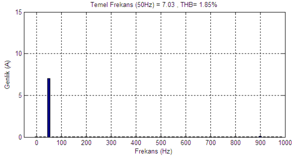
Şekil 6.33. a) Z kaynak eviricinin çıkış faz akımı ve harmonik spektrumu b) Gerilim kaynaklı eviricinin çıkış faz akımı ve harmonik spektrumu ( f_s=1 kHz, DG=0,2 )
