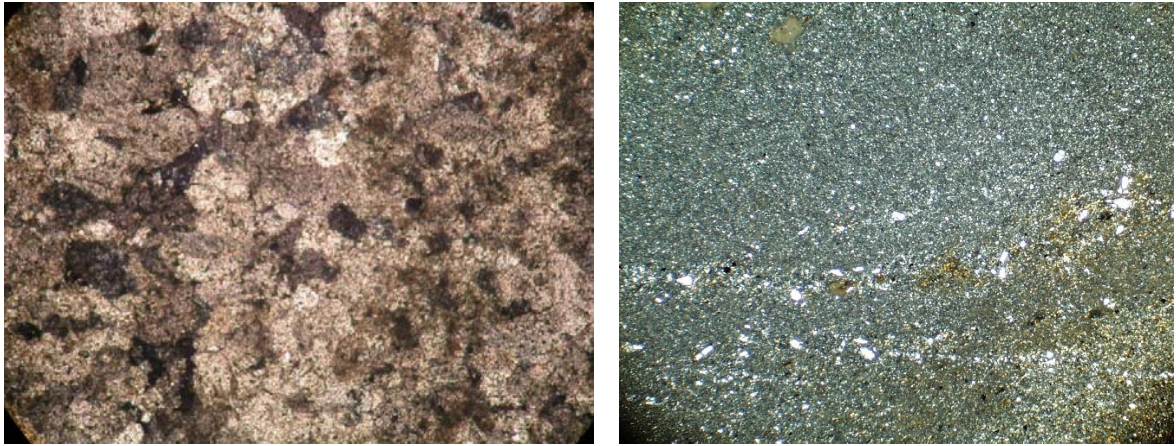
Şekil 3.3. Kireçtaşlarına (a) ve kilitaşlarına (b) ait ince kesit görünümü
