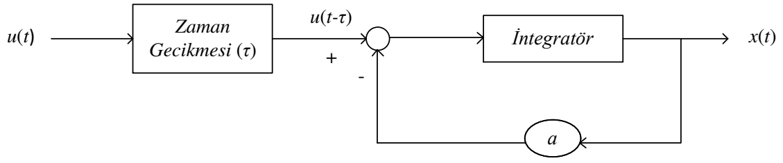
Şekil 4.5. Giriş içinde bir gecikme ile birinci dereceden bir sistem
