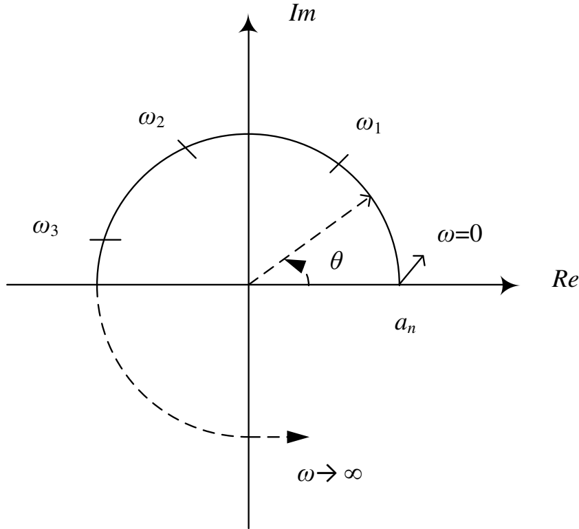
Şekil 6.1. Mikhailov eğrisi
