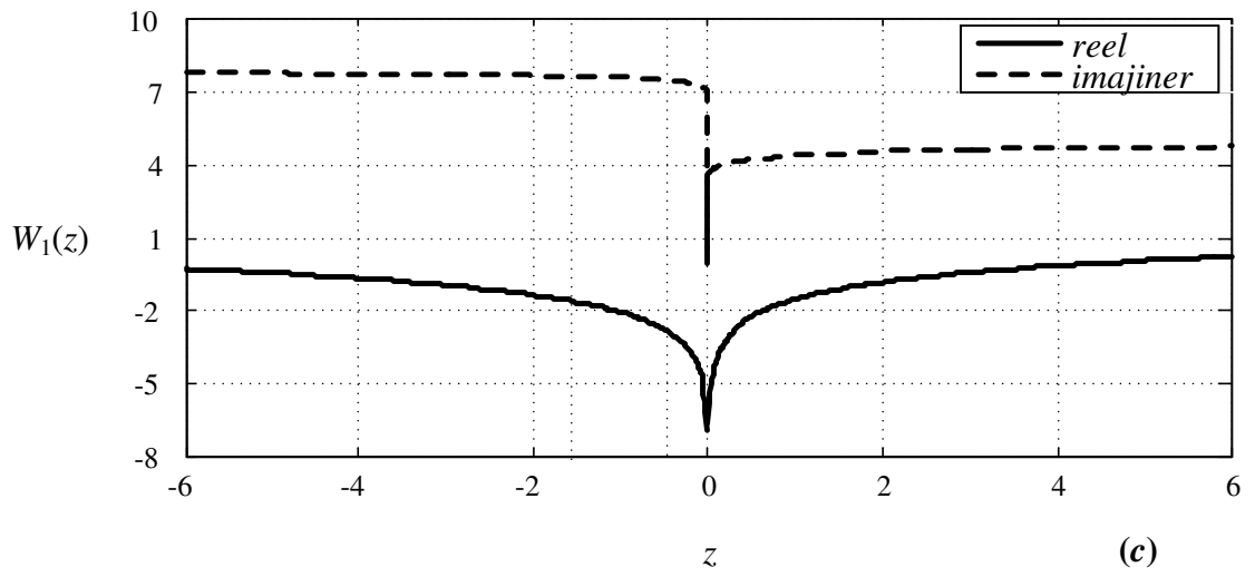
Şekil 5.1. Lambert W fonksiyonunun ; a) -1 , b) 0 ve c) 1 dalına ait reel ve imajiner kısımların çizimi
