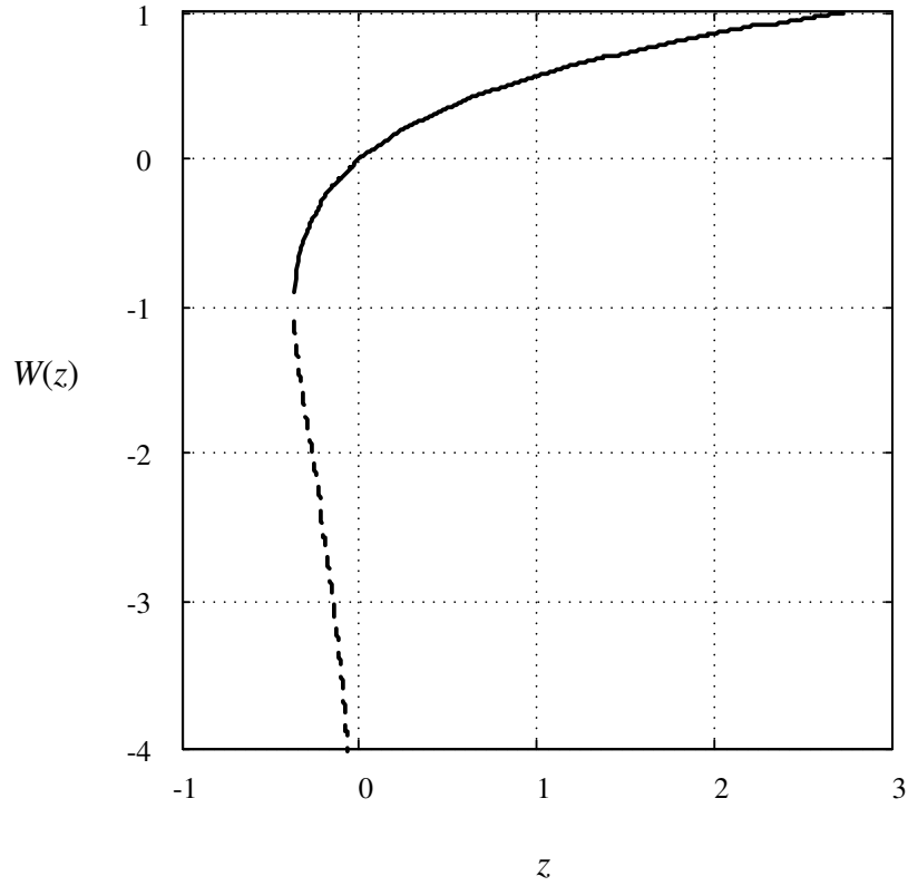
Şekil 5.2. Lambert W fonksiyonunun iki dalının reel değerleri ( W_0 : düz çizgi W_{-1} : kesikli çizgi)
