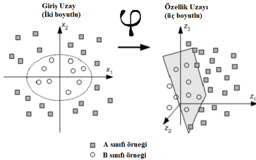
Şekil 2.7. Doğrusal olmayan veri setinin doğrusal olmayan haritalama yaklaşımı
