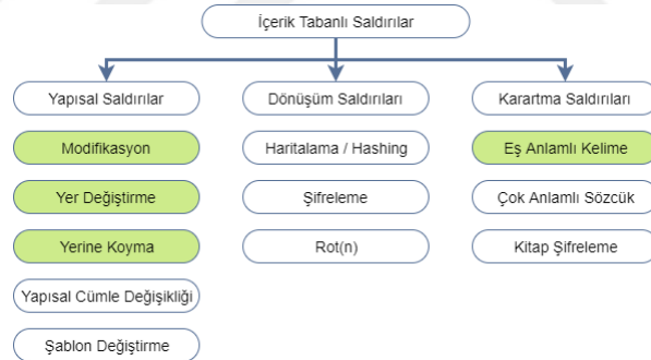
Şekil 2.1. İçerik veri kaçırmada saldırı türleri
