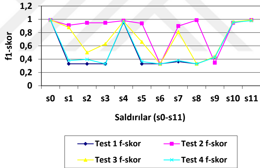
Şekil 4.4. Dynacorp test grafiği
