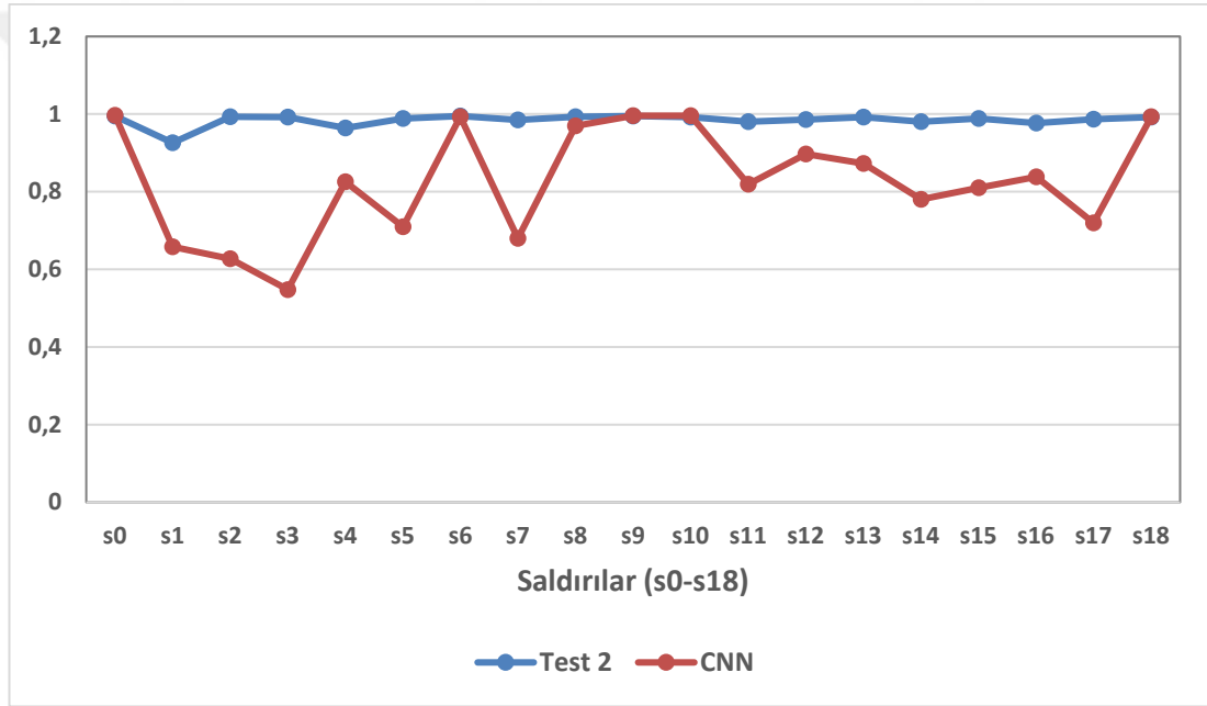
Şekil 4.6. Test 2 modeli ile CNN accuracy değerleri karşılaştırma grafiği
