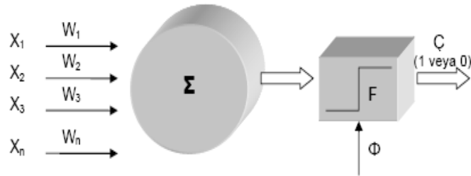
Şekil 2.11. Basit Algılayıcı ağ modeli
