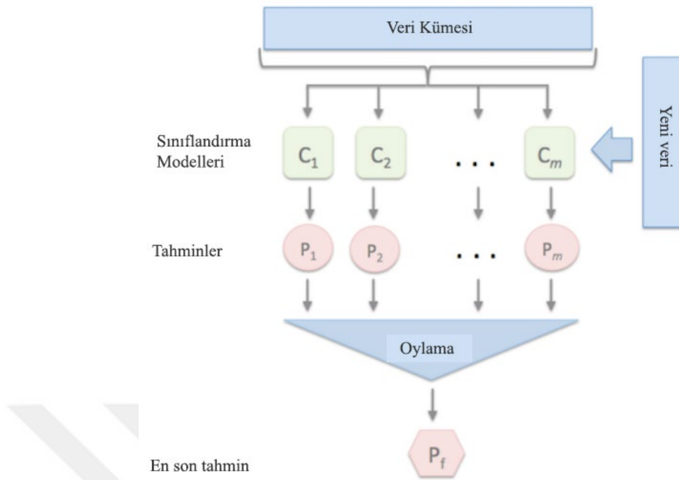
Şekil 2.8. Oylamalı sınıflandırıcı genel çalışma şekli
