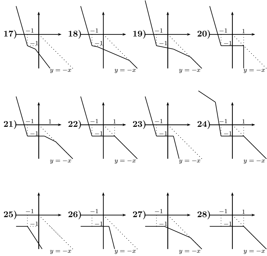
Şekil 3.11: \inf_{x_0 \geq -1} [(ax_0, bx_0) + (d|x_0|, d|x_0|)] - f^w(x_0, a, b, d) kümeleri
