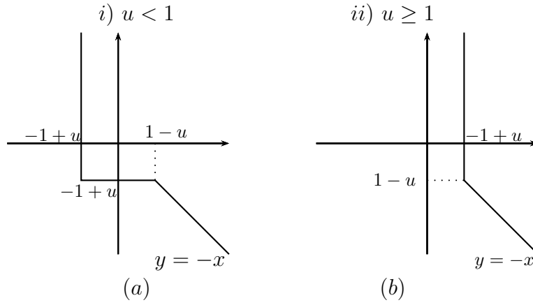
Şekil 3.9: (a) u < 1 iken değer dönüşümünün görüntü kümesi (b) u \geq 1 iken değer dönüşümünün görüntü kümesi
