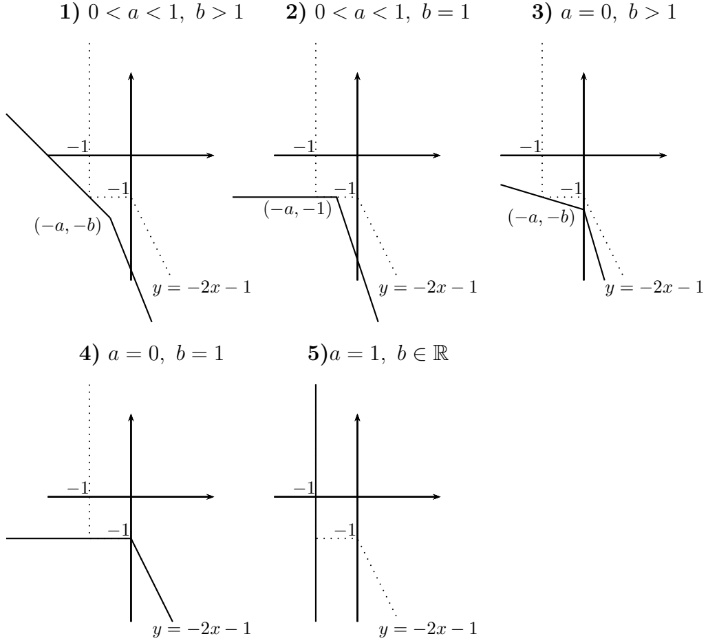
Şekil 3.7: \inf_{x \in \mathbb{R}} (x - ax - a, -|x| - bx - b) kümeleri
