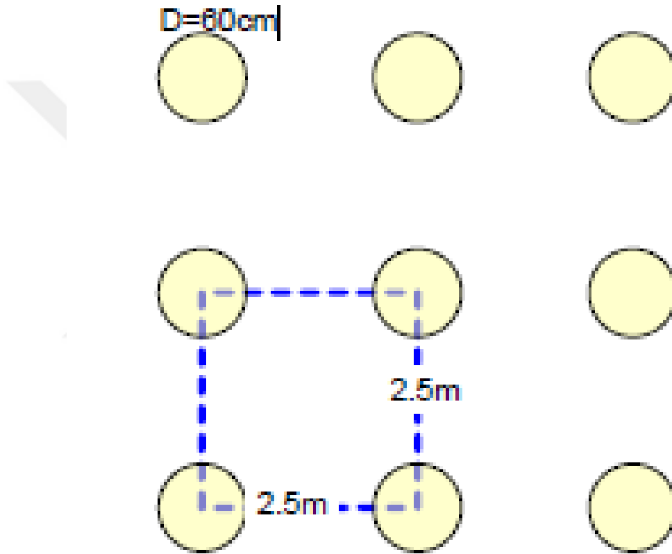
Şekil10.7. İnceleme alanına uygulanan Jetgrout dizilim planı.
