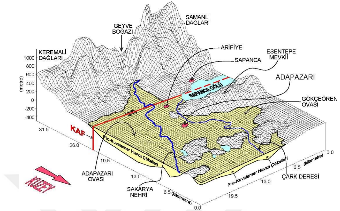
Şekil 2.3. Adapazarı'nın KD'den GB'ya doğru morfolojik görünümü [9].
