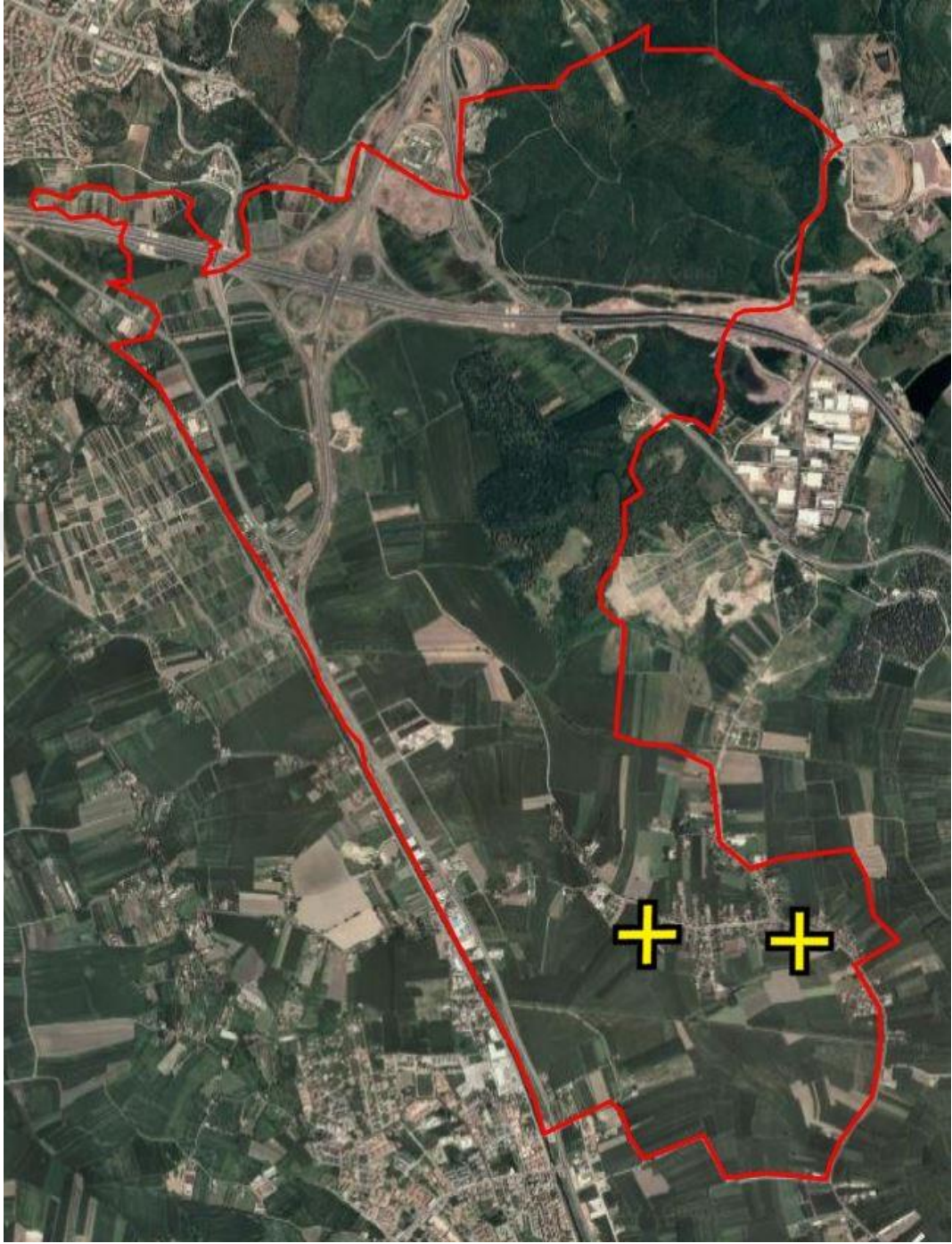
Şekil 11.3. Karakamış Mahallesi'nde yapılan Sismik ve Sondaj çalışmaları yerleri.
