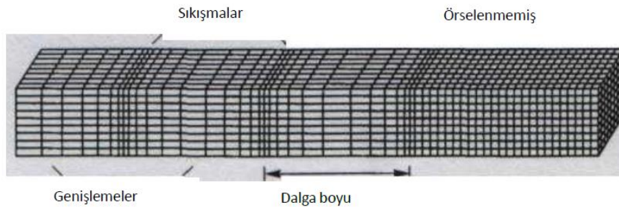
Şekil 3.1. P Dalgası yayılımı [14].
