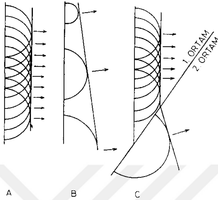
Şekil 3.6. Huygens prensibine göre düzlem dalga yayınımları; A) Homojen ortam B) Hızın düşey yönde doğrusal (lineer) artması C) Ortam değişikliği nedeniyle hızın ani olarak değişimi [15]
