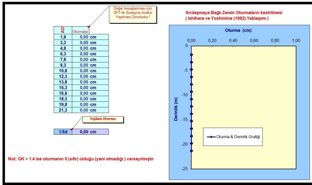
Şekil 5.29. Deprem büyüklüğü 7.5 ve ivme değeri 0.05 için Sıvılaşmaya zemin oturmalarının kestirilmesi analizi
