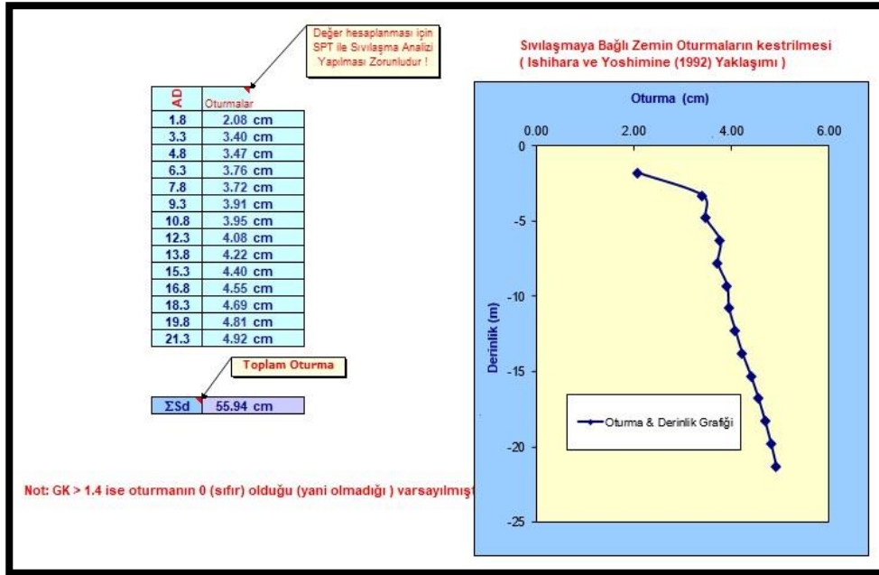
Şekil 5.41. Deprem büyüklüğü 7.5 ve ivme değeri 0.30 için sıvılaşmaya bağlı zemin oturmalarının kestirilmesi
