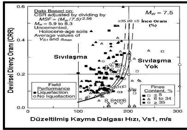
Şekil 4.7. Devirsel direnç oranı (CRR) ve düzeltilmiş V_s hızı arasındaki ilişki (Seed ve Idriss, 1983).
