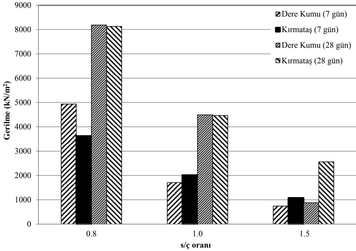
Şekil 5.6. Farklı s/ç oranlarına göre %60 relatif sıkılığa hazırlanmış dere kumu ve kırmataş kullanılarak elde edilen enjeksiyon numunelerinin 7 ve 28 günlük serbest basınç dayanımları
