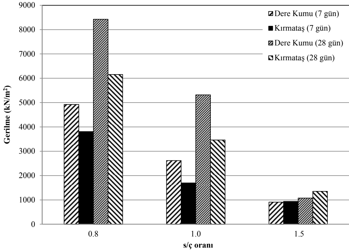
Şekil 5.7. Farklı s/ç oranlarına göre %80 relatif sıkılıkta hazırlanmış dere kumu ve kırmataş kullanılarak elde edilen enjeksiyon numunelerinin 7 ve 28 günlük serbest basınç dayanımları
