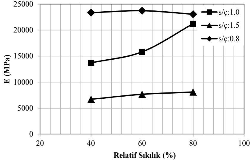
Şekil 5.12. Dere kumu kullanılarak elde edilmiş enjeksiyon numunelerinin artan relatif sıkılık ve değişen s/ç oranlarına göre E değişimleri (7 Günlük)
