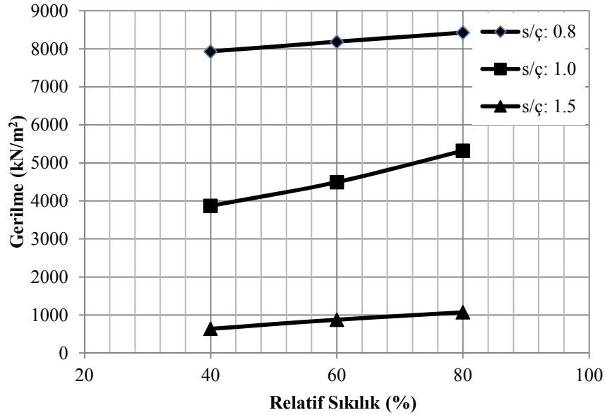
Şekil 5.2. Dere kumu kullanılarak elde edilmiş enjeksiyon numunelerinin artan relatif sıkılık ve değişen s/ç oranlarına göre serbest basınç dayanım değişimleri (28 Günlük)
