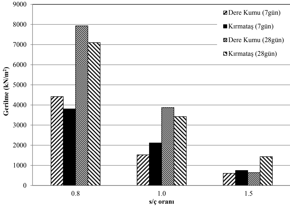
Şekil 5.5. Farklı s/ç oranlarına göre %40 relatif sıkılıkta hazırlanmış dere kumu ve kırmataş kullanılarak elde edilen enjeksiyon numunelerinin 7 ve 28 günlük serbest basınç dayanımları
