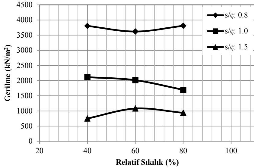
Şekil 5.3. Kırmataş kullanılarak elde edilmiş enjeksiyon numunelerinin artan relatif sıklık ve değişen s/ç oranlarına göre serbest basınç dayanım değişimleri (7 Günlük)
