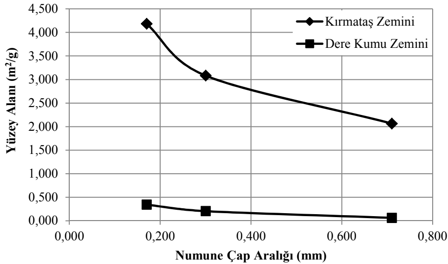
Şekil 6.2. Dere kumu ve kırmataş zemin türlerinin numune çap aralıklarına göre yüzey alanları değişimi
