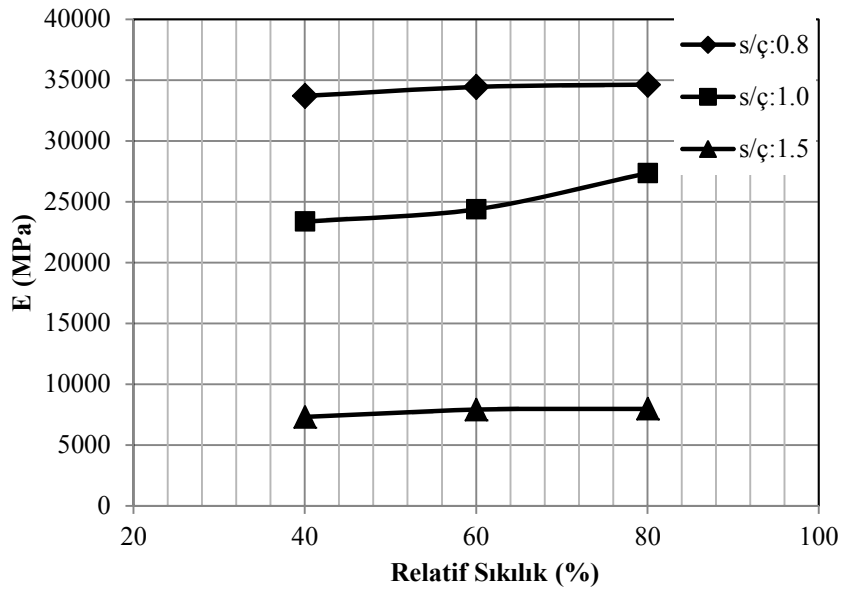
Şekil 5.13. Dere kumu kullanılarak elde edilmiş enjeksiyon numunelerinin artan relatif sıkılık ve değişen s/ç oranlarına göre E değişimleri (28 Günlük)
