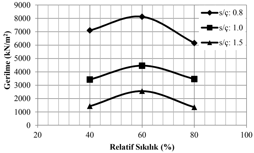
Şekil 5.4. Kırmataş kullanılarak elde edilmiş enjeksiyon numunelerinin artan relatif sıklık ve değişen s/ç oranlarına göre serbest basınç dayanım değişimleri (28 Günlük)
