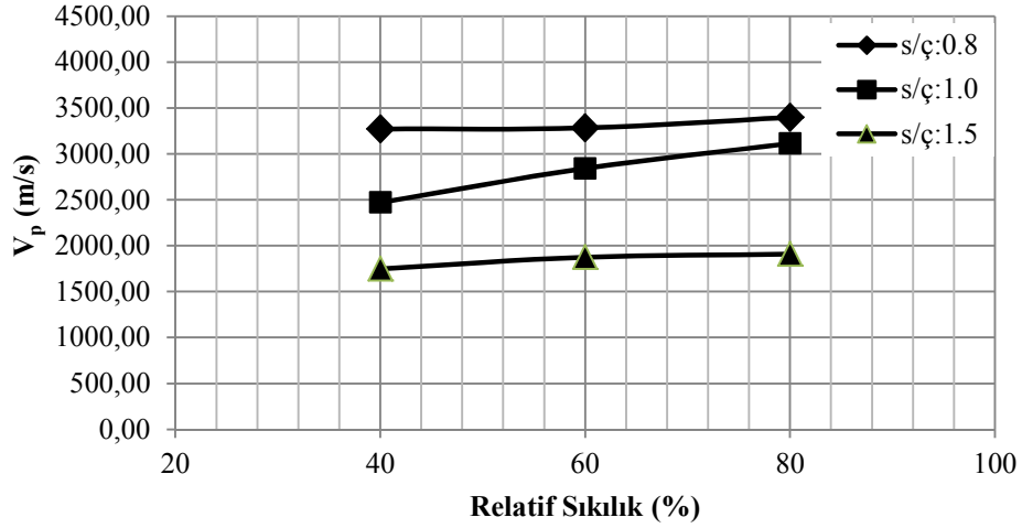
Şekil 5.8. Dere kumu kullanılarak elde edilmiş enjeksiyon numunelerinin artan relatif sıkılık ve değişen s/ç oranlarına göre V_p değişimleri (7 Günlük)
