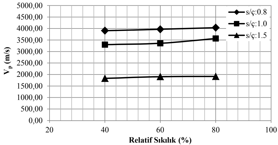
Şekil 5.9. Dere kumu kullanılarak elde edilmiş enjeksiyon numunelerinin artan relatif sıkılık ve değişen s/ç oranlarına göre V_p değişimleri (28 Günlük)
