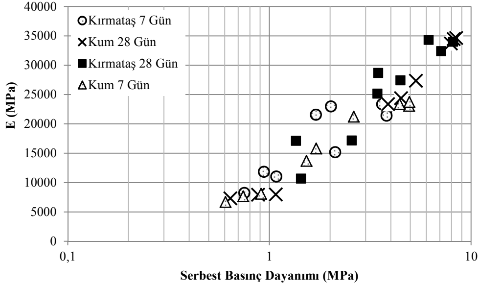
Şekil 6.3. Enjeksiyon numunelerinin serbest basınç dayanımı ile E arasındaki ilişki
