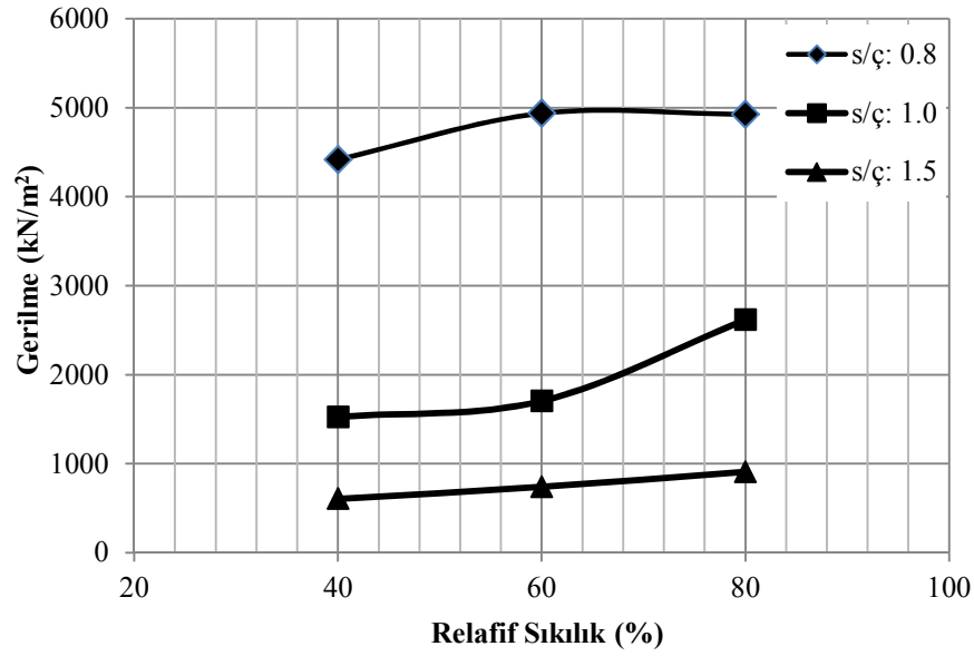
Şekil 5.1. Dere kumu kullanılarak elde edilmiş enjeksiyon numunelerinin artan relatif sıkılık ve değişen s/ç oranlarına göre serbest basınç dayanım değişimleri (7 Günlük)
