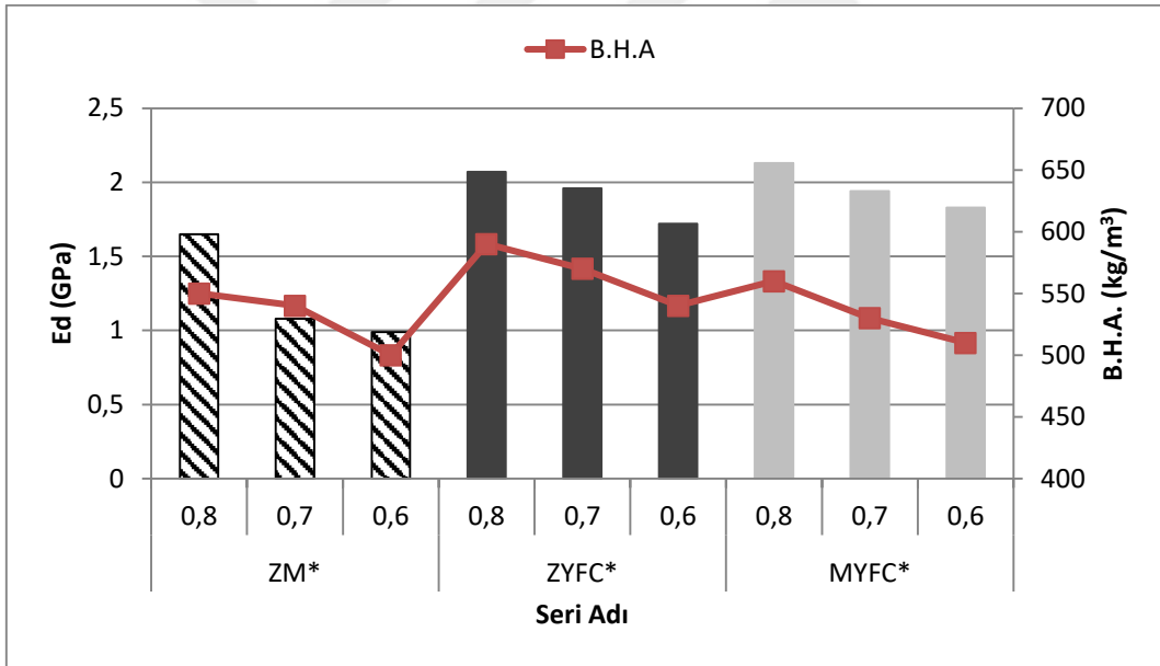
Şekil 4.16 Hammddelerin karıştırılması ve akışkanlaştırıcı ile üretilen serilerin dinamik elastisite modülü bulguları.
