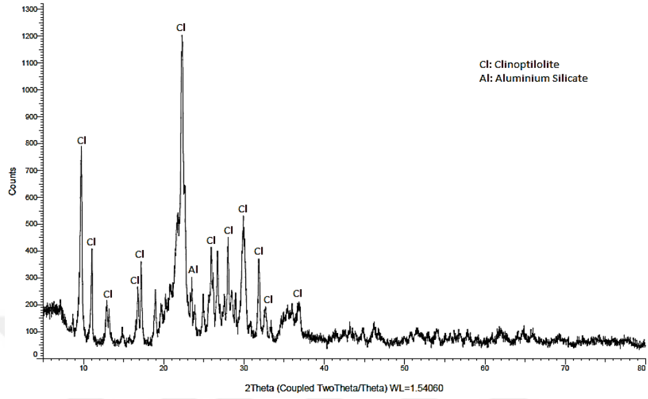
Şekil 3.2 Zeolite ait XRD analizi.
