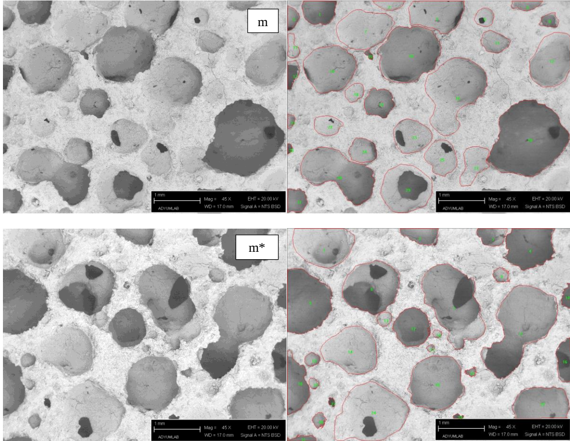
Resim 4.2 Metakaolin ile üretilen örneklere ait makroyapı resmi.
