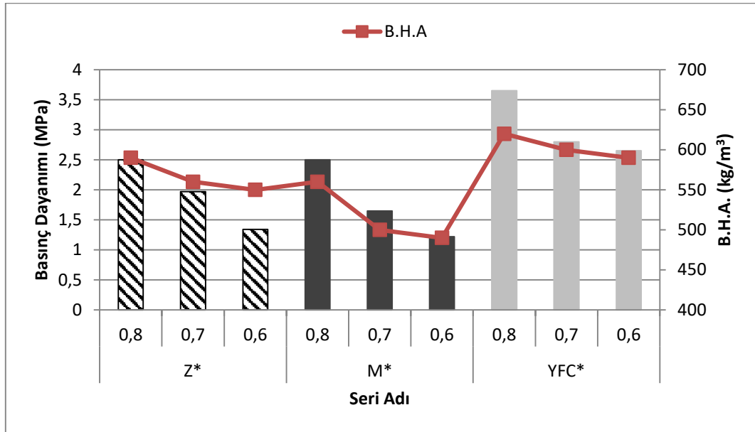
Şekil 4.11 Zeolit, metakaolin, YFC ve akışkanlaştırıcı ile üretilen serilerin basınç dayanımı bulguları.
