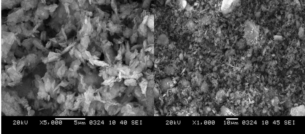
Şekil 2.5 Metakolin mineralinin SEM görüntüleri (Çelikten 2014).
