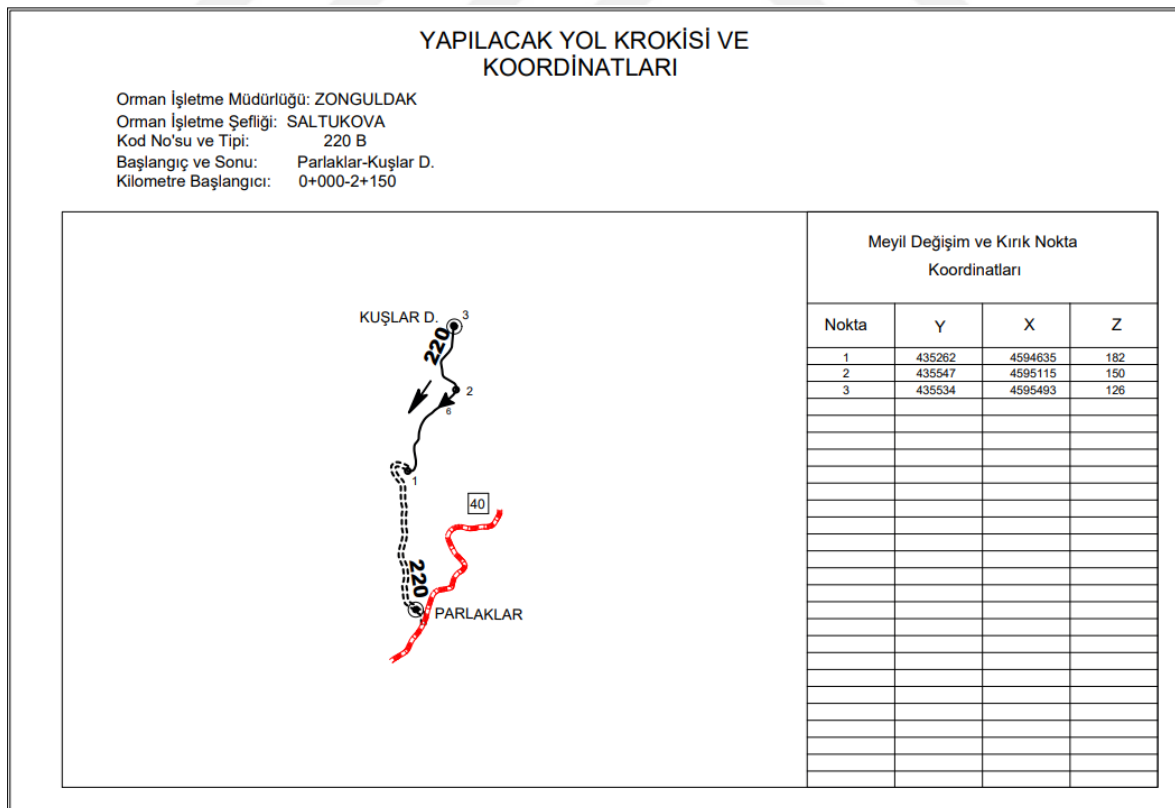
Şekil 4.20: 220 B kodlu Parlaklar - Kuşlar Deresi yol hattı krokisi ve koordinatları
