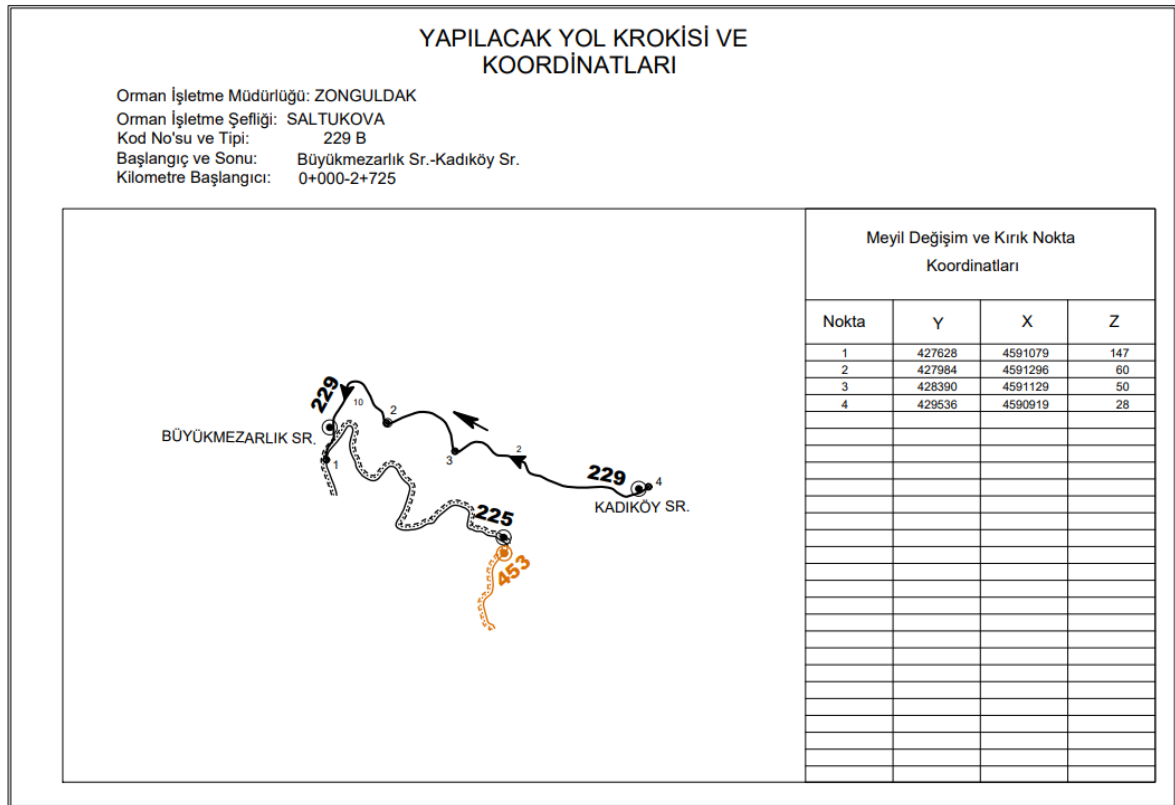
Şekil 4.26: 229 B kodlu Büyük mezarlık – Kadıköy yol hattı krokisi ve koordinat
