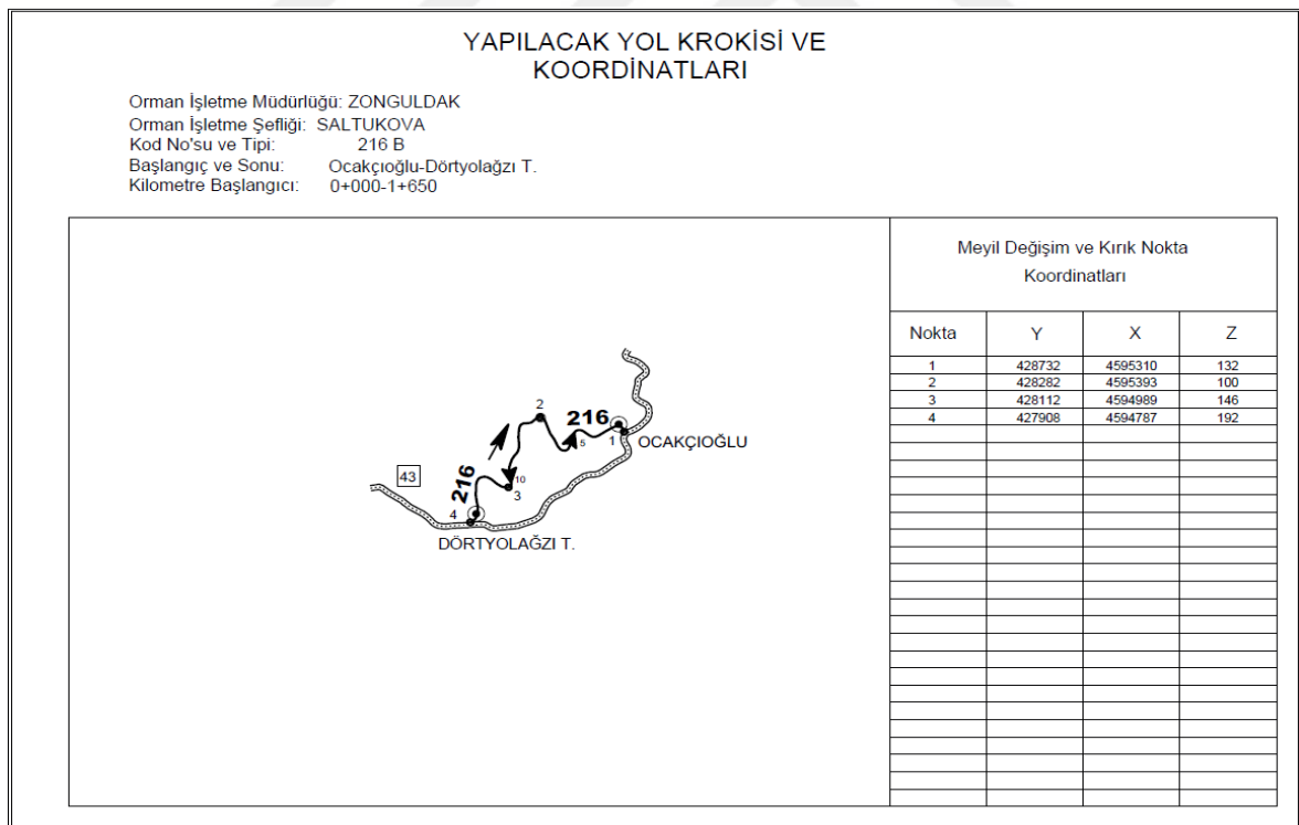
Şekil 4.16: 216 B kodlu Ocakcıoğlu – Dörtyolağzı Tepesi yol hattı krokisi ve koordinatları
