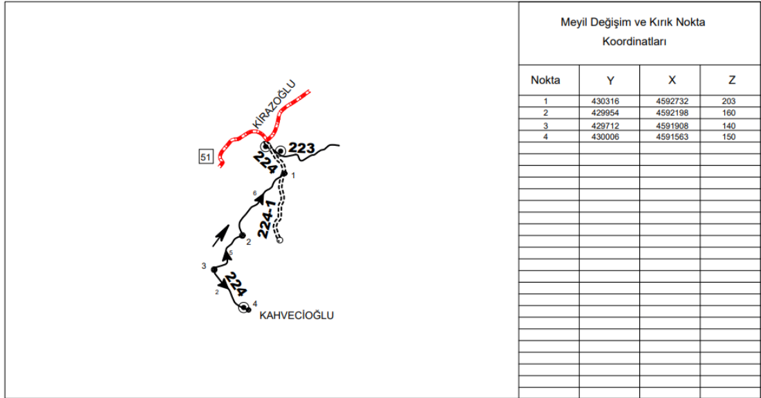
Şekil 4.23: 224 B kodlu Kirazoğlu – Kahvecioğlu yol hattı krokisi ve koordinatları
