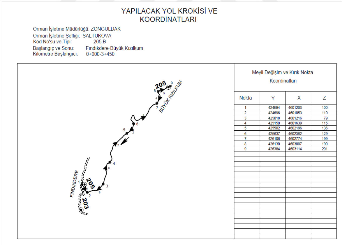
Şekil 4.7: 205 B kodlu Fındıklıdere – Büyük Kızılkum hattı krokisi ve koordinatları
