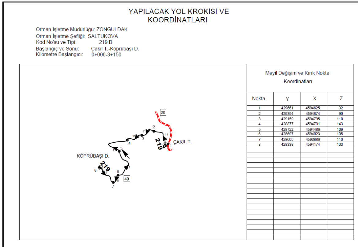
Şekil 4.19: 219 B kodlu Çakıltepe - Köprübaşı Deresi yol hattı krokisi ve koordinatları
