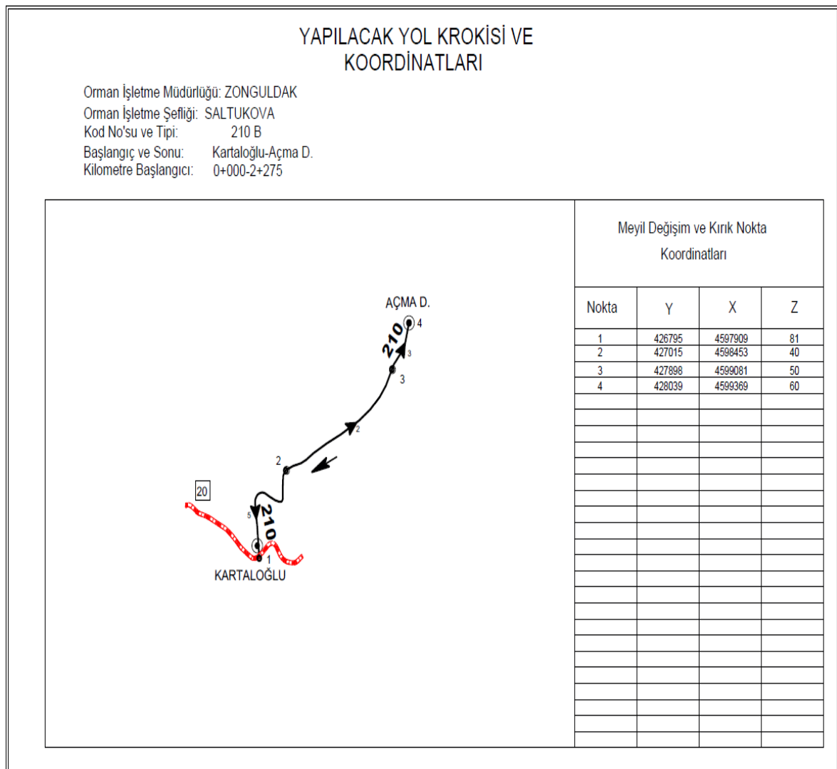
Şekil 4.11: 210 B kodlu Kartaloğlu – Açma Deresi yol hattı krokisi ve koordinatları
