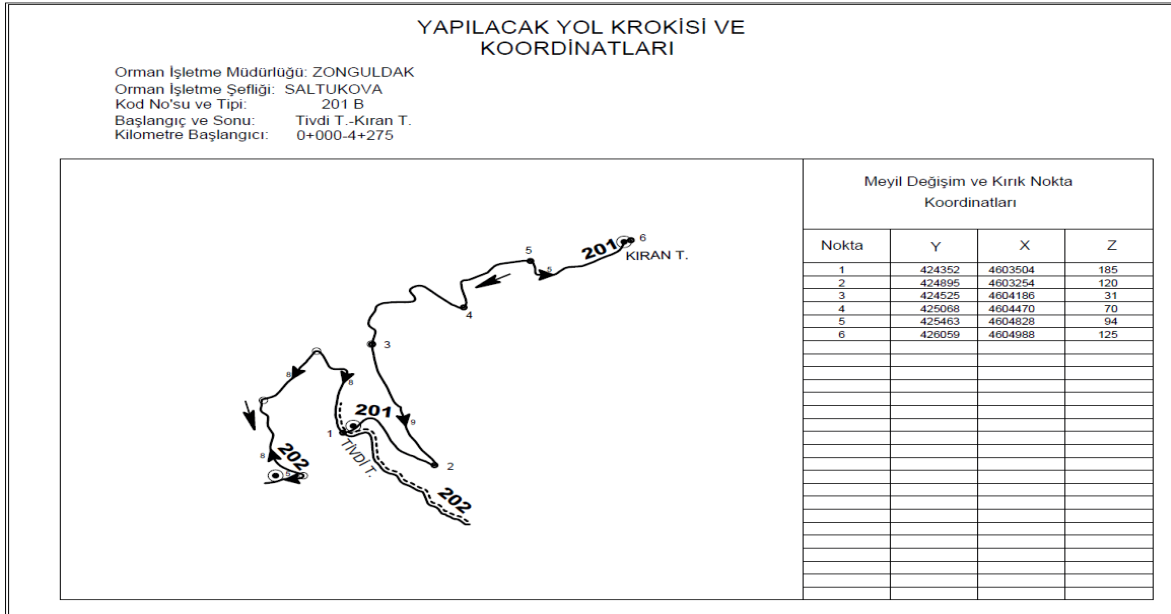
Şekil 4.4: 201 B kodlu Tevdi Tepe Kıran Tepe hattı krokisi ve koordinatları
