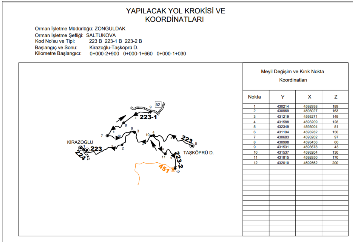
Şekil 4.22: 223 B kodlu Kirazoğlu – Taşköprü Deresi yol hattı krokisi ve koordinatları
