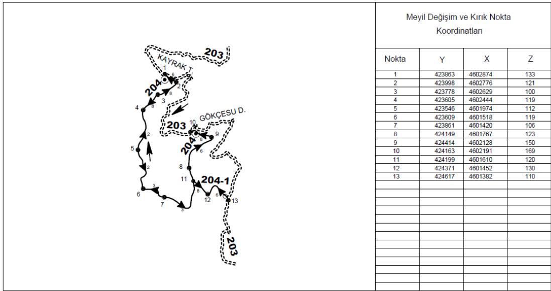
Şekil 4.6: 204 B kodlu Kayrak Tepe-Gökçesu Deresi hattı krokisi ve koordinatları
